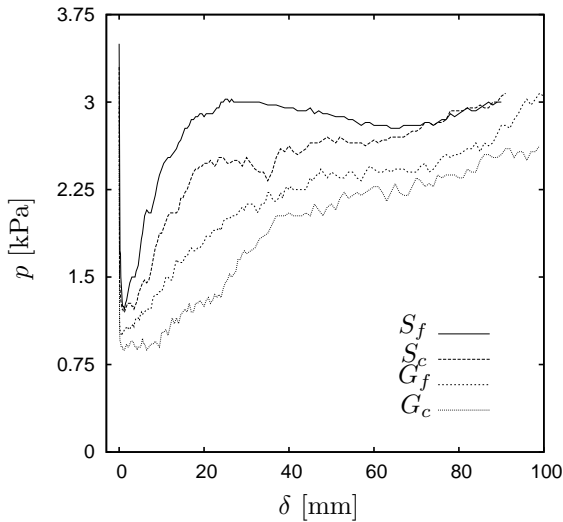
FIGURE 2.48 – Évolution de p en fonction de \delta pour G_c , G_f , S_c et S_f pour h = 0.20 m.
