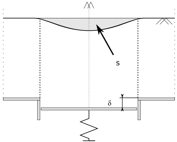
FIGURE 3.15 – Définition de la surface s utilisée pour quantifier le tassement de surface des couches granulaires.
