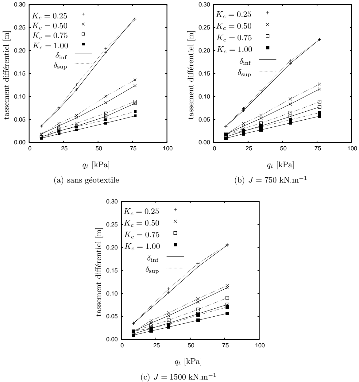
FIGURE 4.27 – Tassements différentiels en base et en surface du matelas en fonction de q_t pour différents modules de réaction K_c ( \text{MPa.m}^{-1} ); h_m = 0.5 m, avec géotextile de renforcement, sans dallage.
