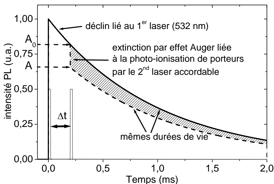
Figure IV-26 : illustration schématique de la chute d'amplitude des déclin enregistrés lors de l'utilisation combinée de deux lasers impulsions.
