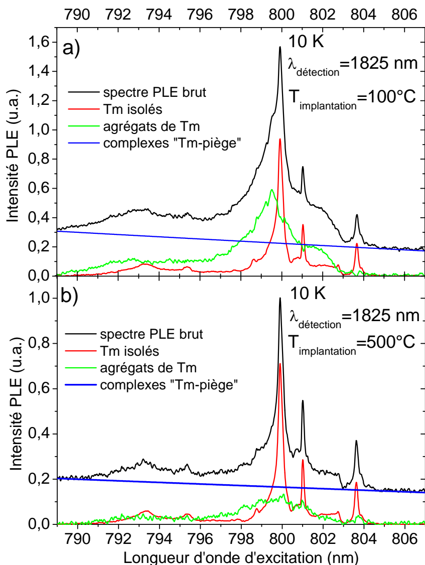
Figure II-23 : Séparation des différentes contributions aux spectres de PLE détectés à 1.8 \mu\text{m} pour les échantillons recuits à 100 et 500^\circ\text{C} .
