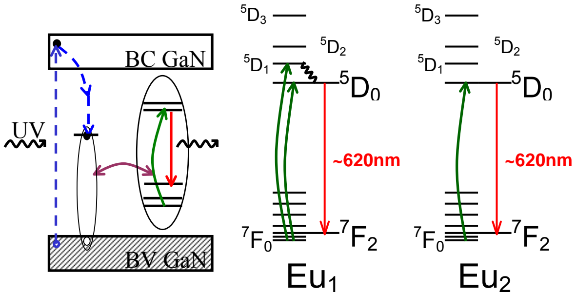
Figure III-23 : Représentation schématique des chemins d'excitation du multiplet ^5D_0 des ions Eu_1 et Eu_2 suite à une excitation bande à bande.
