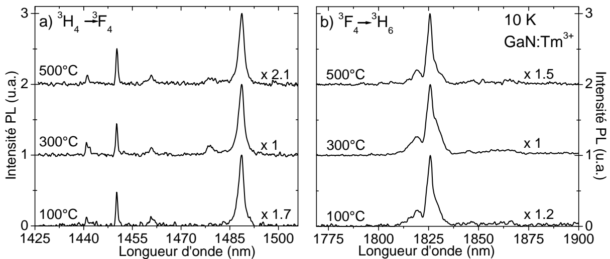
Figure II-20 : Spectres de PL à 1.5 et 1.8 \mu m suite à une excitation résonante à 800 nm dans GaN : Tm^{3+} .
