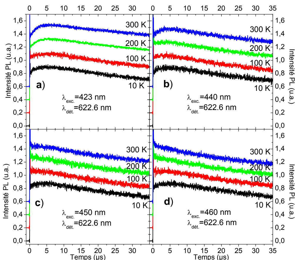
Figure III-26 : Evolution des dynamiques de PL aux temps courts du multiplet ^5D_0 pour le site \text{Eu}_1 en fonction de la température pour quatre longueurs d'onde d'excitation différentes : a) 423 nm, b) 440 nm, c) 450 nm et d) 460 nm.
