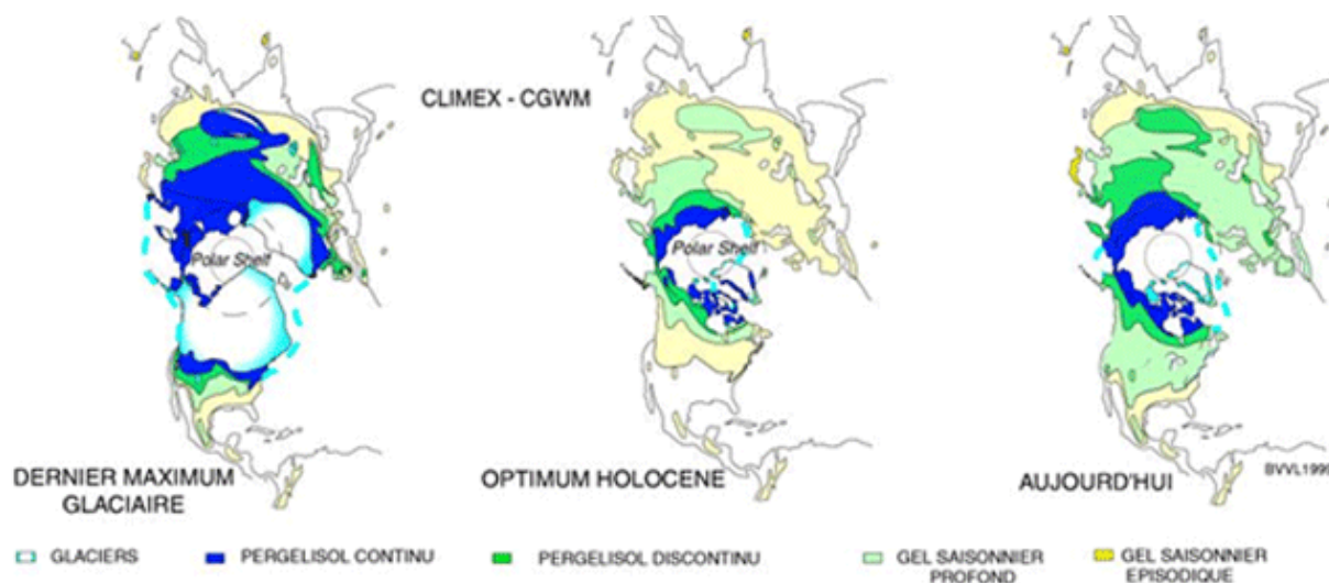
Figure II- 9 : Cartes de l'extension du pergélisol il y a 20 000 ans (maximum glaciaire), 7 000 ans (lors du plus chaud de notre interglaciaire) et à l'actuel.
