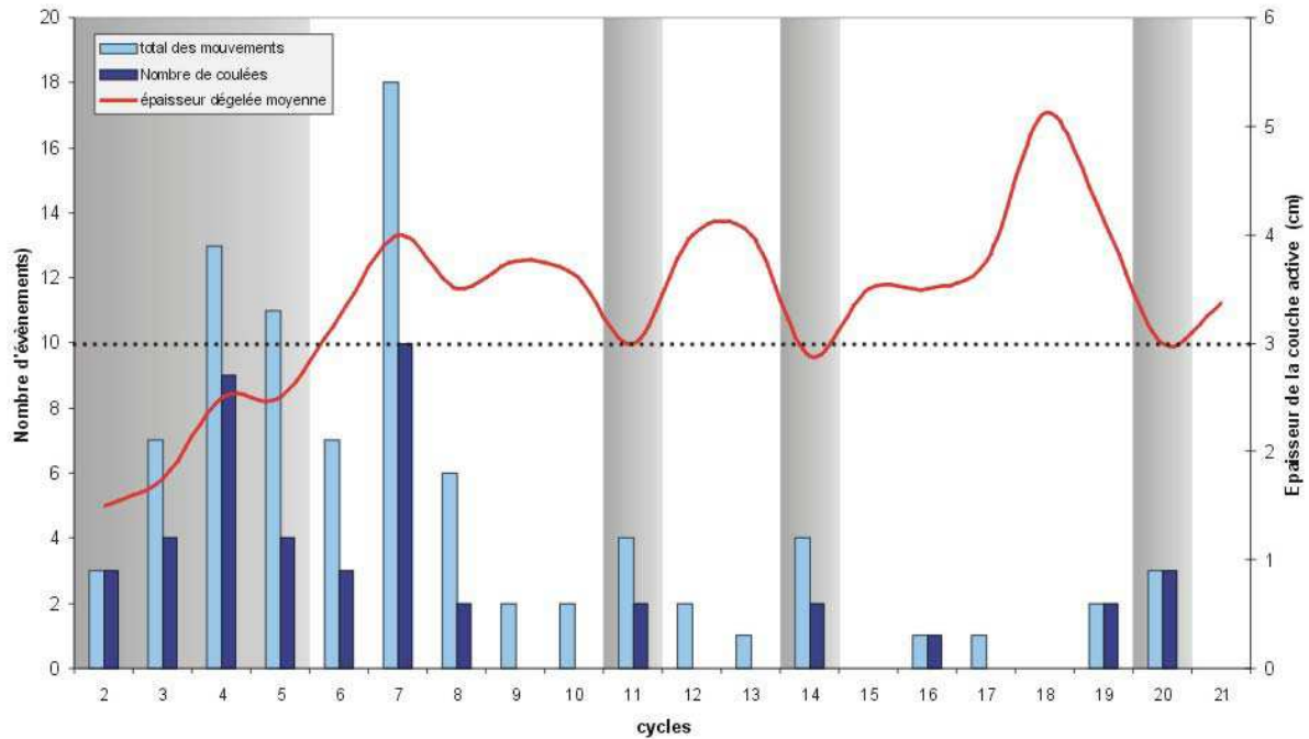
Figure V - 20 : Relation entre l'épaisseur de la couche active et le nombre d'événements « catastrophiques ».
