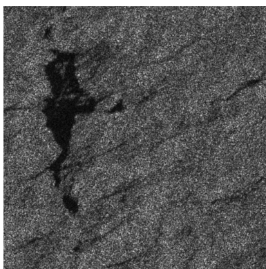
Figure 2.13 – Extrait ( 512 \times 512 ) d'une image ERS-RSO d'une nappe de pétrole au large des côtes Égyptiennes, ©ESA.
