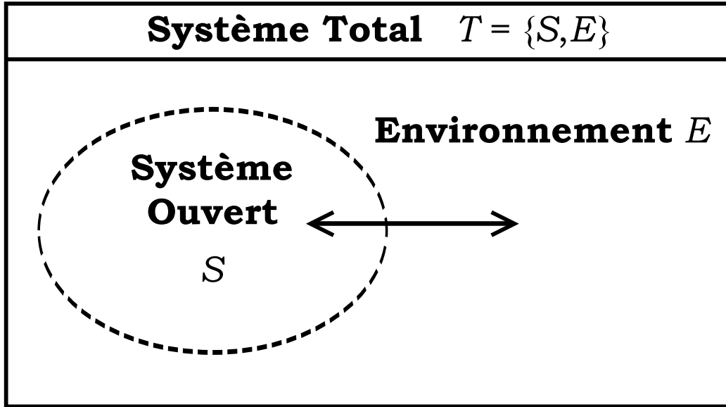
FIG. 1.1 – Représentation schématique d'un système ouvert.
