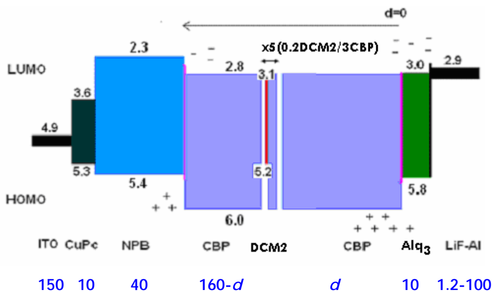
Figure III.21 : Structure utilisée pour l'étude des recombinaisons directes. (Les épaisseurs sont indiquées en nanomètres)
