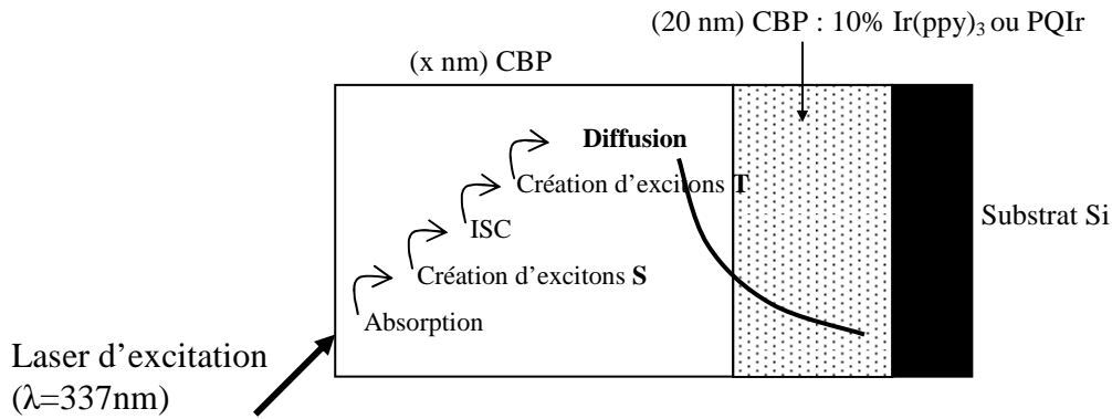
Figure III.7 : Principe de mesure de la longueur de diffusion des triplets du CBP par la méthode de temps de vol.
