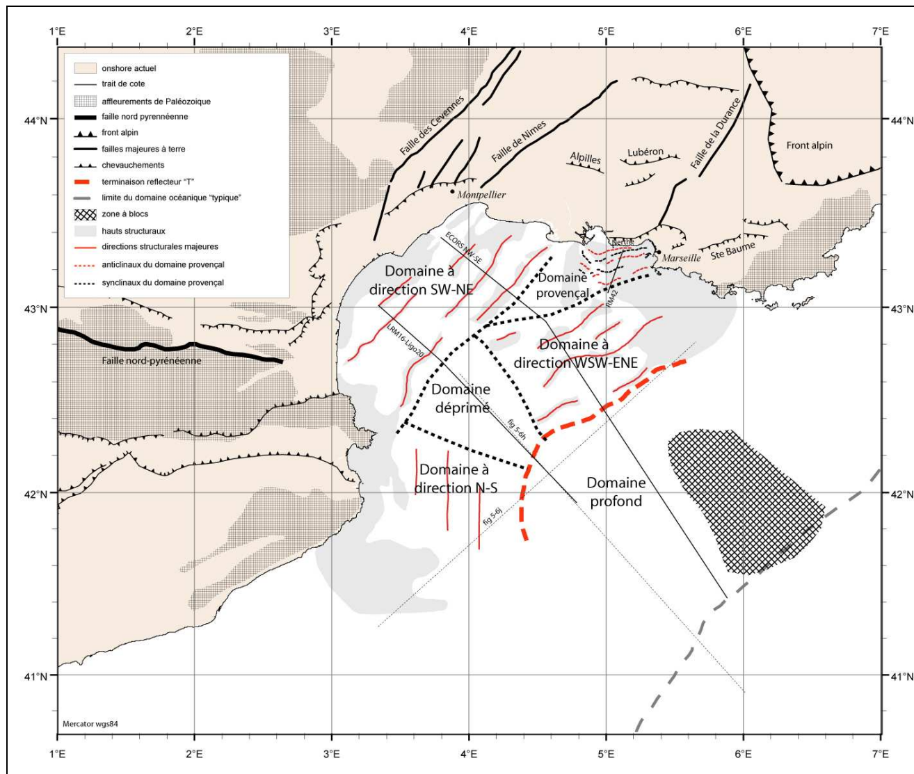
Figure V-2 : les grands domaines structuraux du golfe du Lion. Commentaires dans le texte.
