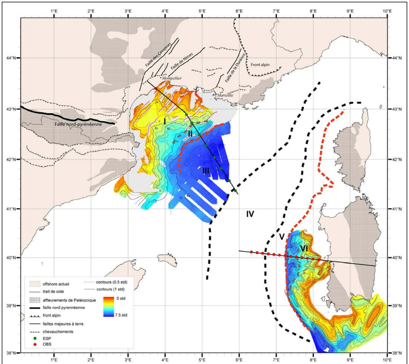
Figure II-17: Carte de la profondeur du substratum (en secondes temps double) dans le golfe du Lion (cette étude) et sur la marge Sarde (Thomas, 1986). Les zones I à VI sont décrites dans le texte.
