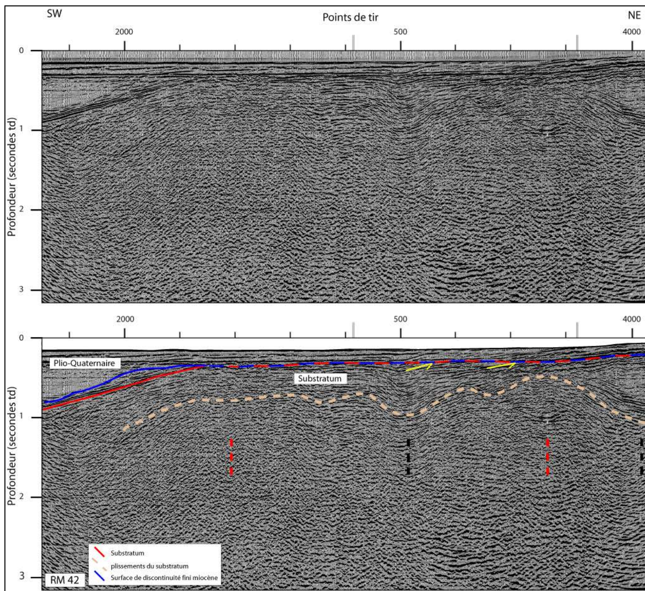
Figure V-4: Morphologie du substratum dans le domaine provençal. On peut observer une allure plissée d'une part et l'aplanissement du toit du substratum par une érosion fini-miocène ou plus ancienne d'autre part. Position sur la Figure V-2 et sur la Figure V-13.
