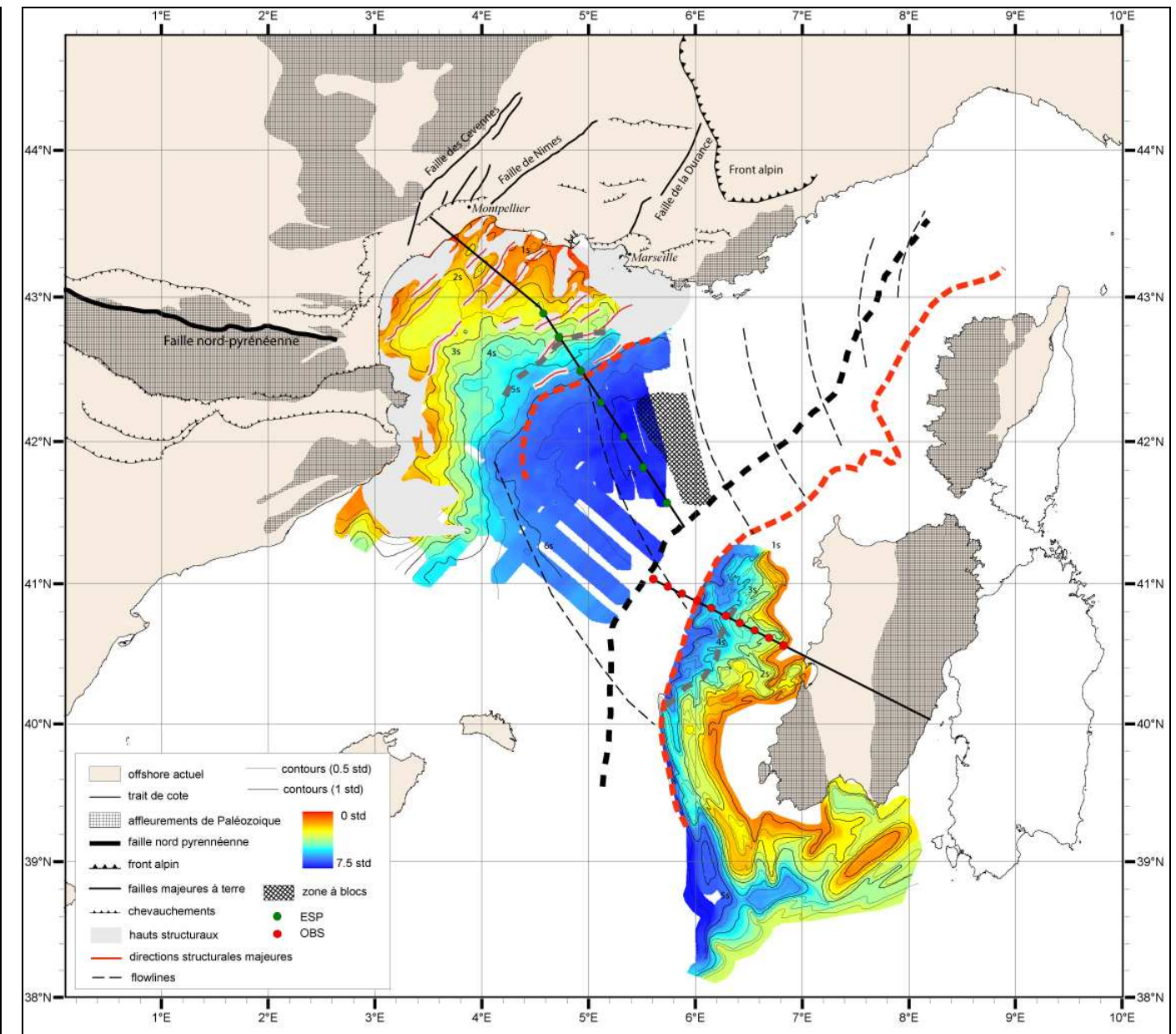
Figure II-20: Reconstruction intermédiaire par fermeture du domaine à fortes anomalies magnétiques (domaine IV) du bloc Corso-Sarde par rapport à l'Europe fixe. Le substratum Sarde (Thomas, 1986) a été roté avec le bloc Corso-Sarde ainsi que le profil Sard04 et ses OBS. Position du bloc Corso Sarde d'après Gueguen (1995).
