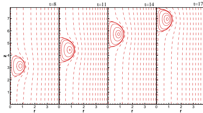
FIG. 3.24 – Phase de post-formation : lignes de courant \psi .
