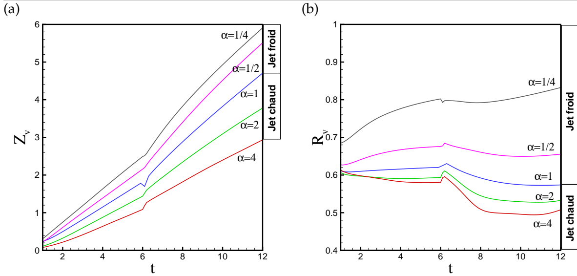
FIG. 7.22 –   volution temporelle de : (a) la coordonn  e axiale, (b) rayon du centroide du tourbillon.
