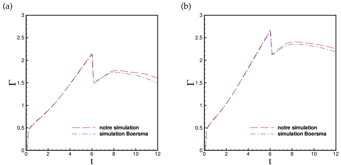
FIG. 7.41 – Évolution temporelle de la circulation : (a) \alpha = 4 , (b) \alpha = 2 .
