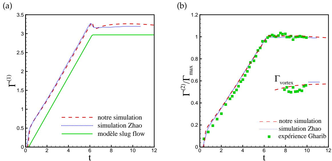
FIG. 3.13 – (a) évolution temporelle de la circulation \Gamma^{(1)} ; comparaison avec le modèle de slug-flow ( \Gamma^{slug} ) et les simulations de Zhao et al. (2000). (b) Évolution de la circulation \Gamma^{(2)} et du \Gamma_{vortex} ; comparaison avec les simulations de Zhao et al. (2000) et les résultats expérimentaux de Gharib et al. (1998).
