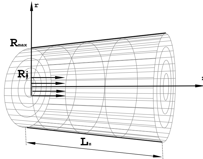
FIG. 5.1 – Domaine de calcul cylindrique ( \Omega ).
