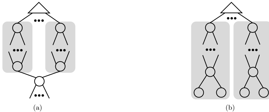
FIG. 7.6 – Blocs d'activité issus de SwitchNode
