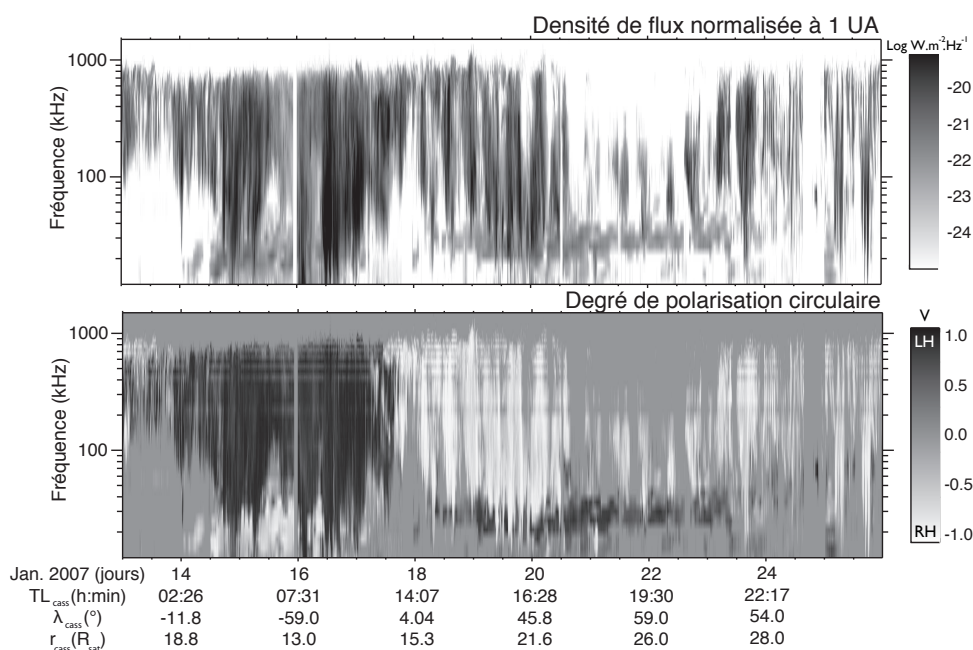
FIG. 6.4: Spectres dynamiques de la densité de flux S normalisée à 1 UA et du taux de polarisation circulaire normalisé V sur une période de 13 jours en janvier 2007. Lorsque Cassini parcourt les hautes latitudes nord ( \lambda_{cass} \geq 55^\circ ), le SKR disparaît aux hautes ( \geq 300 kHz) et basses ( \leq 40 kHz) fréquences. Les émissions observées aux basses fréquences ( \leq 40 kHz) avec une polarisation inverse à celle du SKR dominant correspondent au n-SKR décrit au chapitre 2 et ne sont pas considérées ici.
