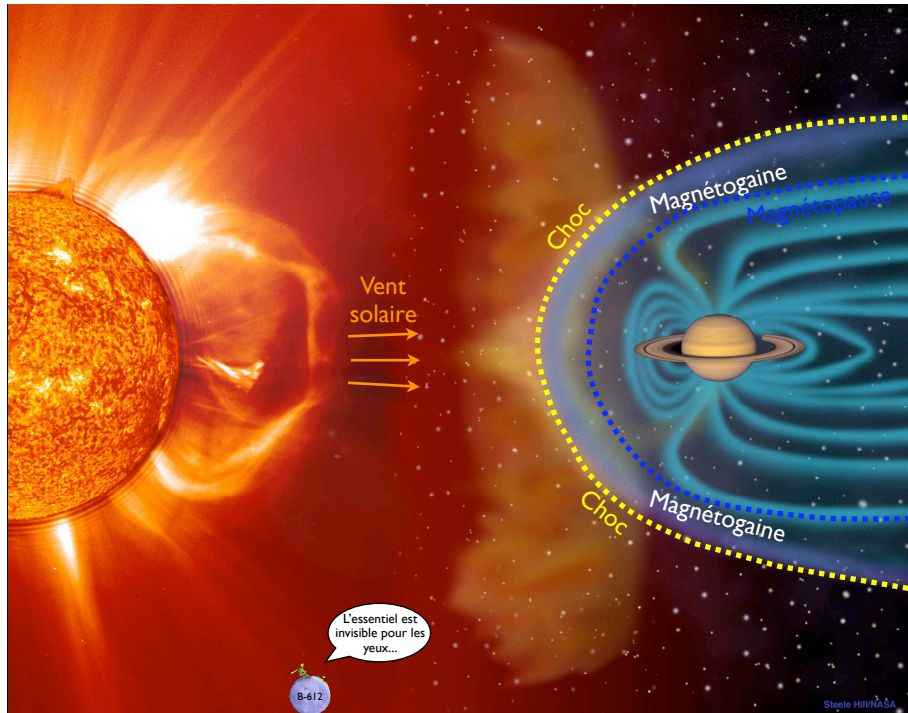
FIG. 1.1: Magnétosphère de Saturne.
