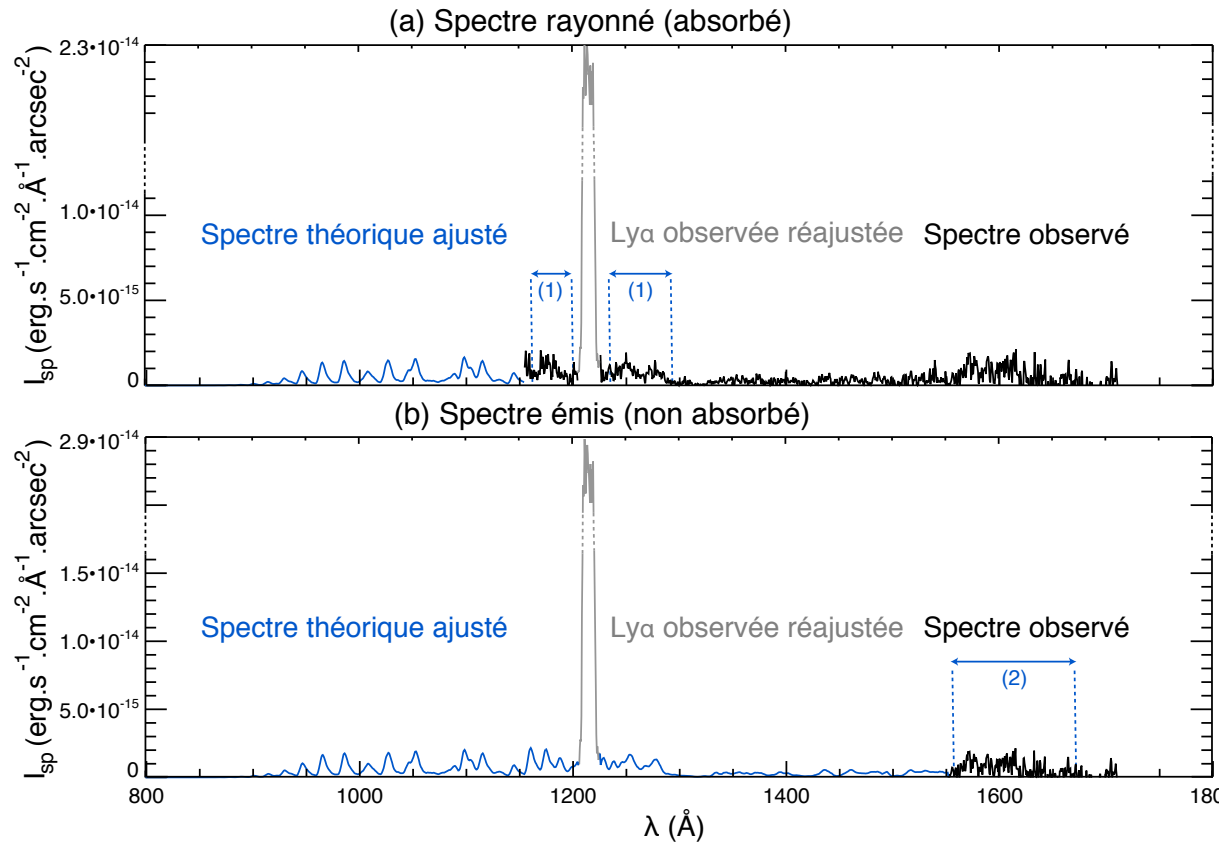
FIG. D.2: Spectres rayonné (a) et émis (b) reconstruits à partir du spectre moyen de l'émission de l'ovale côté disque obtenu à partir de l'observation o5dta1tpq du 8 décembre 2000 et de l'équation D.1. (a) La courbe noire indique le spectre mesuré initial I_{sp}(\lambda) . La courbe grise correspond à la normalisation de la raie Ly_{\alpha} par le facteur 1.5 permettant de tenir compte de l'émission réelle de Ly_{\alpha} , sous-estimée par l'utilisation de la largeur spatiale apparente de l'ovale pour les émissions de H_2 . La courbe bleue indique le spectre théorique de H_2 ajusté sur le spectre observé grâce aux intervalles de \lambda correspondant aux bandes de Werner de H_2 situées de part et d'autre de Ly_{\alpha} (zones indiquées par des traits en pointillés et l'indice (1)). Comme la zone (1) caractérise l'émission absorbée, le spectre reconstruit représente l'émission totale des raies électroniques de H_2 et H pour Ly_{\alpha} qui parvient à l'observateur après absorption par l'atmosphère, c'est-à-dire l'émission rayonnée. (b) La courbe noire indique le spectre mesuré. La courbe bleue montre le spectre théorique de H_2 ajusté sur le spectre observé sur l'intervalle de longueur d'onde correspondant aux bandes de Lyman de H_2 (indiqués par des traits en pointillés et l'indice (2)) qui ne sont pas absorbés par l'atmosphère. Sous l'hypothèse que la raie Ly_{\alpha} est absorbée comme les raies de H_2 , la courbe grise montre la raie Ly_{\alpha} réajustée pour tenir compte d'une part de l'absorption (par le rapport du coefficients d'ajustement calculé pour la zone (2) sur celui calculé pour la zone (1), ici \sim 1.06 ) et d'autre part du coefficient 1.5 (voir partie D.2.3). Le spectre final représente l'émission totale réelle émise par la source aurorale (avant absorption).
