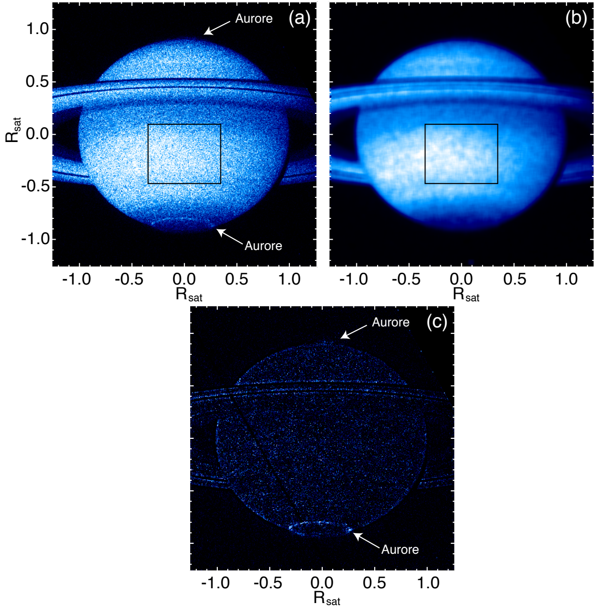
FIG. 4.2: Exemple de soustraction du modèle empirique de réfléchi solaire sur l'image HST-STIS-F115 enregistrée le 23 janvier 2007 à 4h41. Les images sont tracées dans le plan d'observation lié à la planète et l'échelle d'intensité est arbitraire et commune aux trois panneaux. Le panneau (a) montre l'image après soustraction de la diffusion géocoronale. Les émissions aurorales sont visibles mais peu contrastées (en particulier au nord). Le panneau (b) représente le modèle de fond de la figure 4.1c lissé sur 20 pixels. L'application d'une telle moyenne a pour effet d'atténuer les fluctuations d'intensité visibles aux petites échelles spatiales pour ne garder que des variations typiques continues en fonction du temps local et de la latitude. Les rectangles noirs sur les panneaux (a) et (b) délimitent les régions où l'on estime l'intensité du flux solaire réfléchi par le disque. Le rapport de ces deux valeurs sert à étalonner le fond (b) sur l'image (a) : ici le fond semble plus intense que l'image (le calcul donne un facteur normalisation de 0.9). Le panneau (c) montre le résultat de la soustraction du fond (b) à l'image (a) pondérée par le facteur correctif précédent. Une fois le fond soustrait, la moyenne de l'intensité du disque est voisine de 0 et les émissions aurorales apparaissent comme beaucoup plus contrastées. L'effet de lissage du modèle de réfléchi conduit à une soustraction imparfaite au limbe qui se traduit par une surbrillance lorsqu'on ne considère que les valeurs de flux positives mais dont la contribution est nulle en moyenne lorsqu'on considère également les valeurs de flux négatives.
