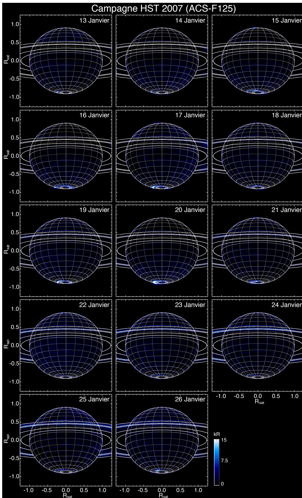
FIG. 4.5: Variabilité de l'ovale auroral moyen (calculé à partir de toutes les images de chaque journée pour augmenter le rapport signal sur bruit) observé par l'instrument ACS doté du filtre F125 lors de la campagne de Janvier 2007. Le réfléchi solaire a été soustrait.
