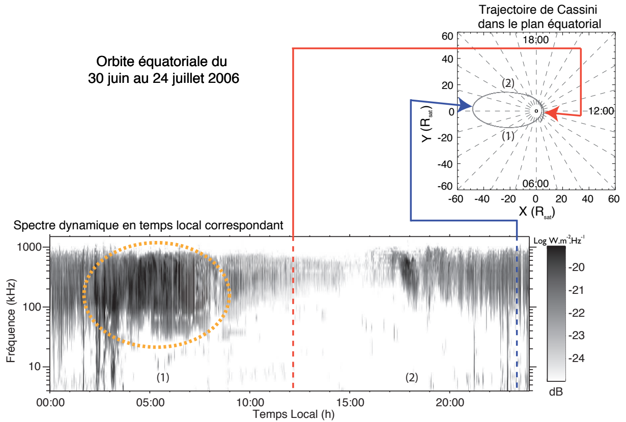
FIG. 2.9: Spectre dynamique de la densité de flux S normalisée à 1 UA des 50 % des événements polarisés ( |V| \geq 0.4 pour obtenir un bon contraste) organisé selon le temps local TL_{cass} pour une orbite équatoriale complète de Cassini. Le panneau du haut indique que cette orbite a la particularité d'offrir une couverture quasiment symétrique entre les côtés "matin" [00:00,12:00] et "soir" [12:00,24:00]. Les lignes rouge et bleue indiquent le perikrone et l'apokrone de l'orbite situés à TL_{cass} \sim 12:00 et 24:00 . On observe des émissions plus intenses lorsque Cassini est située côté matin sur la gamme [02:00,09:00] (pointillés orange).
