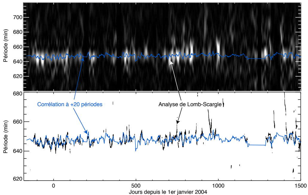
FIG. 3.2: Détermination comparée de la période variable de la composante LH du SKR sur 4.75 années (du 30 juin 2003 au 30 mars 2008) par les deux méthodes d'analyse détaillées dans l'annexe B. La série temporelle analysée correspond à la puissance émise intégrée entre 100 et 400 kHz avec une résolution temporelle de 3 min. Sur chacun des deux panneaux est indiquée en bleu la période calculée par la méthode de corrélation à N = +20 périodes. Le panneau (a) montre la représentation d'une analyse de Lomb-Scargle du signal. Chaque colonne, séparée de la suivante par un pas de temps de 30 min, correspond à une partie du périodogramme (ou spectre) de Lomb-Scargle calculé sur un intervalle de durée 10000 pts, soit \sim 21 jours. L'échelle d'intensité, qui indique la puissance spectrale (du noir au blanc pour une intensité croissante) est arbitraire. Le panneau (b) trace les maxima de chaque colonne en noir en excluant les points peu significatifs grâce à un seuil sur l'intensité spectrale. Chaque périodogramme a été suréchantillonné par rapport à la gamme de fréquence donnée par la FFT sur le même intervalle et sa résolution spectrale (donnée par la largeur à mi-hauteur du pic principal) vaut \sim 10 min à \sim 650 min (alors qu'elle vaut \sim 14 min pour le spectre issu de la FFT, voir l'annexe B). Sur chacun des panneaux, on voit que le pic des spectres (indiquant la période radio) se déplace avec le temps autour d'une valeur moyenne de \sim 650 min. Lorsque le périodogramme est suffisamment bien défini (grande intensité du pic, voir par exemple les intervalles des jours -180 à 180 ou 650 à 800, qui correspondent à des périodes où la latitude change peu), la courbe bleue passe précisément par les maxima des spectres associés.
