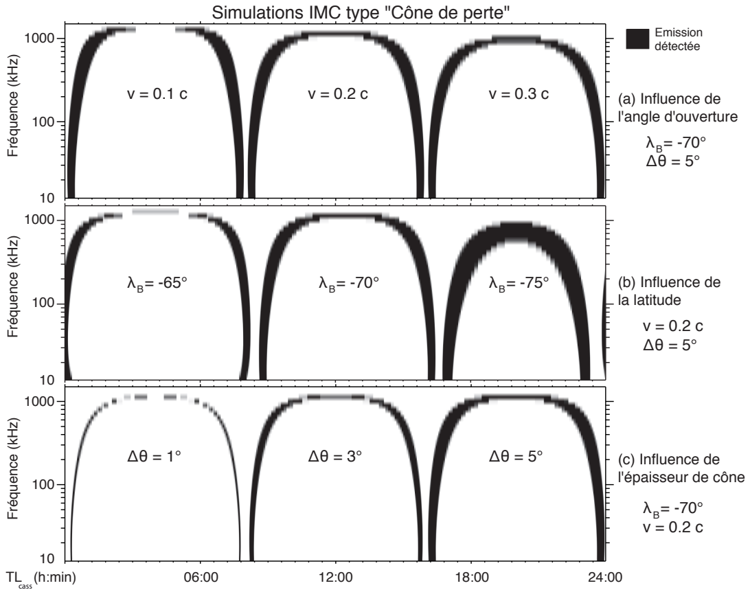
FIG. F.3: Spectres dynamiques organisés en temps local pour des simulations de type "Cône de perte". Les sources sont choisies au sud à TL_B = 04:00, 12:00 et 20:00 . Précisons que le temps local ne joue aucun rôle mais sert uniquement à simuler trois sources différentes sur un même spectre dynamique. Les panneaux (a), (b) et (c) illustrent l'influence de l'angle d'ouverture \theta(f) (variant avec la fréquence et proportionnel à la vitesse des électrons résonants v ), de la latitude \lambda_B de la ligne de champ et de la largeur de cône \Delta\theta sur les émissions simulées. Dans tous les cas, ces dernières prennent la forme d'arcs.
