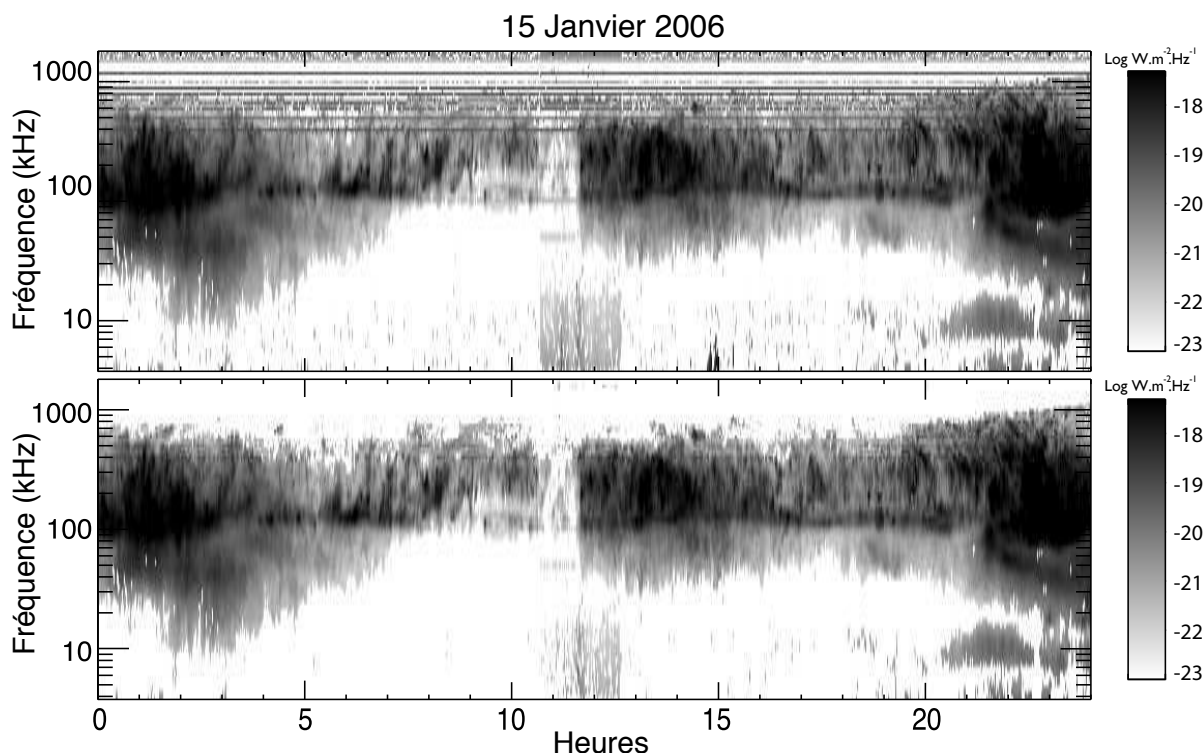
FIG. A.3: Spectres dynamiques (cartes d'intensité temps-fréquence) de la densité de flux S exprimée en W.m^{-2}.Hz^{-1} . Le panneau (a) montre les émissions correspondant à la condition 0.2 \leq |V_G| \leq 1.1 . Le panneau (b) trace les émissions avec la sélection additionnelle 0.2 \leq |V_P| \leq 1.1 . Cette seconde sélection permet d'éliminer plus efficacement les parasites radio (bandes de fréquences horizontales multiples de 100 kHz) ainsi que les émissions électrostatiques locales (visibles autour de 15 h). Les spectres ont été réinterpolés en fréquence après suppression des bandes de fréquence parasitées.
