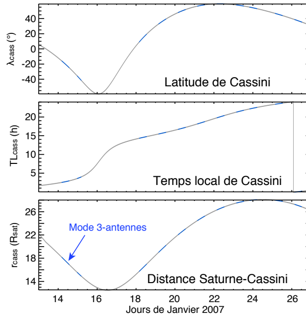
FIG. 2.5: Paramètres orbitaux de Cassini entre le 13 et le 26 janvier 2007. Les parties en bleu correspondent au fonctionnement du HFR en mode 3-antennes.
