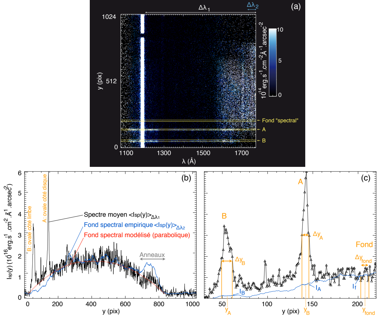
FIG. D.1: Etapes du calcul du spectre moyen I_{sp}(\lambda) pour l'émission de l'ovale "côté disque" (notée A) et "côté limbe" (notée B), suivant l'équation D.1. (a) montre le spectre bi-dimensionnel y(\lambda) utilisé comme exemple de référence dans cette annexe. Ce spectre comprend la contribution des émissions aurorales A et B ainsi que celle du flux solaire réfléchi par le disque. Les lignes oranges indiquent la largeur spatiale caractéristique apparente de l'émission \Delta y . Par ailleurs, \Delta\lambda_1 et \Delta\lambda_2 indiquent les deux intervalles de longueur d'onde utilisés pour calculer d'une part le spectre spatial moyen de H_2 \langle I_{sp}(y) \rangle_{\Delta\lambda_1} (excluant L\gamma_\alpha ) et d'autre part que le fond spatial moyen \langle I_{sp}(y) \rangle_{\Delta\lambda_2} estimé en bord de spectre sur la gamme [1680,1715 \text{\AA} ]. (b) montre le tracé de \langle I_{sp}(y) \rangle_{\Delta\lambda_1} (en noir), du fond spatial moyen normalisé \langle I_{sp}(y) \rangle_{\Delta\lambda_2} (en bleu, lissé sur 30 pixels consécutifs et normalisé à \langle I_{sp}(y) \rangle_{\Delta\lambda_1} sur l'intervalle [1250,1485 \text{\AA} ]) ainsi que du fond spatial modélisé (en rouge) par une fonction parabolique. (c) est un zoom de (b) sur l'intervalle de y concernant les émissions aurorales (A et B). La valeur de y servant à calculer le fond spectral moyen en dehors des aurores est définie par l'intersection entre les courbes bleue et noire. Les valeurs I_A , I_B et I_f correspondent à la valeur de \langle I_{sp}(y) \rangle_{\Delta\lambda_2} pour y = y_A \pm \Delta y_A/2 , y_B \pm \Delta y_B/2 et y_{fond} \pm \Delta y_{fond}/2 (en pratique \Delta y_{fond} = \Delta y_A ou \Delta y_B ).
