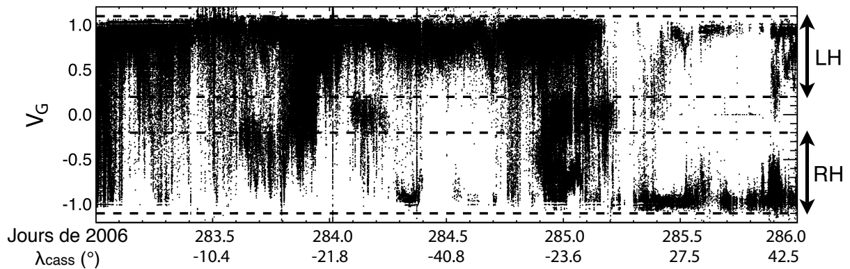
FIG. A.2: Taux normalisé de polarisation circulaire V_G calculé à partir de l'inversion Goniométrique. Seuls les points possédant un SNR supérieur à 25 dB (simultanément sur chacune des 2-antennes) sont tracés. Les lignes en tiretés indiquent les gammes de sélection du SKR : 0.2 \leq V_G \leq 1.1 pour la composante LH et -1.1 \leq V_G \leq -0.2 pour la composante RH. Ces limites permettent de rejeter la plupart des émissions non polarisées. Le signe de la polarisation dominante change avec la latitude de Cassini.
