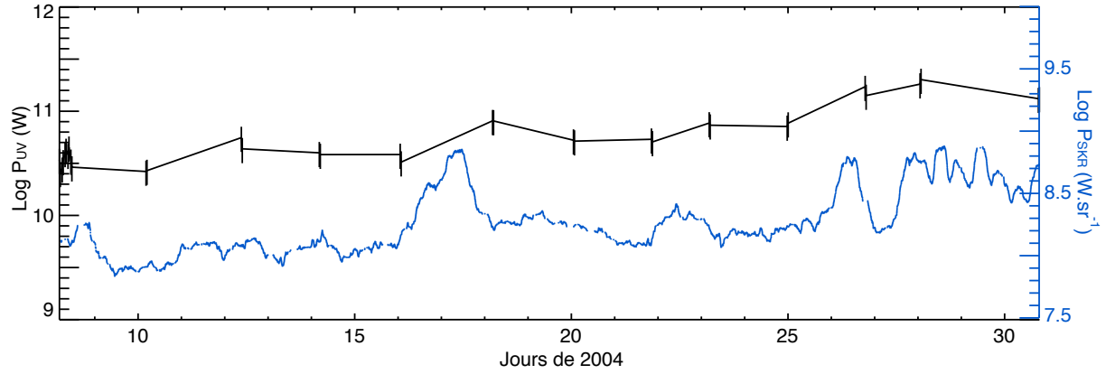
FIG. 4.12: Tracé comparatif des puissances UV (en W) déduites des images HST de la campagne 2004 et de la puissance totale du SKR (intégrée entre 3 kHz et 1500 kHz et exprimée en W.sr^{-1} ) lissée sur une période (prise égale à 648 min). Le coefficient de corrélation du logarithme décimal de ces deux séries vaut C = 0.87 .
