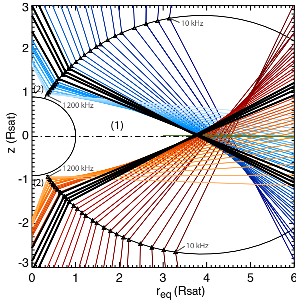
FIG. 6.3: Vue méridienne de Saturne et d'une ligne de champ magnétique de latitude \lambda_B = -70^\circ . Cette ligne est peuplée d'une source nord (échelle de couleur bleue) et d'une source sud (échelle de couleur rouge) conjuguées sur la même ligne de champ et chacune constituée de points source (triangles) dans la gamme [10,1200 kHz]. Pour chaque point source sont représentées les deux directions de son cône d'émission, en coupe méridienne, calculé dans le cas "cône de perte" : plus on s'approche de la planète, plus le champ augmente, plus f \sim f_{ce} augmente et plus \theta(f) diminue. Les fréquences entre 200 kHz et 400 kHz, correspondant à l'extension minimale de la zone d'ombre équatoriale, sont représentées en noir. Les indices (1) et (2) indiquent les zones d'ombre équatoriale et polaires. La trajectoire de Cassini correspondant à la traversée de la zone d'ombre équatoriale de la figure 6.2 est représentée par la courbe verte.
