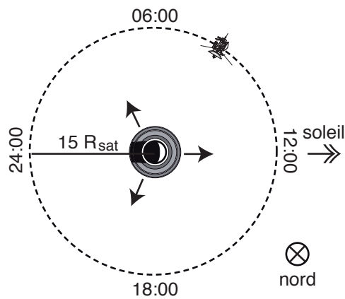
FIG. F.2: Vue du pôle sud d'un orbiteur circulaire à 15 R_{sat} situé dans le plan équatorial et observant des sources situées dans l'hémisphère sud à TL_B = 04:00, 12:00 and 20:00 (flèches noires).
