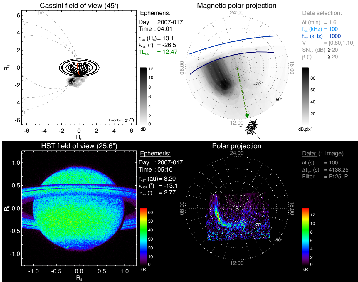
FIG. 5.6: Images radio et UV du 17 janvier 2007 à 04 h 01 min intégrées sur une durée de 100 s. Les éphémérides correspondantes de Cassini et du HST sont indiquées au centre. Les deux panneaux du haut montrent les images radio (voir annexe E) respectivement dans le plan d'observation de Cassini et en projection polaire magnétique à la surface de la planète, utilisant une sélection de données précisée à droite. Cette sélection est sévère pour ne prendre en compte que les sources les plus intenses et fortement polarisées pour toutes les fréquences du SKR entre 100 et 1000 kHz (des effets de réfraction sont probables au dessous de 100 kHz). Sur l'image de gauche le méridien de temps local midi est indiqué en rouge tandis que sur celle de droite (organisée en temps local) TL_{\text{cass}} est indiqué par une flèche verte. Les lignes de champ magnétique notées (1), (2) et (3) ont respectivement un pied de coordonnées \lambda_B = -75^{\circ} et TL_B = 06:00, 08:00 et 10:00 . Les lignes bleues indiquent les horizons radio correspondant aux fréquences limites de la gamme sélectionnées : 100 kHz et 1000 kHz. Les deux panneaux du bas montrent l'image UV brute correspondant aux données indiquées à droite et sa projection polaire après soustraction du réfléchi solaire et correction de l'angle de phase.
