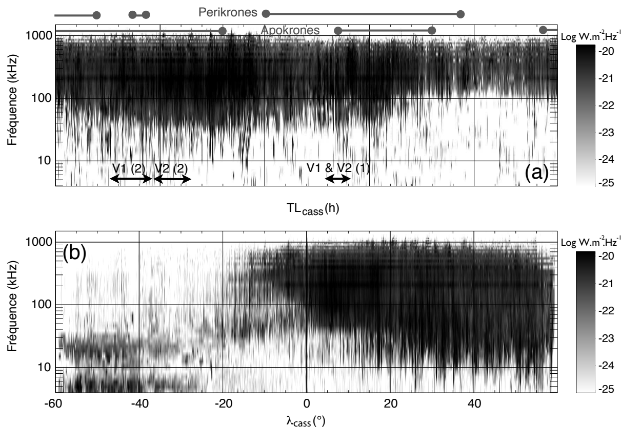
FIG. 2.8: Spectres dynamiques de la densité de flux S normalisée à 1 UA des 50 % des événements les plus polarisés ( |V| \geq 0.8 ) pour la période allant du 29 juin 2004 au 30 mars 2008. (a) Intensité du SKR en fonction du temps local de l'observateur TL_{cass} et de la fréquence, calculée pour des observations équatoriales ( |\lambda_{cass}| \leq 1^\circ ). Les gammes de temps locaux explorées par les sondes Voyager sont indiquées par des doubles flèches noires où les indices (1) et (2) indiquent respectivement les trajectoires pré- et post-rencontre. Les gammes des apokrones et perikrones des orbites de Cassini sont indiquées en gris. (b) Intensité du SKR en fonction de la latitude \lambda_{cass} et de la fréquence, calculée à partir de toutes les données disponibles sur 3.75 années.
