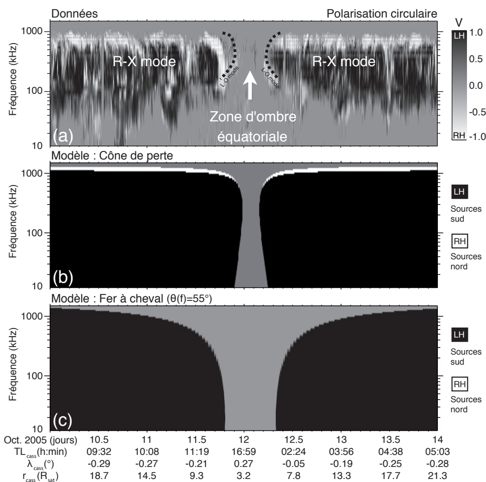
FIG. 6.2: Spectres dynamiques du SKR observés et simulés sur une durée de quatre jours de l'année 2005, incluant une traversée de la zone d'ombre équatoriale. Le panneau (a) montre le taux de polarisation circulaire normalisé V . Les courbes en pointillés indiquent la variation de la disparition du signal avec la fréquence. Ils ajustent le mode dominant R-X (voir chapitre 2). Les zones blanches détectées entre 100 et 300 kHz et situées "sous" les courbes en pointillés au voisinage du 12 octobre correspondent à des émissions identifiées au mode L-O [Cecconi et al., 2008]. Les panneaux (b) et (c) montrent les spectres simulés pour les émissions obliques données par les distributions "cône de perte" et "fer à cheval" (avec \theta(f) = 55^\circ ). Les sources sont distribuées à toutes les longitudes sur des lignes de champ pour lesquelles \lambda_B = -70^\circ et dans les deux hémisphères (correspondant donc à deux ovales circulaires circumpolaires). Les autres paramètres de simulation sont indiqués dans le tableau 6.1
