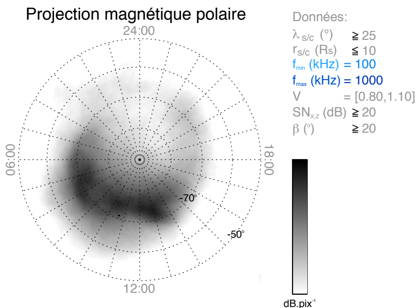
FIG. 5.9: Ovale radio statistique déduit des 11.7 jours d'observation cumulés (durant lesquels la sonde a observé tous les temps locaux) en mode 2-antennes pour les sélections indiquées à droite entre le 31 juin 2004 et le 31 décembre 2007. Les données de l'hémisphère nord et de l'hémisphère sud ont été utilisées ensemble sur une seule et même projection sous l'hypothèse d'une conjugaison magnétique des sources. On a donc une incertitude intrinsèque de \Delta\lambda_B \sim 2^\circ due au modèle de \mathbf{B} sur la latitude de l'émission. Un seuil a été appliqué pour augmenter le contraste.
