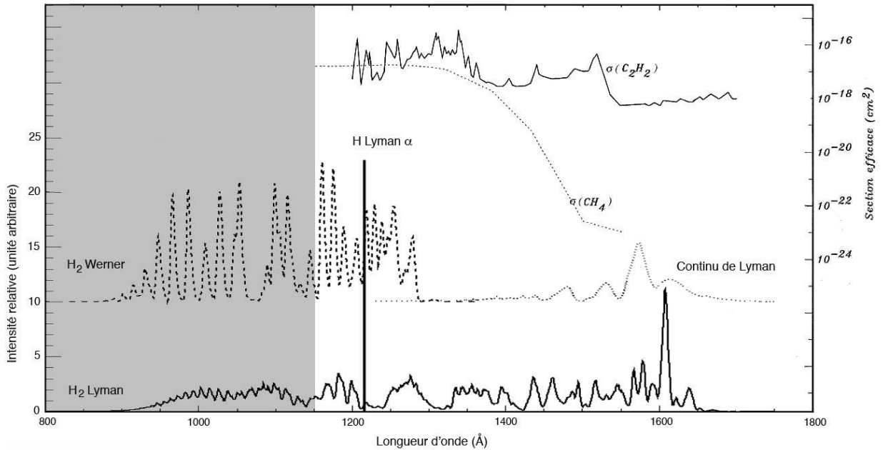
FIG. 4.10: Spectre théorique des raies électroniques de H_2 (Shemansky, communication personnelle) donné dans une échelle arbitraire. La section efficace \sigma (échelle de gauche) est superposée pour deux hydrocarbures absorbants dominants : dans l'ordre CH_4 et C_2H_2 . On voit qu'elle chute au delà de 1500 Å pour le méthane et 1550 Å pour l'acétylène.
