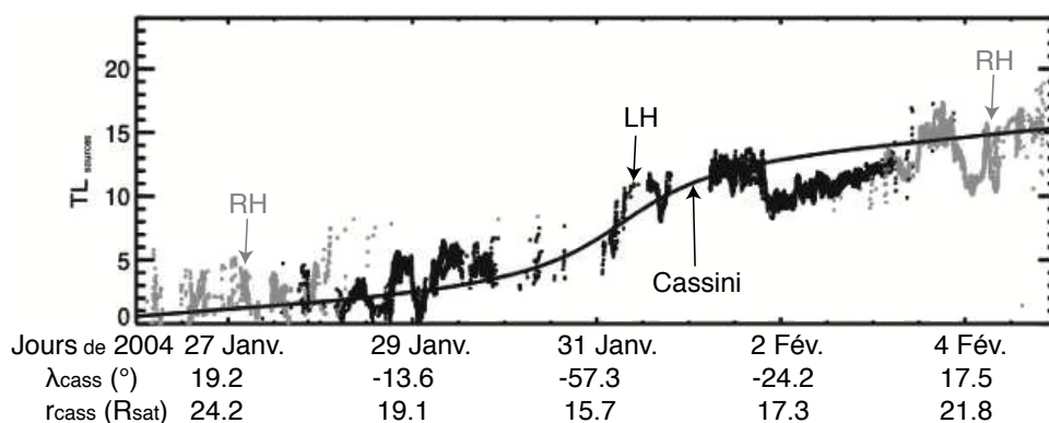
FIG. 3.5: Temps local des sources observées par Cassini. Les points correspondent au tracé TL(t) pour chaque fréquence dans la gamme [117.6, 249.6 kHz] et lissé sur 10 points consécutifs. Une sélection préalable a été appliquée : le flux des mesures retenues est supérieur au flux médian (voir chapitre 2) et sa polarisation circulaire est supérieure en valeur absolue à V_{\min} = 0.8 . La courbe en trait plein indique le temps local de Cassini. La partie grise correspond à l'émission RH (observé préférentiellement dans l'hémisphère nord) et la partie noire à l'émission LH (observé préférentiellement dans l'hémisphère sud). Les sources observées ont des temps locaux voisins de celui de Cassini. Les variations de temps local sont homogènes pour toutes les fréquences étudiées. Les brusques variations observées (par exemple le 29 janvier ou le 2 février) pourraient être la manifestation de la visualisation du mouvement des sources en temps réel.
