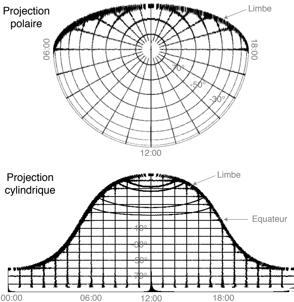
FIG. C.4: Projections polaire et cylindrique de la grille de coordonnées ajustée à la surface de la planète le 26 janvier 2004 à 19h16 (image des figures C.2e,f,g et C.3). L'incertitude intrinsèque à la méthode de projection peut se mesurer à l'épaisseur apparente de la grille projetée au niveau du limbe. On peut comparer notre projection polaire à celle de la figure 2 de Grodent et al. [2005] qui montrait à la fois une résolution de projection moins bonne (bien visible au limbe) et des valeurs de latitudes faussées (de 2 à 3° au maximum) provenant d'une équation de l'ellipsoïde utilisant la latitude planétographique au lieu de la latitude planétocentrique.
