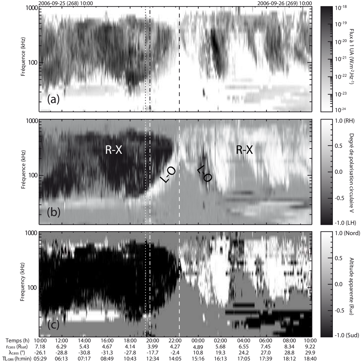
FIG. 5.2: Spectres dynamiques du flux du SKR normalisé à 1 UA (en \text{W.m}^{-2}.\text{Hz}^{-1} ) (a), du taux de polarisation circulaire V (b) et de l'hémisphère apparent des sources (c) fourni par l'analyse goniopolarimétrique dans le plan d'observation. Les données des panneaux (a) et (b) sont issues du traitement détaillé dans l'annexe A : elles correspondent à une exclusion des données |V| \leq 0.2 . Sur le panneau (c), l'altitude apparente z (telle que définie à la figure E.1) est saturée aux valeurs -1 et 1 de façon à faire ressortir l'hémisphère d'origine de l'émission plutôt que son altitude projetée.
