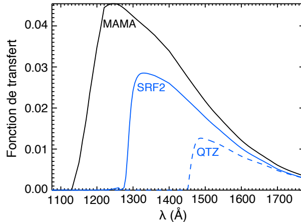
FIG. D.3: Fonction de transmission des trois filtres MAMA (noir), SRF2 (bleu) et QTZ (tiretés bleus) de l'imager de l'instrument STIS. Ils sont respectivement comparables aux trois filtres F115, F125 et F140 de l'imager ACS utilisé depuis 2007. Les filtres SRF2 et QTZ permettent, respectivement, d'exclure l'émission dominante de Ly \alpha et d'isoler les photons \lambda \geq 1450 Å qui ne subissent aucune absorption par les hydrocarbures atmosphériques. Ce dernier filtre fournit ainsi des images dont l'intensité est directement proportionnelle au flux d'électrons (ou d'ions) qui précipitent dans la magnétosphère.
