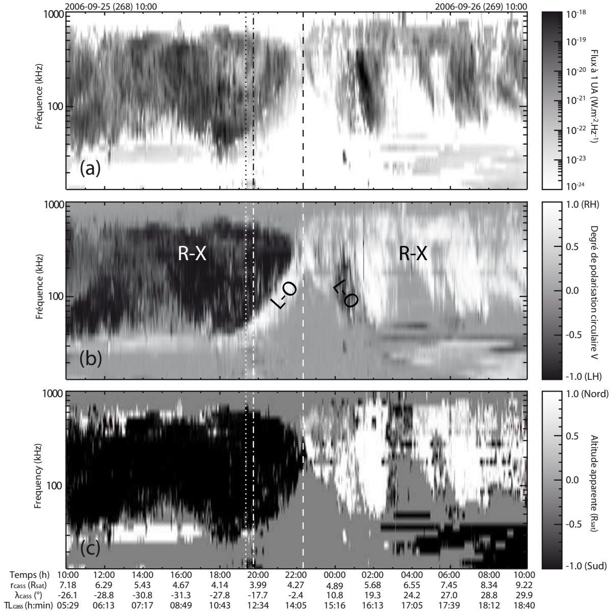
FIG. 5.2: Spectres dynamiques du flux du SKR normalisé à 1 UA (en \text{W}\cdot\text{m}^{-2}\cdot\text{Hz}^{-1} ) (a), du taux de polarisation circulaire V (b) et de l'hémisphère apparent des sources (c) fourni par l'analyse goniopolarimétrique dans le plan d'observation. Les données des panneaux (a) et (b) sont issues du traitement détaillé dans l'annexe A : elles correspondent à une exclusion des données |V| \leq 0.2 . Sur le panneau (c), l'altitude apparente z (telle que définie à la figure E.1) est saturée aux valeurs -1 et 1 de façon à faire ressortir l'hémisphère d'origine de l'émission plutôt que son altitude projetée.
