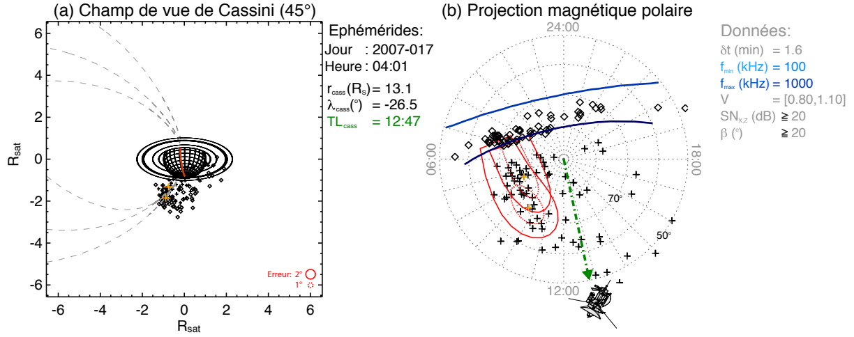
FIG. E.2: Localisation des sources radio et des lignes de champ magnétique associées. Les éphémérides de Cassini sont indiquées au centre et les paramètres de sélection des données à droite. (a) donne les directions d'arrivée sélectionnées dans le plan d'observation de Cassini. Les croix indiquent celles qui interceptent l'iso-surface f = f_{ce} et les losanges celles qui ne l'interceptent pas. L'erreur angulaire sur la position des sources est indiquée par les cercles rouges (en pointillés pour \Delta\theta, \phi = 1^{\circ} et en trait plein pour \Delta\theta, \phi = 2^{\circ} ). Le méridien rouge indique le temps local midi. Les tiretés gris représentent les lignes de champ magnétique dont les pieds ont les coordonnées (\lambda_B, TL_B) = (-75^{\circ}, 06:00) , (-75^{\circ}, 08:00) et (-75^{\circ}, 10:00) . La distribution des sources est organisée approximativement autour de ces lignes de champ. (b) indique la position à la surface de la planète du pied des lignes de champ associées aux sources radio. La flèche verte sur cette projection polaire magnétique donne le temps local de Cassini. Les croix oranges illustrent trois positions particulières (déjà repérées sur le panneau (a)) entourées de leur barre d'erreur projetée en rouge. Les lignes bleues correspondent aux horizons radio des fréquences limites de la gamme sélectionnée (pour une fréquence, on ne peut pas 'voir' de source située derrière son horizon radio). Les losanges correspondent aux points qui n'interceptent pas leur iso- f_{ce} . Ils s'accumulent le long de leur horizon radio respectif.
