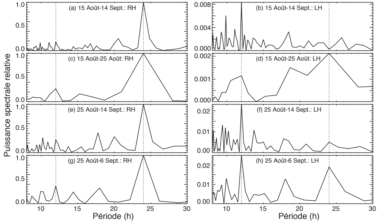
FIG. 3.11: Spectres de Fourier des séries de puissances RH et LH (tracées sur la figure 3.9) pour différents intervalles de temps. Les panneaux (a,b) portent sur la totalité du survol. Les panneaux (c,d) sur la période avant le 25 août et les panneaux (e,f,g,h) sur deux périodes différentes après le 25 août (incluant ou excluant les deux derniers jours de données, très parasites). Les lignes en pointillés indiquent les périodes 12 h et 24 h. Chaque paire de spectres RH/LH est normalisée par la valeur du pic le plus intense dans le spectre RH. L'échelle horizontale est linéaire en fréquence, donc non linéaire en période ( 1/f ) ce qui explique pourquoi les pics à 24 h sont plus larges que ceux à 12 h.
