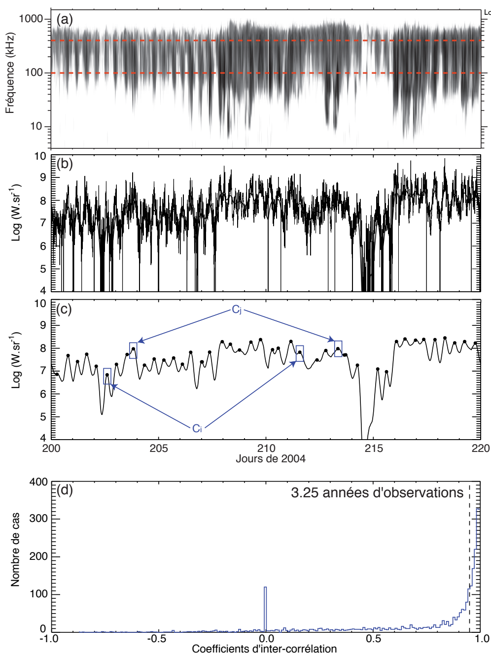
FIG. B.1: Exemple du traitement des données permettant d'estimer précisément P_{skr} sur un intervalle de N périodes. Le panneau (a) montre un spectre dynamique de l'émission kilométrique de l'hémisphère sud (composante LH polarisée à gauche) pendant 20 jours d'observation. Les lignes rouges en tirets indiquent la gamme de fréquences [100,400 kHz] correspondant à la partie la plus intense du spectre du SKR. Le panneau (b) trace la série temporelle de puissance associée intégrée entre 100 et 400 kHz. La courbe noire superposée correspond à la même série lissée deux fois consécutivement sur un intervalle glissant de 5 h. Ce traitement permet d'éliminer les fluctuations de haute fréquence et faire ressortir la variation principale modulée à P_{skr} . Le panneau (c) indique par des points noirs les maxima locaux de la série lissée, détectés automatiquement. Pour chaque point, on calcule alors le coefficient d'intercorrélacion entre deux fenêtres larges de 6 h (boîtes bleues reliées par des flèches) dont l'une est centrée sur le maximum local considéré et l'autre sur le maximum situé N périodes plus loin. Ici, C_i et C_j illustrent le cas N = +20 . Le panneau (d) montre la distribution de ces coefficients d'intercorrélacion pour la composante LH et N = +20 sur 3.25 années d'observations correspondant à l'étude [Zarka et al., 2007]. Cette distribution témoigne d'un pic marqué proche de la valeur 1. Partant, on choisit par la suite un coefficient de corrélation limite C_{lim} = 0.95 correspondant à la largeur à mi-hauteur du pic afin de sélectionner uniquement les évènements les mieux corrélés.
