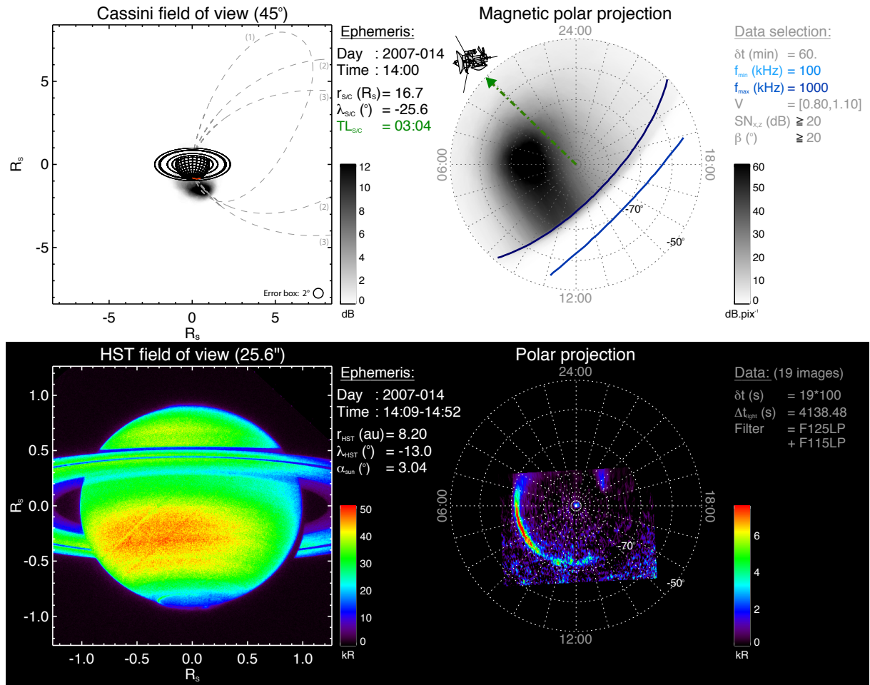
FIG. 5.8: Idem figure 5.7 pour la journée du 14 janvier. Les pieds des lignes de champ magnétique notées (1), (2) et (3) sur l'image radio en haut à gauche ont pour coordonnées : \lambda_B = -75^{\circ} et TL_B = 04:00, 06:00 et 08:00 .
