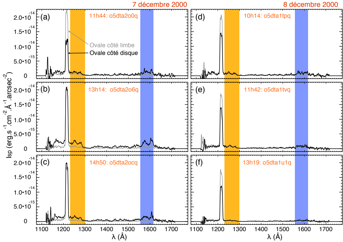
FIG. 4.11: Spectres de l'émission I_{sp} de l'ovale côté disque (en noir) et de l'ovale côté limbe (en gris) issus de six spectres 2D initiaux de la campagne d'observation de 2000 (voir tableau 4.2). Chaque spectre est en réalité un spectre moyen (calculé avec l'équation D.1, voir annexe D), lissé sur 5 valeurs consécutives. Les zones orange et violette indiquent les domaines de longueurs d'onde utilisés pour calculer les rapports de couleur et correspondant respectivement l'émission absorbée et l'émission non absorbée.
