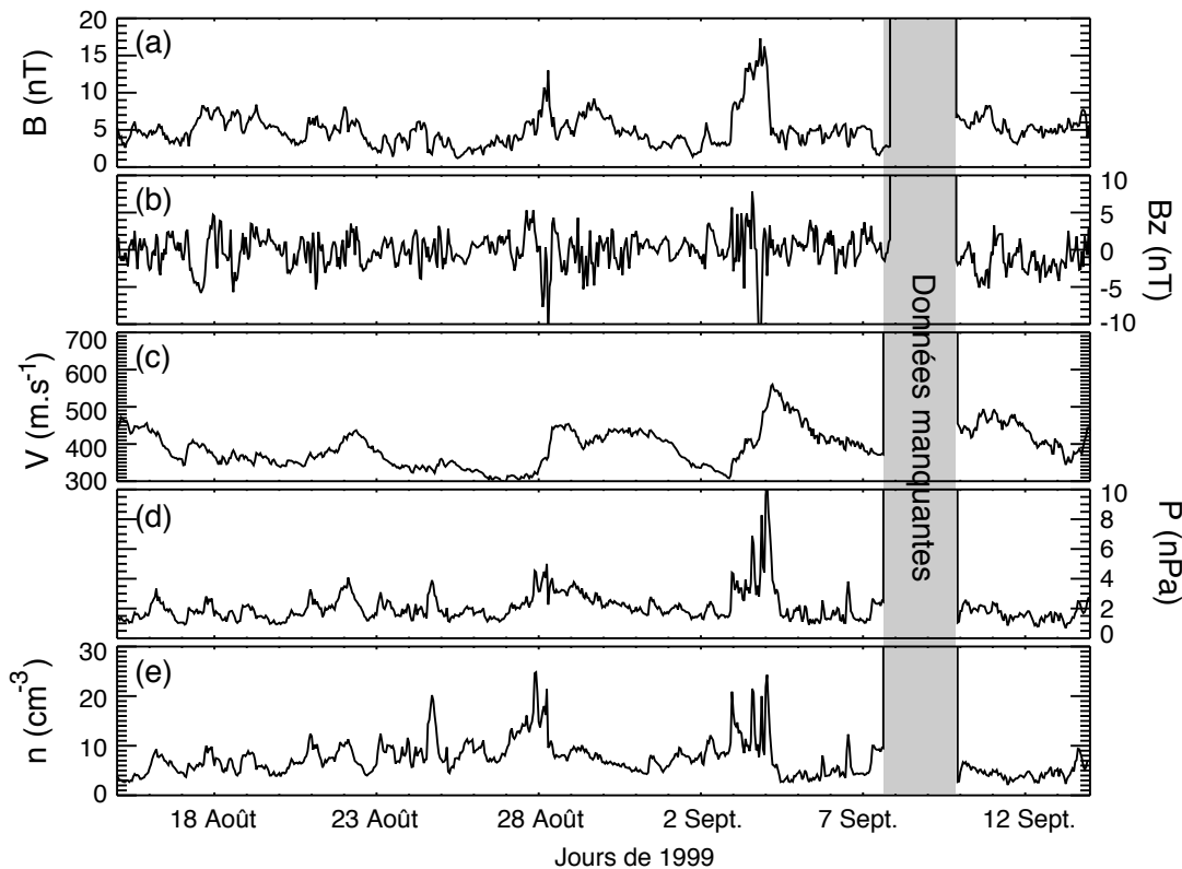
FIG. 3.12: Variations des paramètres du vent solaire (obtenus à partir du site http://omniweb.gsfc.nasa.gov/ ) pendant le survol de la Terre par Cassini mesurés par la sonde WIND au point de lagrange L1. (a) indique le module B du champ magnétique interplanétaire et (b) le module de sa composante B_z (normale à l'écliptique). (c,d,e) donnent respectivement la vitesse, la pression dynamique et la densité des protons dans le vent solaire. Aucune modulation à 24h n'est présente dans ces données. On remarque que globalement, l'activité du vent solaire est plus intense approximativement entre le 25-27 août et le 13 septembre.
