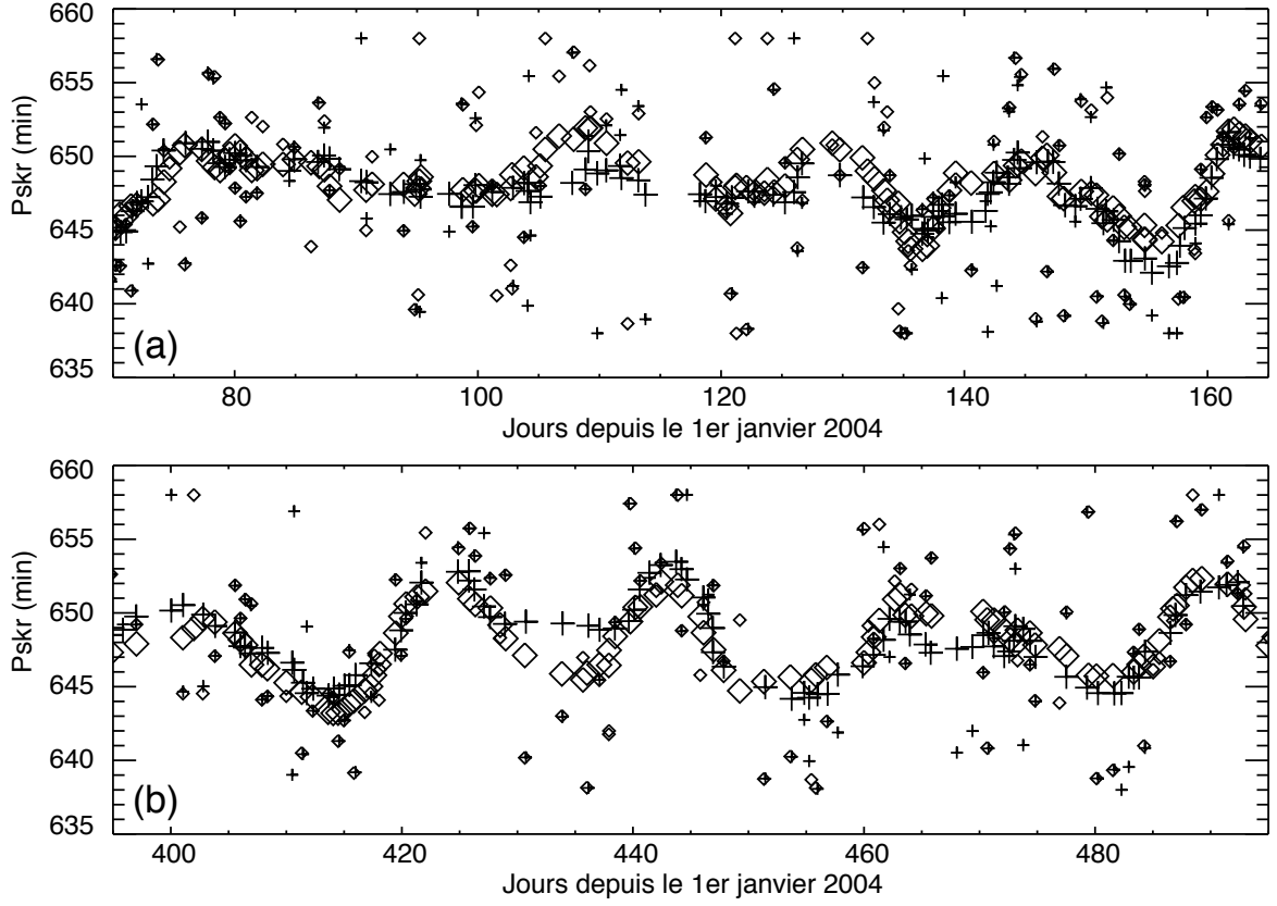
FIG. B.2: Détermination de P_{skr} de la composante LH sur deux périodes arbitraires de \sim 100 jours. Sur chacun des deux panneaux sont tracées les valeurs individuelles de P_{skr} calculées pour les coefficients de corrélation \geq C_{lim} (approximativement une valeur par rotation). Les petits symboles croix et losanges indiquent les valeurs calculées avec N = +20 et N = -20 respectivement. Les nuages de points correspondants montrent une variation de \pm 10 min à l'échelle de 20-30 jours avec des fluctuations de bruit de l'ordre de \pm 5 min. Si on lisse chacune de ces séries sur dix valeurs consécutives, on obtient les valeurs indiquées par les grands symboles losanges et croix. On voit alors que la modulation à 20-30 jours persiste (avec une amplitude de \pm 3-4 min pour le panneau (a) et \pm 7 min pour le panneau (b)) avec une amplitude des fluctuations de bruit réduite à \pm 1-1.5 min. La modulation de P_{skr} correspond ainsi à une détection à \sim 3\sigma pour le panneau (a) et \sim 5\sigma pour le panneau (b). Chaque mesure finale a donc été calculée avec des mesures étalées sur \sim 30 rotations ( |N| = 20 rotations initiales ajoutées à un lissage sur 10 valeurs consécutives), c'est-à-dire \sim 13 jours.
