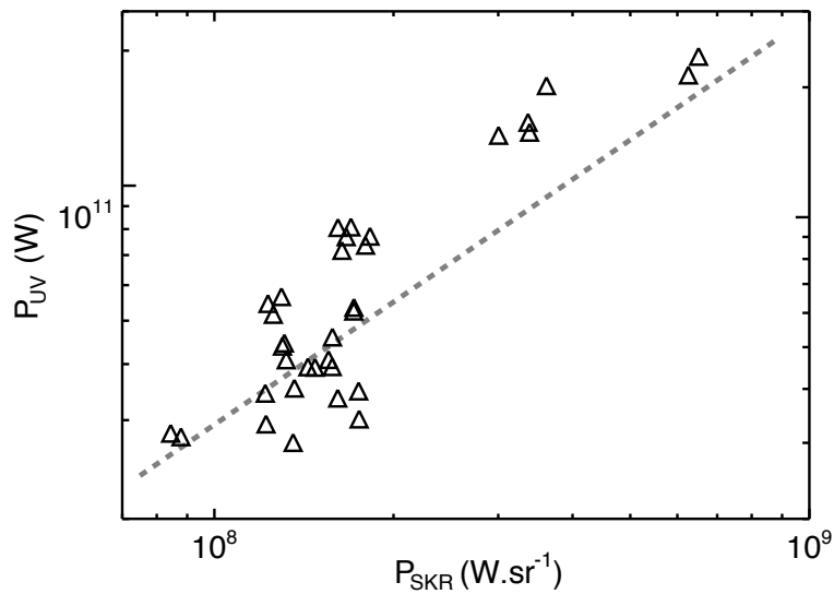
FIG. 4.13: Tracé de la puissance apparente totale de l'ovale UV en fonction de la puissance apparente du SKR en janvier 2004 (similaire à la figure 1c de Kurth et al. [2005]). Les barres d'erreur ne sont pas indiquées puisqu'elles ne sont pas connues pour l'émission radio dont l'anisotropie empêche d'évaluer quelle partie de la totalité des émissions est observée. La ligne en pointillés indique donc de façon qualitative la corrélation entre les émissions.
