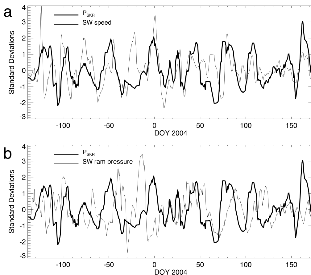
FIG. 3.4: Comparaison entre les variations de la période du SKR P_{skr} , la vitesse v_{vent\ solaire} (notée SW [solar wind] speed) et la pression dynamique (notée SW RAM pressure) P_{vent\ solaire} du vent solaire à la position de Saturne. L'intervalle représenté correspond à la phase d'approche de Cassini avant sa mise en orbite autour de la planète. Il n'y a donc pas d'influence périodique des paramètres orbitaux sur la visibilité de l'émission et cette période est la plus intéressante pour étudier directement l'influence du vent solaire sur P_{skr} . Pour clarifier la comparaison, les grandeurs tracées ont été préalablement corrigées de leur variation à long terme (par soustraction d'une moyenne glissante sur une durée de \sim 2 mois). Le panneau (a) superpose P_{skr} (en trait gras) et v_{vent\ solaire} (en trait fin). Excepté pour les intervalles d'une dizaine de jours autour des jours -25 et +65 (liés à des trous de données, une mésestimation partielle du temps de propagation balistique, ou l'occurrence de CME), la corrélation est forte avec une corrélation linéaire C \geq 40\% . Le panneau (b) superpose P_{skr} (en trait gras) et P_{vent\ solaire} (en trait fin). La corrélation est faible sur tout l'intervalle avec C \sim -10\% .
