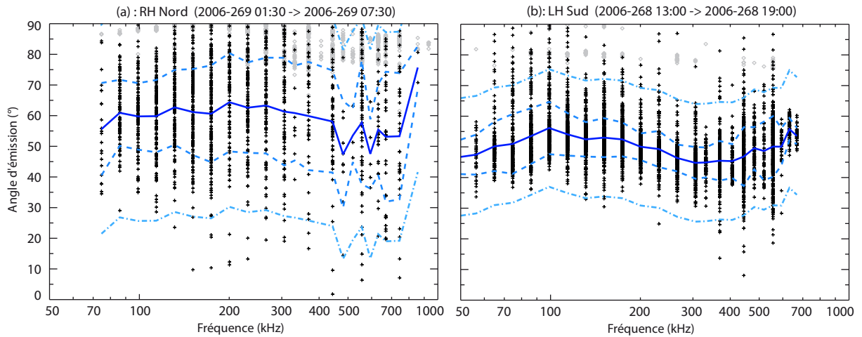
FIG. 5.5: Angle d'émission (entre la direction du champ magnétique à la source et la direction d'arrivée de l'onde) pour les sources nord (a) et sud (b) correspondant à un intervalle de 6 h précisé dans le titre de chaque panneau. Seules les données avec un taux de polarisation circulaire |V| \geq 0.9 ont été retenues. Les croix noires et les diamants gris représentent les directions d'arrivée qui interceptent ou non leur iso- f_{ce} (cf annexe E). Les courbes bleues en trait plein et en pointillés indiquent respectivement la moyenne et sa valeur \pm l'écart type calculées uniquement sur les croix. Les courbes mixtes en bleu clair montrent l'erreur maximale sur l'angle d'émission si on considère une barre d'erreur initiale de 2^\circ sur la direction d'arrivée de l'onde dans le plan des antennes.
