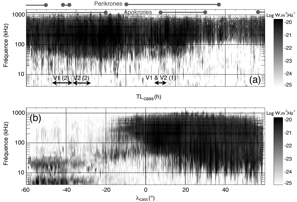
FIG. 2.8: Spectres dynamiques de la densité de flux S normalisée à 1 UA des 50 % des événements les plus polarisés ( |V| \geq 0.8 ) pour la période allant du 29 juin 2004 au 30 mars 2008. (a) Intensité du SKR en fonction du temps local de l'observateur TL_{cass} et de la fréquence, calculée pour des observations équatoriales ( |\lambda_{cass}| \leq 1^\circ ). Les gammes de temps locaux explorées par les sondes Voyager sont indiquées par des doubles flèches noires où les indices (1) et (2) indiquent respectivement les trajectoires pré- et post-rencontre. Les gammes des apokrones et perikrones des orbites de Cassini sont indiquées en gris. (b) Intensité du SKR en fonction de la latitude \lambda_{cass} et de la fréquence, calculée à partir de toutes les données disponibles sur 3.75 années.
