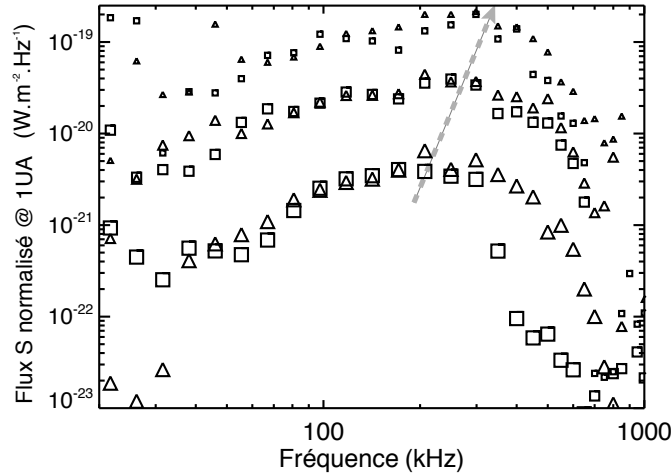
FIG. 3.6: Flux de l'AKR normalisés à 1 UA atteints 50, 10 et 1 % du temps (appelés niveaux d'occurrence), observés par Cassini lors du survol terrestre, représentés par les gros, moyens et petits symboles, en fonction de la fréquence. Les triangles indiquent la composante RH (hémisphère sud) et les carrés la composante LH (hémisphère nord). La flèche grise souligne le déplacement du pic spectral avec le niveau d'occurrence. Le décalage observé de 200 kHz à 300 kHz lors du passage des niveaux d'occurrence de 50 % à 1 % pourrait être dû soit à un effet de visibilité (causé par l'évolution du diagramme d'émission en fonction de l'énergie des électrons), soit à une pénétration des cavités aurorales - où est émis l'AKR - à une plus grande profondeur dans l'ionosphère.
