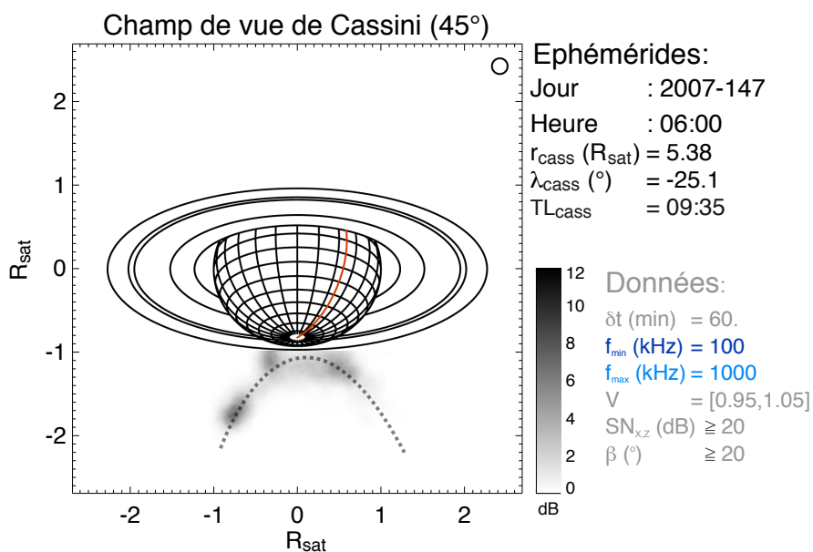
FIG. 6.8: Image radio dans le plan de Cassini le 27 mai 2007 de TL = 06:00 à TL = 07:00. La distribution des sources au sud suit la forme caractéristique d'une cloche (en tiretés gris). Le méridien rouge indique midi (TL = 12:00). Lorsqu'une source radio (c'est-à-dire une ligne de champ active) balaie le méridien occupé par Cassini, l'émission observée évolue le long de la courbe en pointillés. Sa traduction dans le plan temps-fréquence est un arc.
