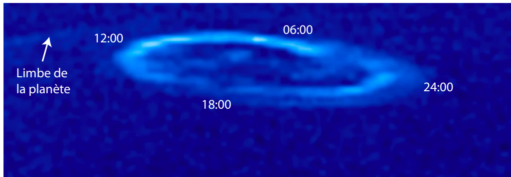
FIG. 4.14: Image de l'ovale nord UV (situé sur la face nuit) prise par le spectro-imageur de Cassini UVIS le 25 mai 2007. La position de Cassini correspondait alors à \lambda_{cass} \sim 26^\circ , TL_{cass} \sim 18:30 et r_{cass} \sim 18 R_{sat} . On distingue une forme double de l'ovale côté minuit.
