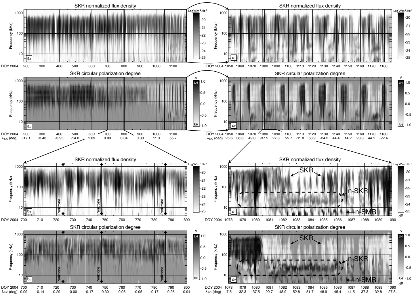
FIG. 2.4: Spectres dynamiques (distributions temps-fréquence), de la densité de flux S normalisée à 1 UA (indice 1) et du taux de polarisation circulaire V (indice 2) observés entre 3.5 et 1500 kHz. (a) correspond à la période du 29 juin 2004 au 31 mars 2007. Le spectre a_2 montre que la polarisation dominante (noire pour la polarisation LH, blanche pour la polarisation RH) varie avec la latitude de Cassini. La polarisation gauche est observée préférentiellement lorsque Cassini est située dans l'hémisphère sud. (b) présente un zoom du panneau (a) correspondant à des orbites quasi-équatoriales. La polarisation gauche domine le spectre sous 600 kHz. (c) trace un zoom du panneau (a) correspondant à des excursions de haute latitude. Les deux composantes polarisées sont observées de façon alternée, suivant la variation de \lambda_{\text{cass}} . Enfin, (d) présente un zoom de (c) où l'on distingue, en sus du SKR à large bande, des émissions basse fréquence à bande étroite pour f \leq 40 kHz.
