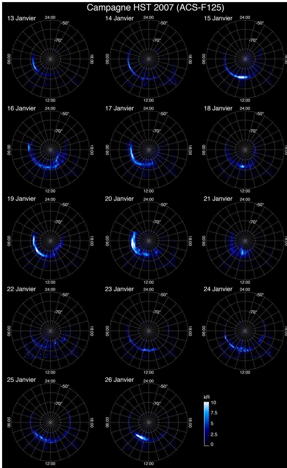
FIG. 4.7: Idem figure 4.5 avec une observation en projection polaire et correction de l'angle de phase \gamma (voir annexe C). Sur la majorité des images, les anses de l'ovale sont situées à TL = 06:00 et 18:00.
