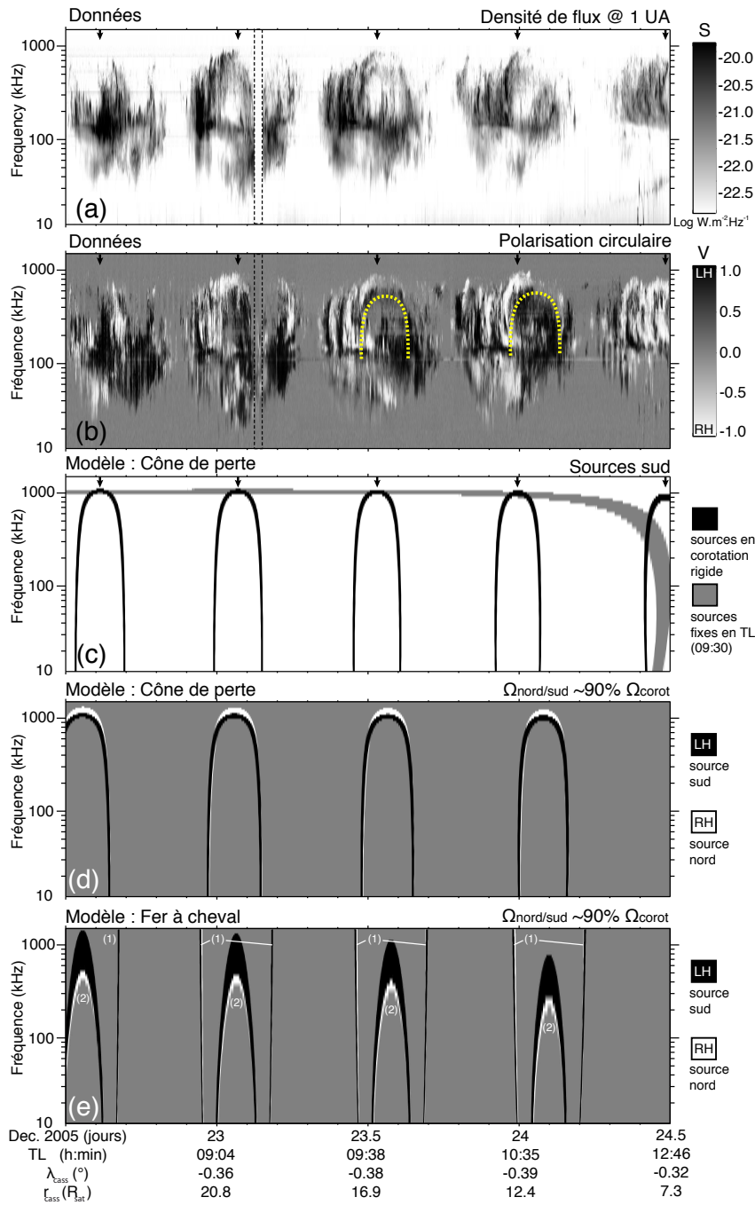
FIG. 6.1: Spectres dynamiques du SKR observés et simulés sur une durée de 2 jours de l'année 2005. Les panneaux (a) et (b) indiquent conventionnellement la densité de flux S normalisée à 1 UA et le taux de polarisation circulaire normalisé V . Les flèches noires indiquent la période radio (correspondant à chaque occurrence de SKR). Les pointillés jaunes indiquent les arcs "doubles" observés. Le panneau (c) montre le résultat de simulation de deux sources sud. Chacune est constituée de points source répartis le long de la ligne de champ entre 10 et 1200 kHz pour une latitude du pied de la ligne de champ \lambda_B = -70^{\circ} . L'angle d'ouverture \theta(f) associé à chaque point source de fréquence f est calculé sur la base de l'instabilité "cône de perte". L'émission représentée en gris est fixée à TL = 09:30 tandis que l'émission en noir est en sous-corotation avec la planète (l'observateur la voit donc passer autant de fois que la planète a fait de tours sur elle même). Le panneau (d) représente le résultat de la simulation "cône de perte" de deux sources conjuguées nord/sud qui sont entraînées en sous-corotation à 90% de la période radio (proche de la période de rotation planétaire, voir chapitre 3). Comme pour le panneau (b), les émissions sud sont représentées en noir et les émissions nord en blanc. Enfin, le panneau (e) montre le résultat de simulation de deux sources conjuguées nord/sud obtenu dans l'hypothèse "fer à cheval" pour deux angles d'ouverture constants différents : l'indice (1) indique \theta(f) = 90^{\circ} tandis que l'indice (2) correspond à \theta(f) = 55^{\circ} .
