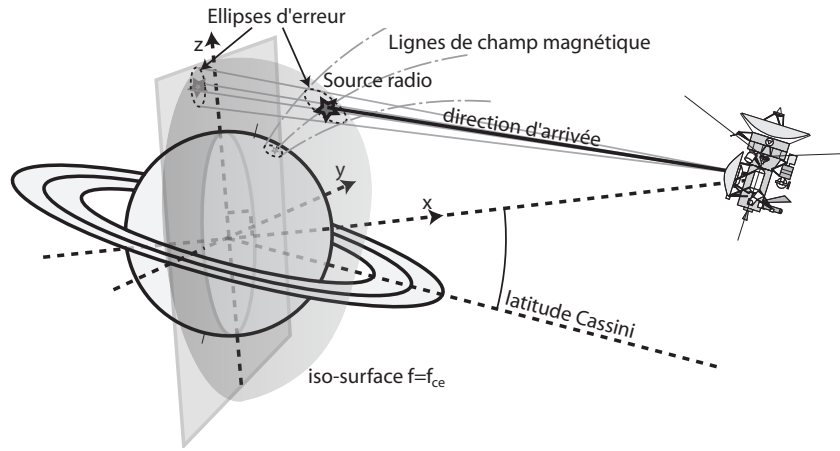
FIG. E.1: Figure tirée de [Ceconi et al., 2008] illustrant le principe de l'imagerie radio par goniopolarimétrie. Cassini observe une source radio (représentée par une étoile) avec une direction d'arrivée indiquée par la ligne en trait plein. L'intersection de cette ligne avec le plan d'observation ( y, z ) donne la position projetée de la source à deux dimensions. La connaissance du champ magnétique, et par extension de la gyrofréquence en tout point permet de calculer l'iso-surface f = f_{ce} dont l'intersection avec la direction d'arrivée donne la position de la source dans l'espace et permet d'identifier la ligne de champ magnétique associée ainsi que les coordonnées de son "pied" (footprint) à la surface de la planète. Les ellipses en tiretés indiquent l'incertitude sur la direction d'arrivée.
