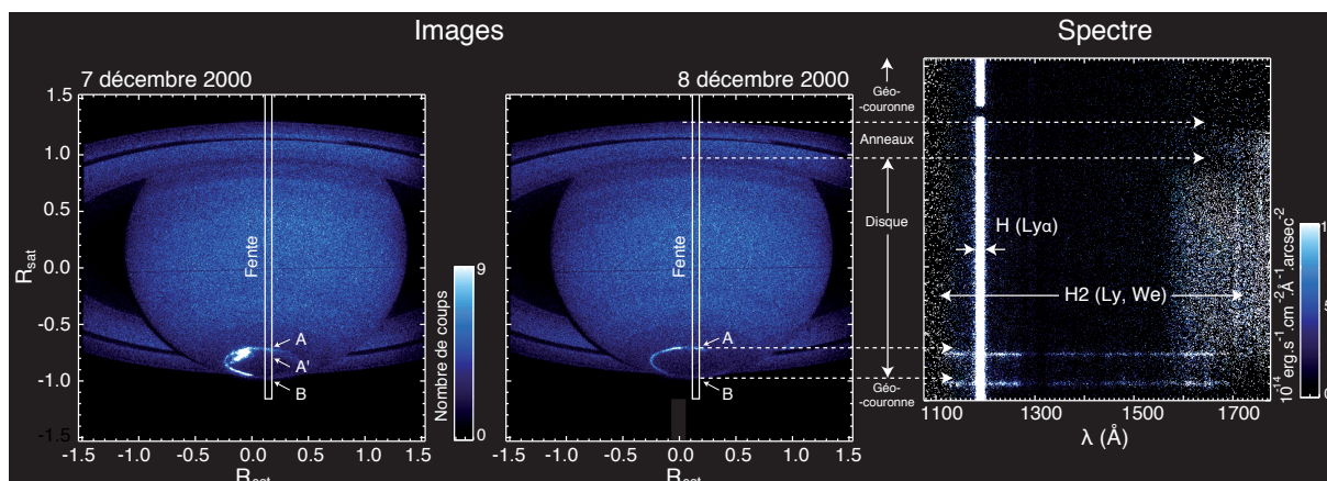
FIG. 4.9: Images des 7 et 8 décembre 2000 et spectre mesuré le 8 décembre 14 min après l'image prise le même jour (voir tableau 4.2). Un embrillancement est visible le 7 décembre, mais il a disparu le jour suivant. La dimension spatiale y du spectre (le long de la fente) a été ajustée à l'image (par le rapport des résolutions angulaires et un ajustement spatial sur la trace des ovales) et les correspondances importantes sont indiquées par les flèches en tiretés. Les composantes A et B désignent les parties de l'ovale interceptées par la fente du spectromètre côté disque et côté limbe respectivement. La composante A' (vue dans les spectres du 7 décembre) pourrait correspondre à l'embrillancement observé sur l'image ayant tourné avec la planète. Le spectre montre que la raie Ly \alpha à 1217 Å est observée partout (sauf dans l'extinction vers le haut du spectre 2D qui correspond à un masque servant à définir le bruit de fond lié au HST). Les raies de H 2 sont visibles sur le disque. Les émissions aurorales montrent une intensification du spectre par rapport au disque.
