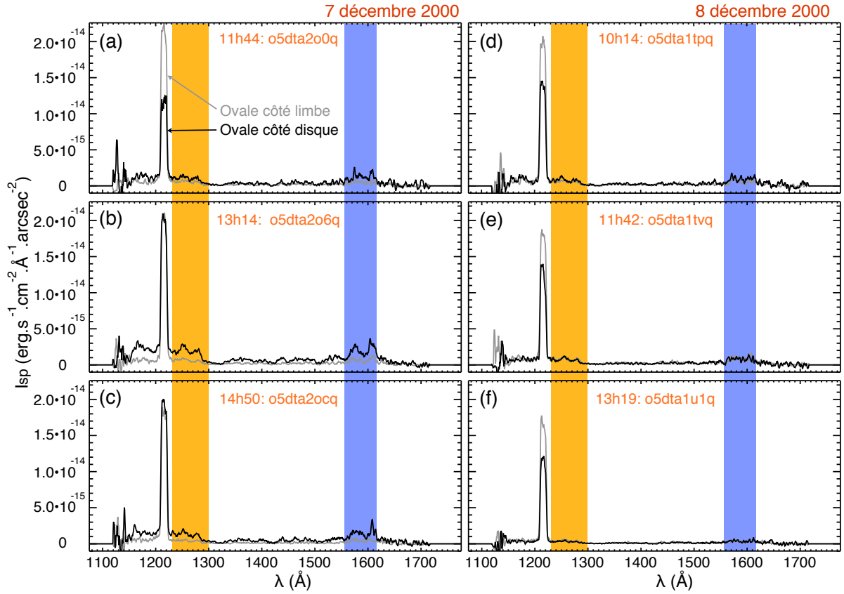
FIG. 4.11: Spectres de l'émission I_{sp} de l'ovale côté disque (en noir) et de l'ovale côté limbe (en gris) issus des six spectres 2D initiaux de la campagne d'observation de 2000 (voir tableau 4.2). Chaque spectre est en réalité un spectre moyen (calculé avec l'équation D.1, voir annexe D), lissé sur 5 valeurs consécutives. Les zones orange et violette indiquent les domaines de longueurs d'onde utilisés pour calculer les rapports de couleur et correspondant respectivement l'émission absorbée et l'émission non absorbée.
