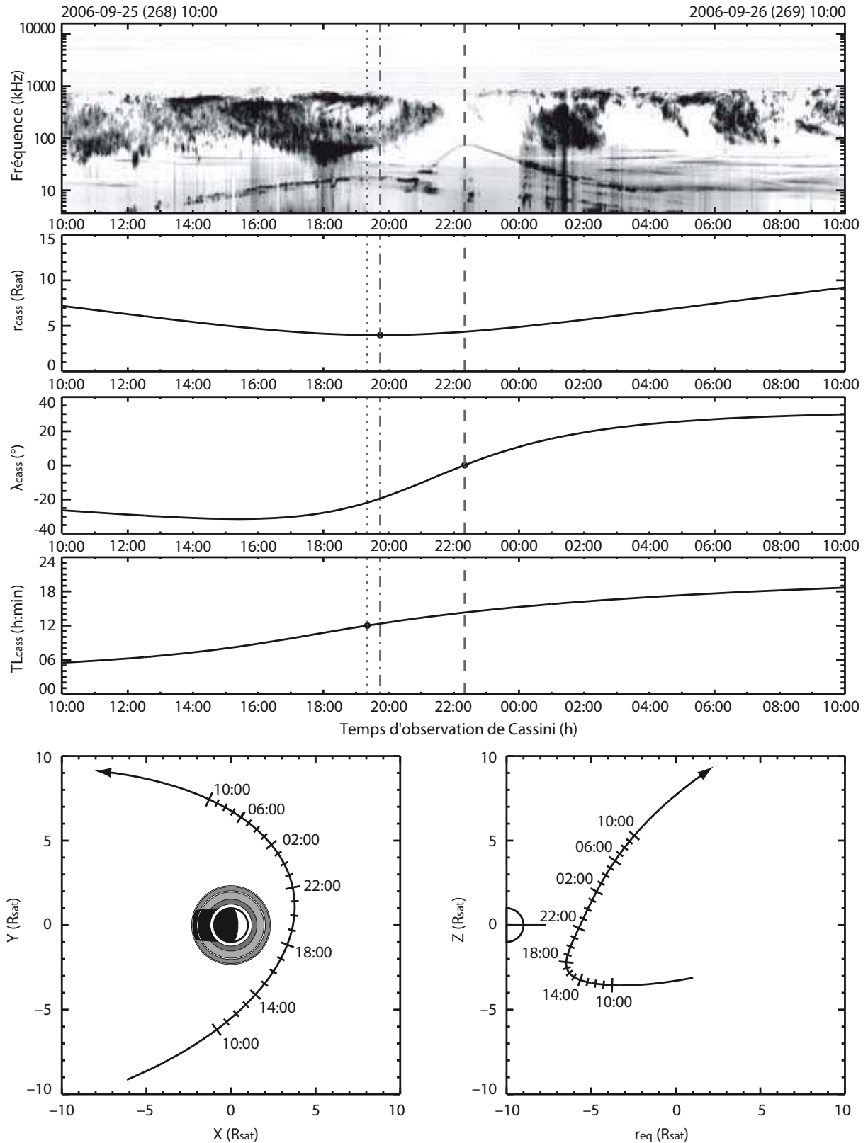
FIG. 5.1: Spectre dynamique du flux radio reçu (un fond a été retiré pour chaque fréquence) et éphémérides de la sonde Cassini pendant son passage au périkrone de l'orbite 29. Les lignes verticales indiquent le passage à TL_{cass} = 12:00 (pointillés), la traversée du plan équatorial (tiretés) et la position de Cassini la plus proche de Saturne (pointiretillés). Le SKR disparaît lorsque Cassini entre dans la zone d'ombre équatoriale autour du temps d'observation 22 h.
