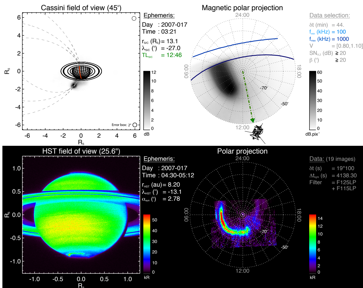
FIG. 5.7: Idem figure 5.6 à l'exception de la durée d'intégration des images, qui correspond ici à l'intégralité des prises de vue HST de la journée du 17 janvier 2007 (19 poses de 100 s chacune).
