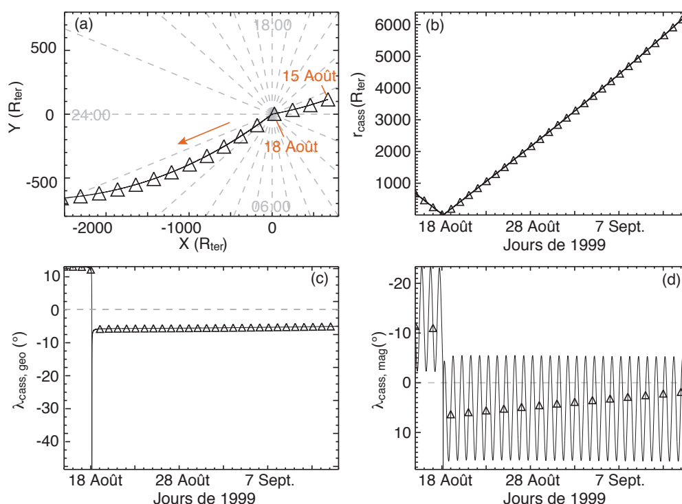
FIG. 3.7: Ephémérides de la sonde Cassini entre le 15 août et le 14 septembre 2004 lors du survol de la Terre. Sur chaque graphe, les triangles indiquent les jours à minuit. Le panneau (a) donne une vue de la trajectoire de la sonde dans le plan de l'écliptique. La flèche orange indique le sens de sa trajectoire. Les coordonnées X et Y correspondent au repère équatorial Terre-soleil : l'axe X pointe de la planète vers le soleil, l'axe Z est aligné avec l'axe de rotation planétaire et l'axe Y complète le trièdre direct. R_{ter} = 6400 km indique le rayon terrestre. Les temps locaux sont indiqués par les tirets gris et les mentions 06:00, 08:00 et 24:00 (la direction du soleil à 12:00 n'a pas été mentionnée par souci de clarté). La sonde passe au plus près de la Terre le 18 août puis passe la majorité des observations côté nuit entre 01:00 et 02:00 en temps local. Le panneau (b) donne la distance r_{cass} de Cassini à la Terre. La vitesse de la sonde atteint \sim 9 R_{ter} par heure. Le panneau (c) trace la latitude géocentrique. Comme la sonde est dans le plan de l'écliptique \lambda_{cass, geo} passe de \sim 12^\circ à \sim -6^\circ lors du passage du côté jour au côté nuit. Le panneau (d) trace la latitude magnétique de Cassini. Le dipôle magnétique étant incliné sur l'axe de rotation de \sim 10.5^\circ , \lambda_{cass, mag} oscille quotidiennement sur la gamme [-2, -23^\circ] avant le 18 août et sur [5, 16^\circ] après.
