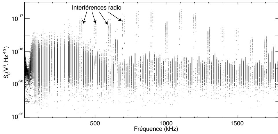
FIG. A.6: Flux S_G ( V^2.Hz^{-1} ) en fonction de la fréquence pour le jour 115 de l'année 2004. Les parasites se traduisent sous la forme de valeurs de flux plus intenses que la normale sur les canaux de fréquence au voisinage des harmoniques de 100 kHz. La largeur typique de ces parasites est en général de 2 à 3 canaux.
