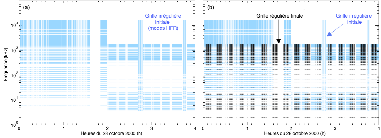
FIG. A.5: (a) Exemple de la distribution temps-fréquence hétérogène des différents modes du HFR utilisés le 28 octobre 2000 entre minuit et 4 h. (b) Superposition de la distribution temps-fréquence homogène (définie à la partie A.4) pour intégrer les données (en noir).
