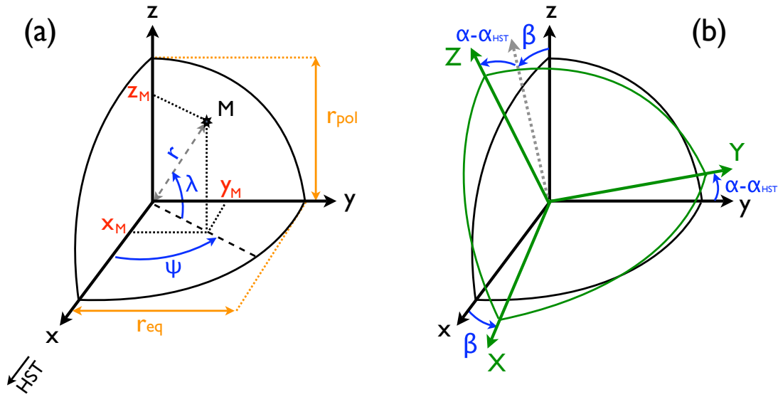
FIG. C.1: (a) Coordonnées de l'ellipsoïde dans le repère constitué par ses axes principaux (x,y,z) . x_M , y_M et z_M indiquent les coordonnées cartésiennes du point M et r , \psi et \lambda ses coordonnées sphériques (respectivement la distance, la longitude et la latitude planétocentrique de M ). r_{eq} et r_{pol} indiquent les rayons équatorial et polaire. (b) Changement de repère de (x,y,z) vers (X,Y,Z) , correspondant au repère (-V_1,-V_2,V_3) lié au HST, par une rotation de \beta autour de l'axe y et \alpha-\alpha_{HST} autour de l'axe x .
