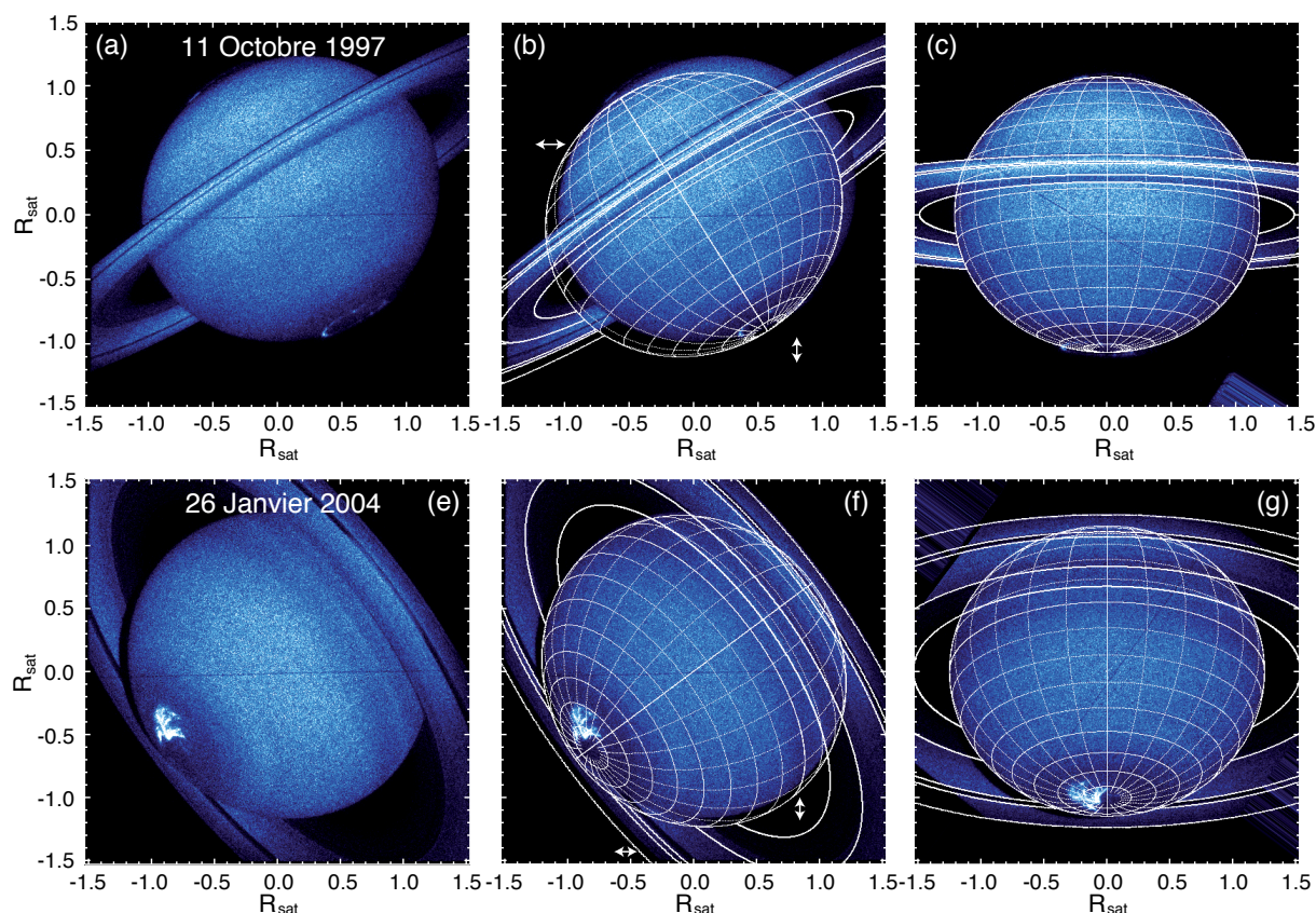
FIG. C.2: (a) Image HST-STIS prise avec le filtre SRF2 le 11 octobre 1997 dans le repère du HST. (b) Même image avec sa grille de coordonnées sphériques nominale construite à l'aide de la position et des paramètres physiques de Saturne. Les parallèles sont tracés tous les 10 degrés et les méridiens tous les 15 degrés ( i.e. 01:00 de temps local) (c) Image et sa grille dans le repère lié à l'axe de rotation \Omega de Saturne après correction des dérives de pointage du HST (-34 et -42 pixels [soit -0.83 et -1.03 arcsec] en translation et 0.15^\circ en rotation) et ajustement de sa résolution angulaire ( 0.0245 \text{ arcsec.pix}^{-1} ). (c,d,e) Idem avec une image HST-STIS-SRF2 prise le 26 janvier 2004. Les corrections appliquées à l'image correspondent à des valeurs de -2 et -16 pixels en translation, 0.3^\circ en rotation et une résolution angulaire de 0.0244 \text{ arcsec.pix}^{-1} .
