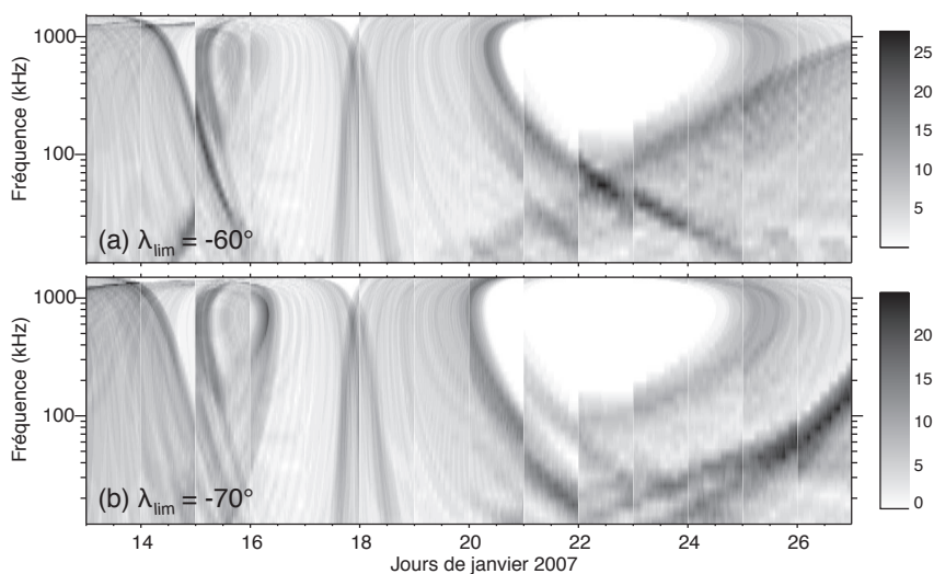
FIGURE 6.10 – Spectres dynamiques des émissions radio simulées par le modèle "cône de perte" entre le 13 et le 26 janvier 2007. L'angle d'ouverture est calculé pour une vitesse v_{e^-} = 0.2 c et la position des sources radio est celle d'un ovale typique UV quotidien utilisant une altitude de projection de 1000 km. La partie manquante des ovales UV a été extrapolée côté nuit à la valeur \lambda_{B, lim} = -60^\circ (panneau (a)) et \lambda_{B, lim} = -70^\circ (panneau (b)) au temps local TL_B = 24:00 . Ces deux valeurs encadrent la valeur \lambda_{B, lim} = -65^\circ , utilisée pour tracer les figures 6.7b et 6.9a
