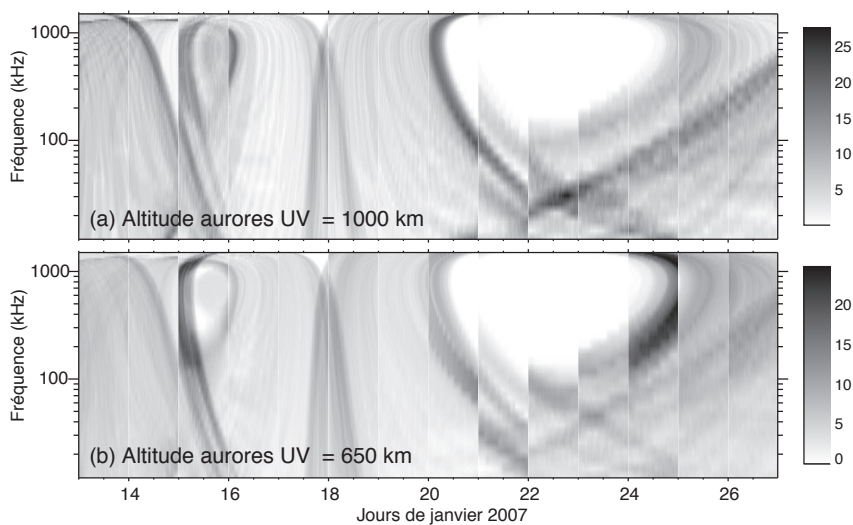
FIGURE 6.9 – Spectres dynamiques des émissions radio simulées par le modèle "cône de perte" entre le 13 et le 26 janvier 2007. L'angle d'ouverture est calculé pour une vitesse v_{e^-} = 0.2 c et la position des sources radio est celle d'un ovale typique UV quotidien dont la partie manquante a été extrapolée côté nuit à \lambda_{B, lim} = -65^\circ pour TL_B = 24:00 . Pour le panneau (a) (identique au panneau (b) de la figure 6.7), la projection des ovales UV quotidiens ainsi que la grandeur \omega_{ce,max} utilisée dans l'équation 6.6 ont été calculées pour une altitude des aurores fixée à 1000 km. Pour le panneau (b), l'altitude des aurores utilisée est 650 km.
