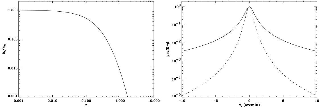
FIG. 3.5 – (a) Rapport normalisé de la brillance X à la brillance SZ en fonction du redshift pour un amas de 10 keV. (b) Profil d’amas en X (ligne pointillée) et en SZ (ligne pleine) pour un amas de 10 keV, avec \beta = 2/3 , r_c = 0.3 h_{50}^{-1}(q_0 = 0.5) Mpc, situé à z = 1 .
