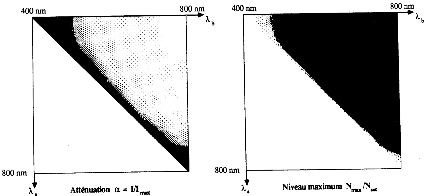
FIGURE II.2 : Résultats obtenus pour des filtres portes dans le cas d'un échantillon \text{SiO}_2 5500 Å sur Si.
