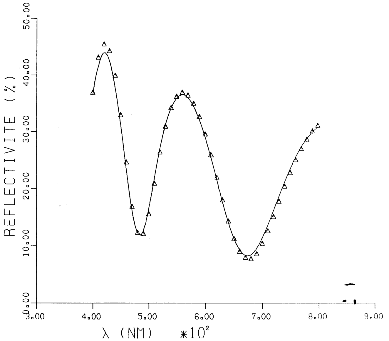
Figure III.2 : Spectre de réflectivité en ondes planes d'un échantillon \text{SiO}_2 5800 Å sur Silicium. ( \Delta Expérimental ; — théorique).
