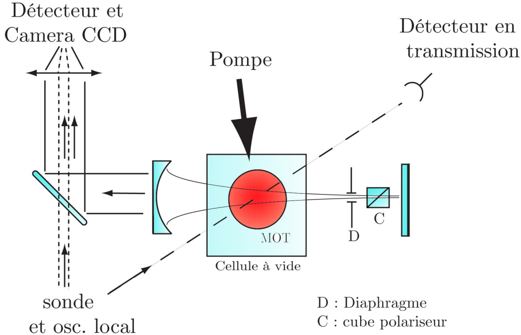
FIG. 4.8 – Cavité laser et détection. L'angle d'incidence des pompes par rapport à la cavité vaut environ 20 degrés. Une sonde nous sert à effectuer des battements avec le laser pour déterminer sa fréquence.
