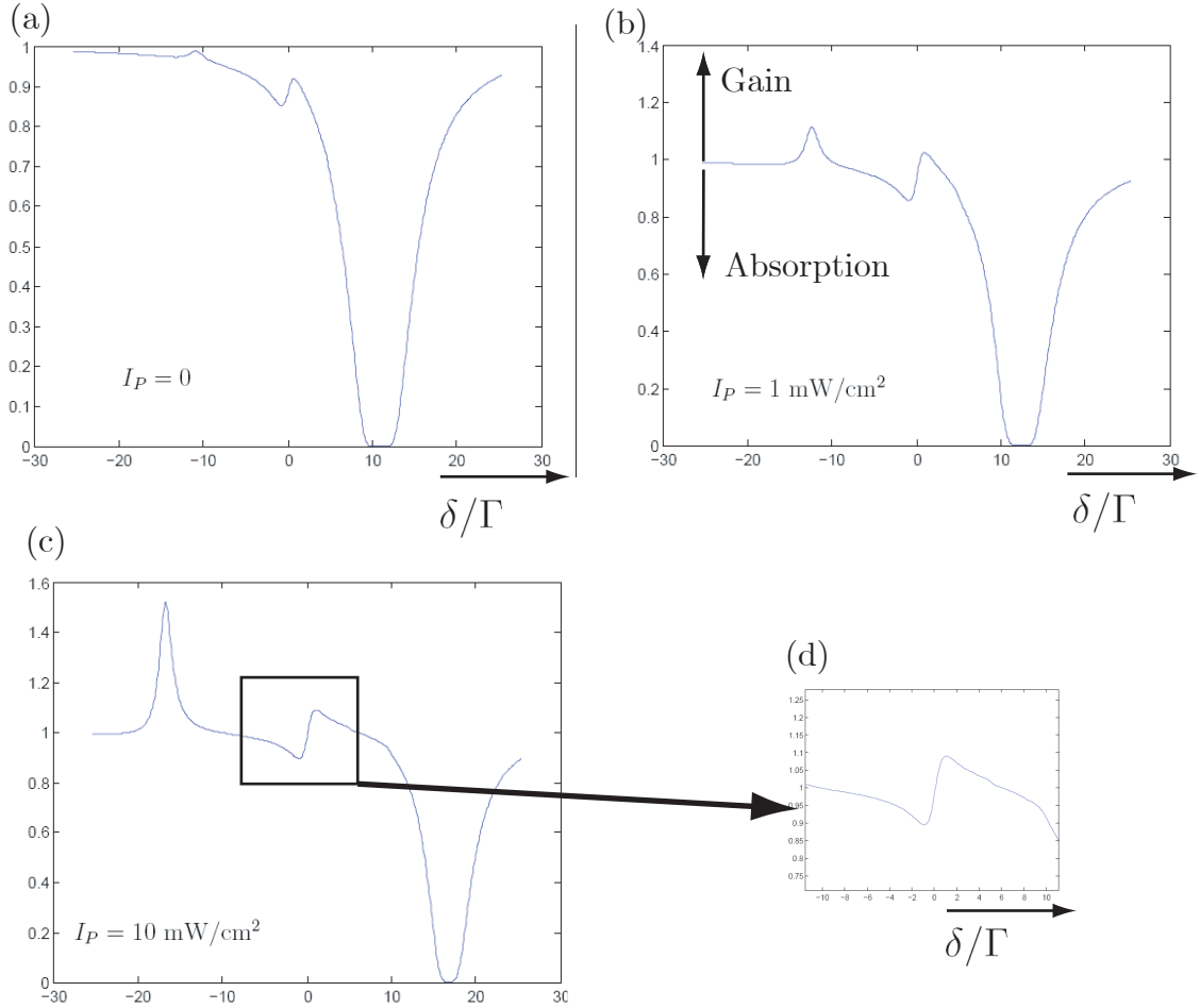
FIG. 3.6 – Spectre de transmission normalisé du faisceau sonde à travers un nuage d'atomes d'épaisseur optique à résonance b_0 = 20 , avec pompe décalée de la résonance atomique \Delta = -10 MHz. (a) pompe d'intensité faible, (b) et (c) est augmentant l'intensité pompe. (d) est un zoom de (c) autour \delta = 0 , on observe une structure dispersive présentant également du gain.
