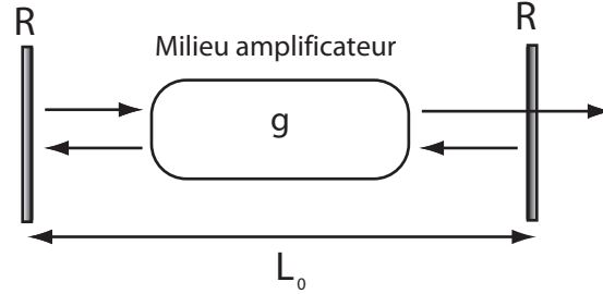
FIG. 3.1 – Cavity d'amplification linéaire. Les miroirs ont un coefficient de réflexion de valeur R et la cavity est de longueur L_0 .
