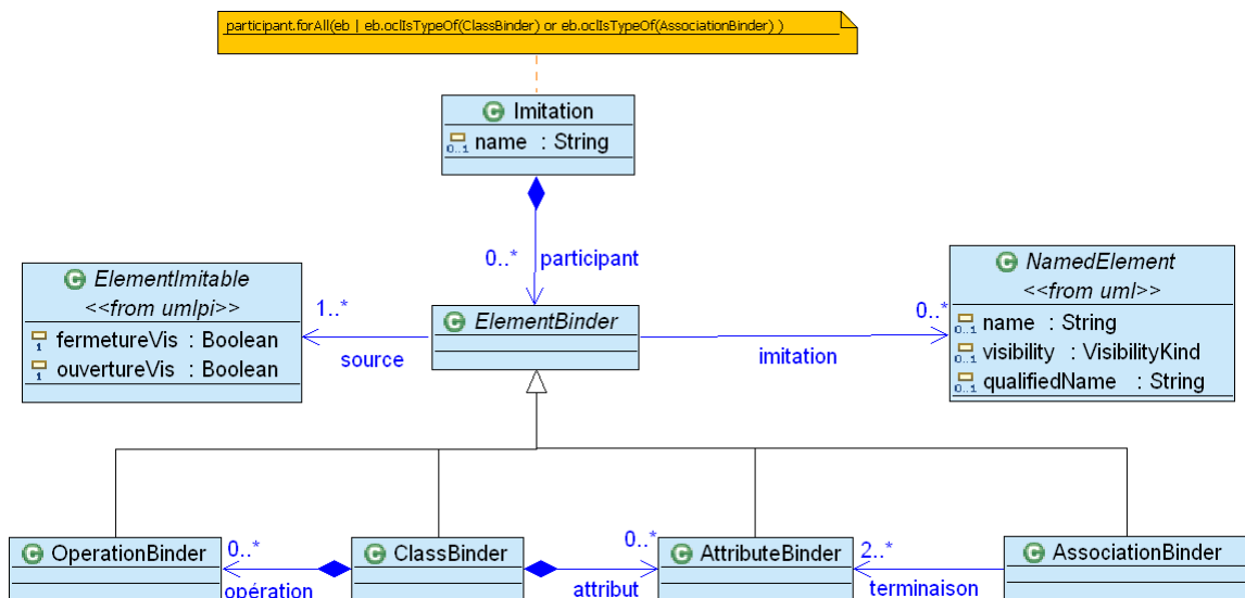
Figure 4.11 : Méta-modèle UML \pi iBind .
