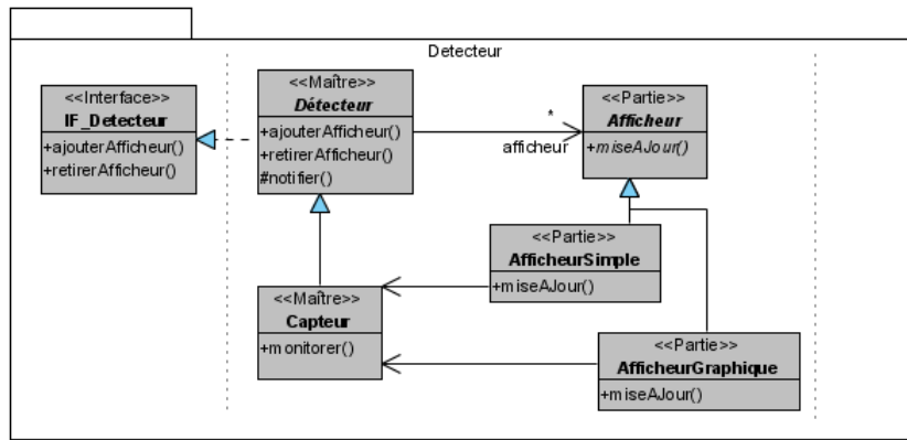
Figure 5.3 : Encapsulation d'une imitation du patron « Observateur » : le composant Detecteur .
