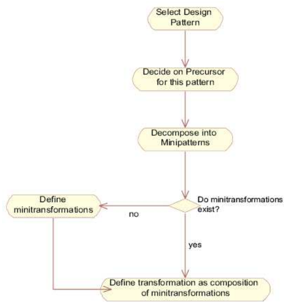
Figure 2.5 : Processus d'imitation proposé par (O`Kinneide, 2001)
