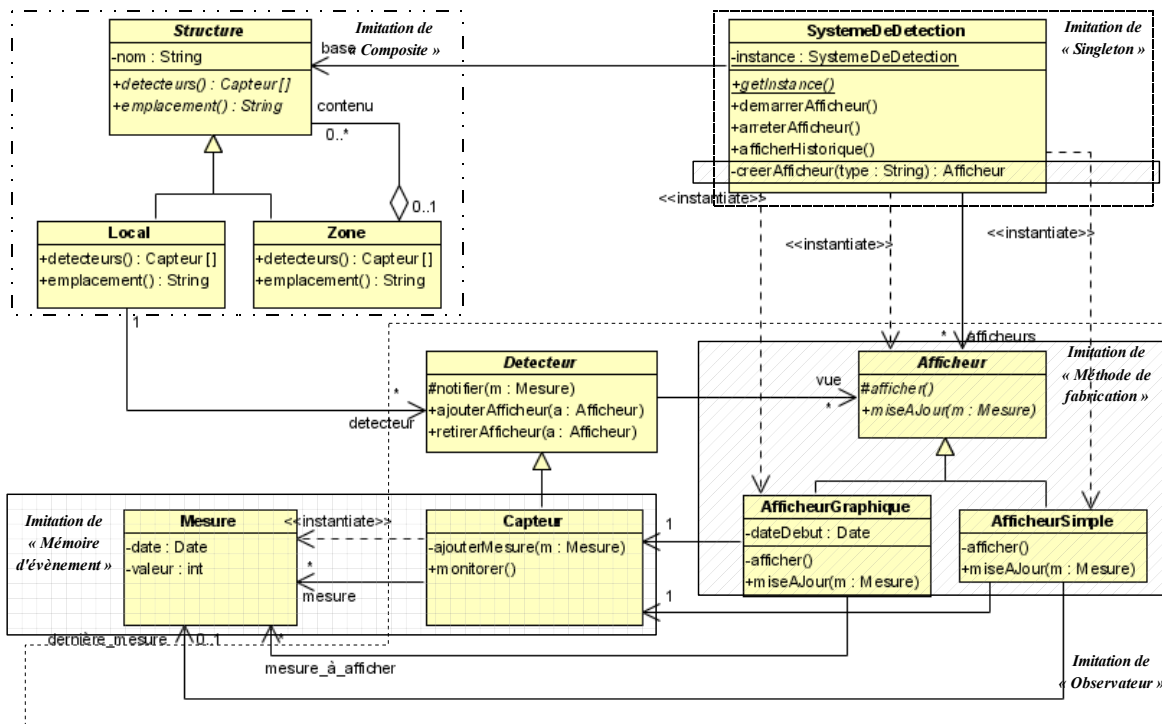
Figure 4.7 : Récapitulatif des patrons imités (tiré du cas d'étude)
