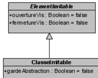
Figure 3.23 : Nouvelles propriétés génériques : abstraction et visibilité.
