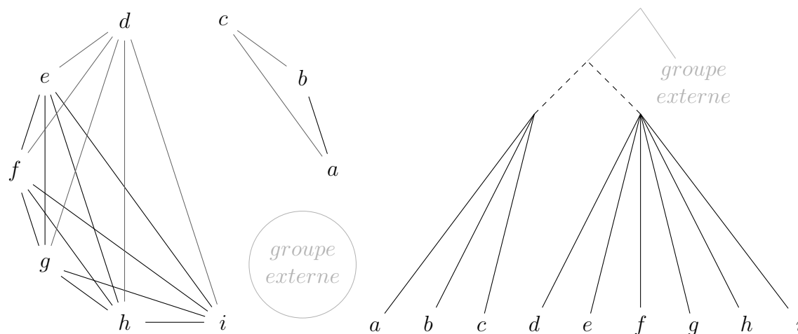
Figure 4.3. Déroulement de l'algorithme OneTree (suite). On s'intéresse ici uniquement aux taxons a à i , qui formaient une des composantes connexes du graphe de l'étape précédente. Le groupe extérieur n'est plus pris en compte (d'où la couleur grise choisie ici). Le triplet (ae|\text{groupe externe}) était le seul à soutenir l'arête a - e ; cette arête n'est donc plus présente dans le graphe. Les deux composantes connexes obtenues sont constituées des ensembles de taxons a à c et d à i . Le sous-arbre des taxons a à i peut donc être décomposé en deux sous-arbres.
