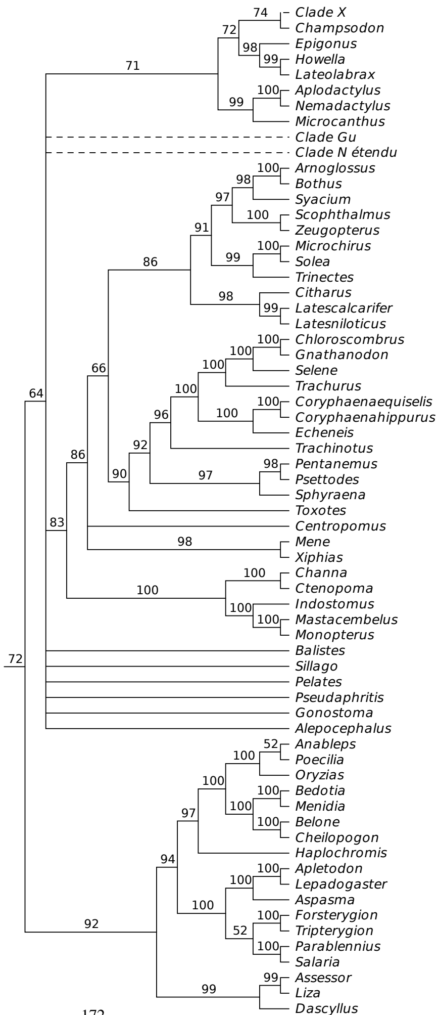
Figure 8.7. Arbre de synthèse construit par la méthode dérivée du MRP (suite). Suite page suivante (clades N étendu et Gu) et page 174 (clade X).
