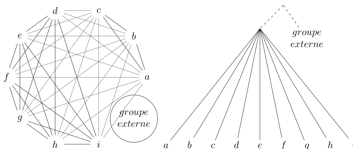
Figure 4.2. Déroulement de l'algorithme OneTree. Application aux triplets de l'arbre de la figure 4.1. Étape initiale. Chaque sommet du graphe de gauche représente un taxon. Il y a une arête entre deux sommets quand il existe un triplet dans lequel la partie interne est constituée des deux taxons correspondant, c'est-à-dire quand ces taxons forment une paire incluse. L'arête a - b , qui correspond à la paire incluse \{ab\} , est soutenue entre autres par les triplets (ab|c) et (ab|\text{groupe externe}) . À ce stade, seul le groupe extérieur n'est dans aucune paire incluse. Les taxons a à i forment une composante connexe du graphe ; ils constituent un sous-arbre de l'arbre en cours de construction (le groupe externe constitue un autre sous-arbre).
