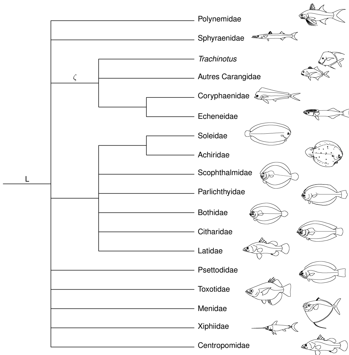
Figure 9.5. Résumé de la topologie du clade L.
