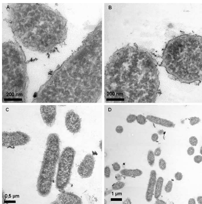
Photo 16 Différentes vues d'un échantillon observé en MET de E. coli ayant incubées 3h dans l'eau ultrapure avec 240 ppm de \text{CeO}_2 nanoparticulaires.
