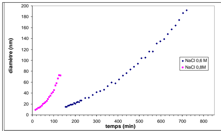
Figure 62 Comparaison de l'évolution du diamètre des nanoparticules de \text{CeO}_2 (12 g/L) pour deux concentrations en sel (0,6 M et 0,8 M de NaCl) en fonction du temps.
