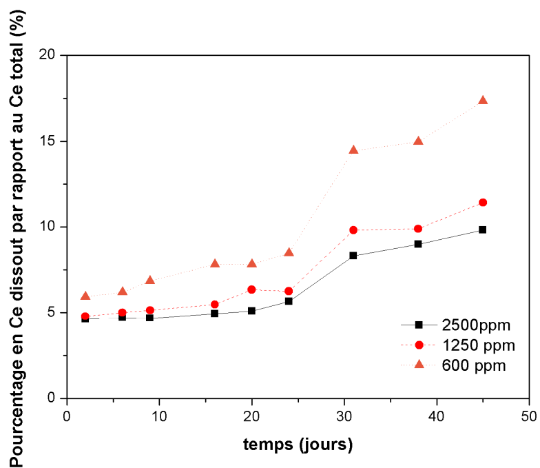
Figure 20 Cinétique de dissolution de trois suspensions de nanoparticules de concentrations : 2,5 ; 1,25 et 0,6 g/L de CeO 2 . Concentration en pourcentage de cérium dissous par rapport au cérium total au cours du temps.
