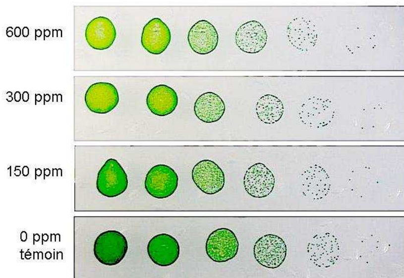
Photo 31 Test en gouttes réalisé sur des cellules de Synechocystis incubées pendant 3 h avec des nanoparticules de \text{CeO}_2 -PAA dans l'eau ultrapure avant dépôt sur milieu solide. Première goutte non diluée puis dilutions successives de 10 en 10.
