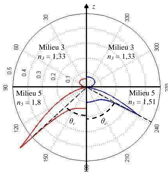
Figure 3.12. Diagramme d'émission d'un ensemble de dipôle orientés de façon isotrope et situés à une altitude de 10 nm par rapport à une lame de verre d'indice de réfraction 1,8 (en rouge) et 1,51 (en bleu). On a également reporté les deux droites qui matérialisent les angles limites de réflexion totale \theta_c entre les milieux 3 et 5 et qui séparent l'émission sous-critique (pour des angles inférieur à \theta_c ) de l'émission sur-critique (pour des angles supérieur à \theta_c ).
