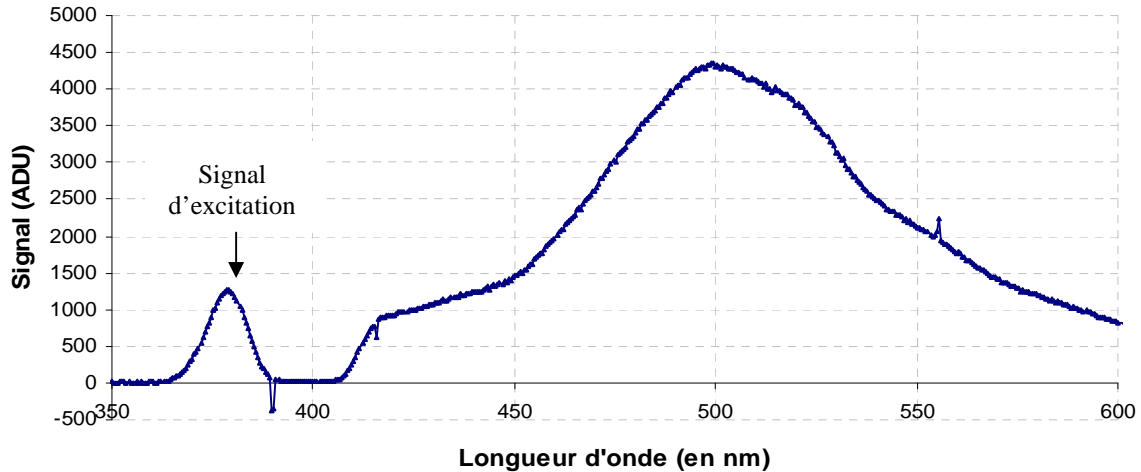
Figure 3.37. Spectre d'une couche de TiO 2 dopée à l'aide d'un fluorophore organique, la Coumarine 500. Ce spectre a été obtenu en excitant la couche émettrice à l'aide d'une diode UV centrée sur 470 nm. Un ADU (Analog to Digital Unit) représente 1 pas de la conversion du signal analogique en signal numérique par la caméra CCD du spectrographe.
