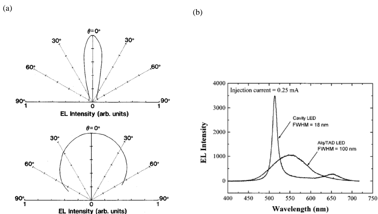
Figure 2.21. Illustration des effets d'une cavité de type Fabry Péroต์ sur le diagramme d'émission et le spectre d'émission d'une OLE. (a) : diagramme d'émission d'une OLED située au non dans une cavité (d'après Tsutsui 1994). (b) : spectre d'émission d'une OLED avec ou sans cavité (d'après Dodabalapur 1996)
