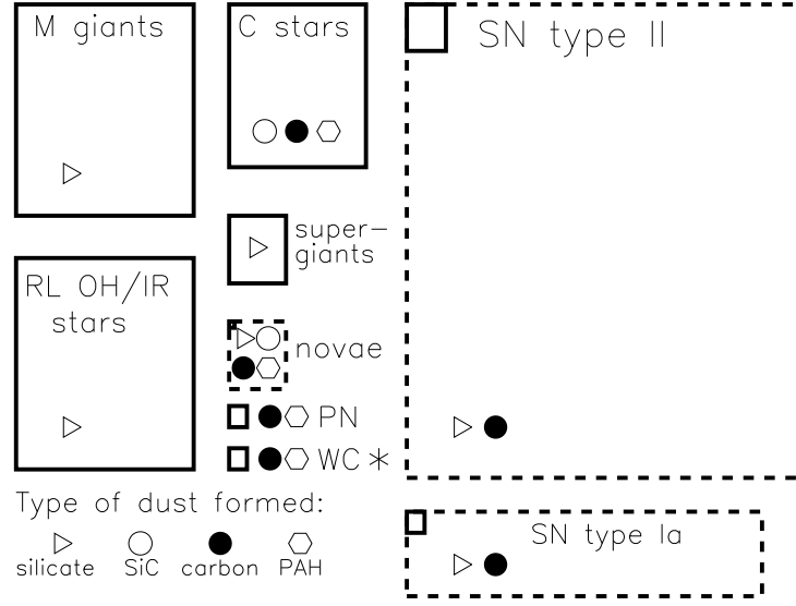
FIGURE 1.15 – Contributions relatives (en surface) des différents sites de formation des poussières, hors formation dans le milieu interstellaire. C stars : étoiles à carbone, PN : nébuleuse planétaire, WC : Wolf-Rayet Carbon rich star, RL OH/IR : étoiles en fin de vie caractérisées par une émission IR et à 18 cm caractéristiques des radicaux hydroxyyles OH. Les pointillés indiquent une limite supérieure. Extrait de Jones et al. (1997) .
