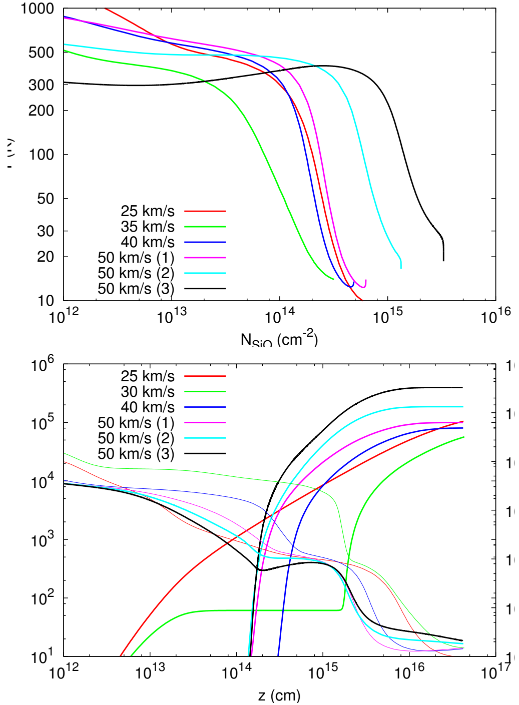
FIGURE 9.12 – Densité de colonne de SiO produite dans le choc, en fonction ( Haut ) de la température du gaz ou ( Bas ) de la position dans le choc avec le profil de température correspondant. Les codes de couleur sont identiques sur les deux figures. Pour le choc de 50 \text{ km s}^{-1} , 3 modèles sont présentés : (1) Modèle d'érosion de May et al. (2000) et Barlow (1978) sans piégeage dans le front de choc, (2) idem avec le modèle d'érosion de Tielens et al. (1994) , et (3) Destruction des poussières dans le front de choc (érosion des petits grains piégés) suivi d'une destruction dans le choc (vaporisation des gros grains).
