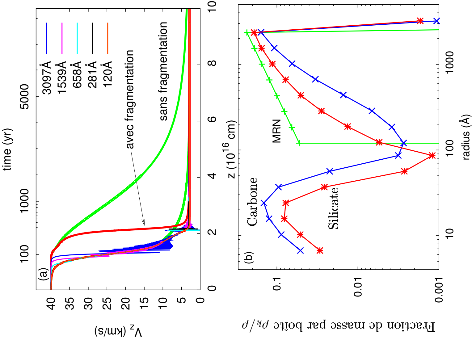
FIGURE 11.8 – (a) Profil de vitesse dans la direction de propagation du choc dans un choc C de 40 \text{ km s}^{-1} se propageant dans un nuage de densité initiale n_H = 10^4 \text{ cm}^{-3} . (b) Distribution en taille des poussières silicatées et carbonées au sortir du choc. La densité de masse par boîte \rho_k est rapportée à la densité de masse totale des poussières silicatées dans le milieu pré-choc.
