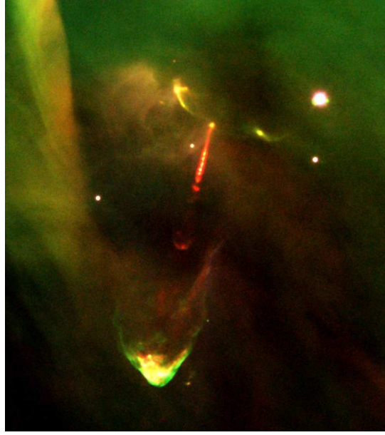
FIGURE 2.19 – Choc d'étrave HH34 avec son jet (Nébuleuse d'Orion, à \sim 500 pc).
