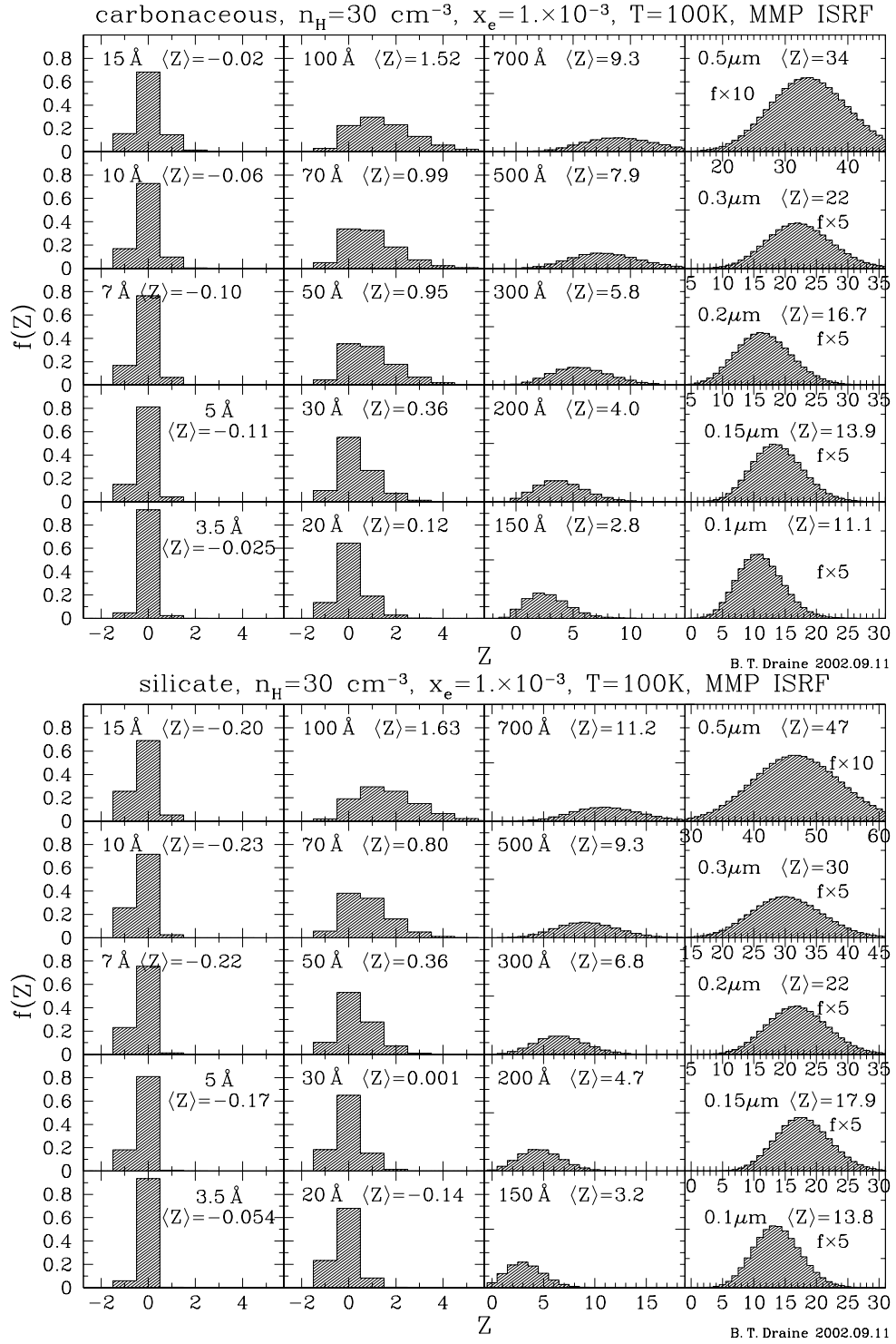
FIGURE 5.13 – Charge distribution functions for carbonaceous grains and silicate grains in "cold neutral medium" diffuse HI. Reproduction de la figure (30) de Draine (2002) pour comparaison avec la figure 5.12.
