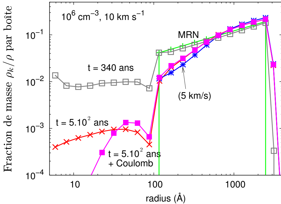
FIGURE 10.7 – Distribution en taille des poussières silicatées avant (MRN), à la fin de la phase de fragmentation des poussières ( t = 340 ans) et après le passage du choc ( t = 10^4 ans) pour un choc de 10 \text{ km s}^{-1} se propageant dans un nuage de densité initiale n_{\text{H}} = 10^6 \text{ cm}^{-3} . On observe une nette accélération de la coagulation par attraction coulombienne entre petits grains chargés négativement et gros grains positifs. La distribution finale des grains silicatés du choc de 5 \text{ km s}^{-1} de la figure 10.4 est indiquée comme point de comparaison.
