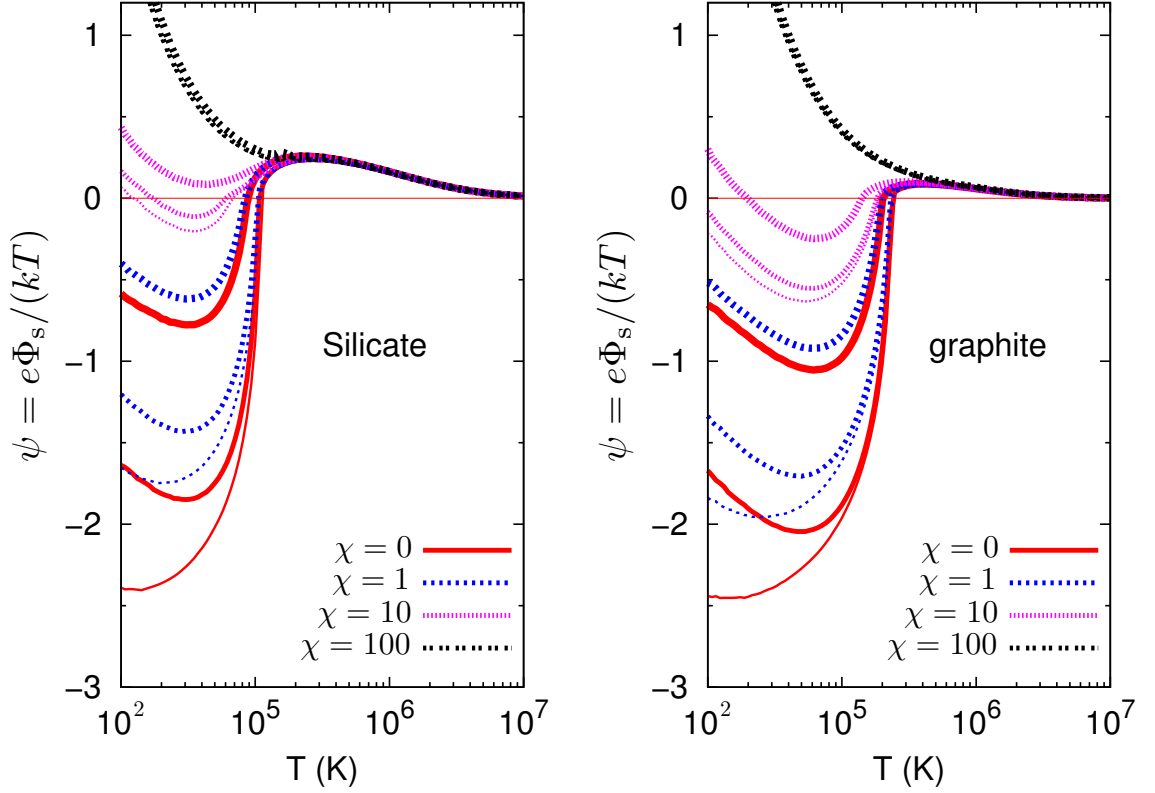
FIGURE 5.14 – Le rapport \psi de l'énergie potentielle électrique e\Phi_s du grain à l'énergie thermique kT du plasma pour des grains silicatés et carbonés, en fonction de la température d'un plasma totalement ionisé et pour différentes valeurs de l'intensité \chi du champ de rayonnement (relativement au champ ISRF de Mezger et al. (1982) ) et de la vitesse \Delta V du grain relativement au plasma (fin : 31.6 km/s, épais : 100 km/s, très épais : 316 km/s). Le décalage entre les courbes des grains carbonés et celles des grains silicatés provient du modèle d'émission secondaire des électrons, propre à chaque matériau ( cf. Table 5.1). Ces graphes reproduisent de manière très satisfaisante la figure 6 de McKee et al. (1987) .
