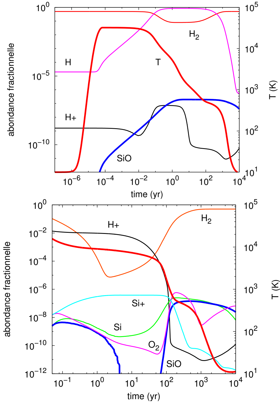
FIGURE 9.9 – Profil de l’abondance de SiO dans deux chocs de 25 \text{ km s}^{-1} ( Haut ) et 35 \text{ km s}^{-1} ( Bas ) Dans le choc de 25 \text{ km s}^{-1} , l’érosion est négligeable et le SiO produit par vaporisation n’est pas dissocié alors que \text{H}_2 l’est (l’énergie de liaison de SiO \sim 8 \text{ eV} est supérieure à celle du dihydrogène \sim 4 \text{ eV} ). Dans le choc de 35 \text{ km s}^{-1} , le SiO produit par vaporisation est rapidement dissocié, puis reformé par réaction en phase gazeuse entre Si et \text{O}_2 . L’abondance de SiO en phase gazeuse diminue dans le post-choc car il est adsorbé à la surface des grains.
