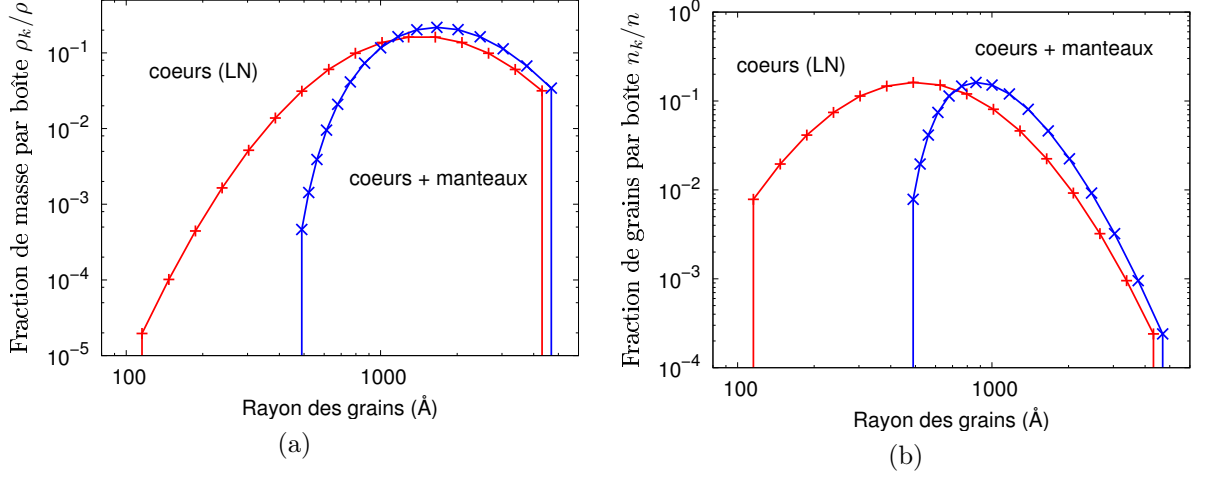
FIGURE 4.4 – Même chose que la figure 4.2 mais pour une distribution log-normale des coeurs ( a_0 = 500 \text{ \AA} , \sigma = 0,6 ). Le nombre total de grains dans la distribution log-normale est \sim 10 fois moins élevé que dans la distribution MRN de la figure 4.2b. L'épaisseur du manteau est de 375 \text{ \AA} .
