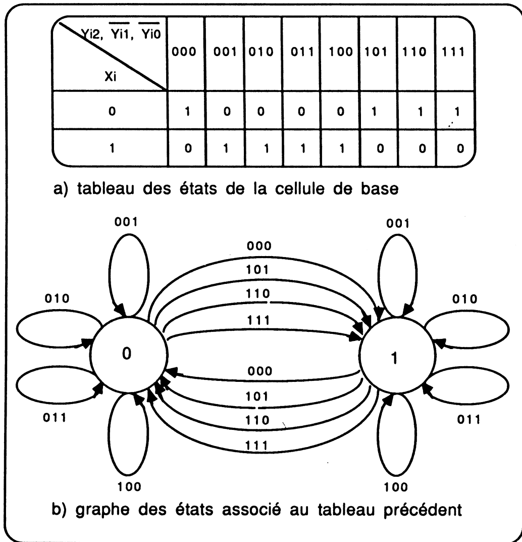
Figure 4.25 : tableau des états et graphe de la cellule de base du circuit de signature intégré au sein du microprocesseur.
