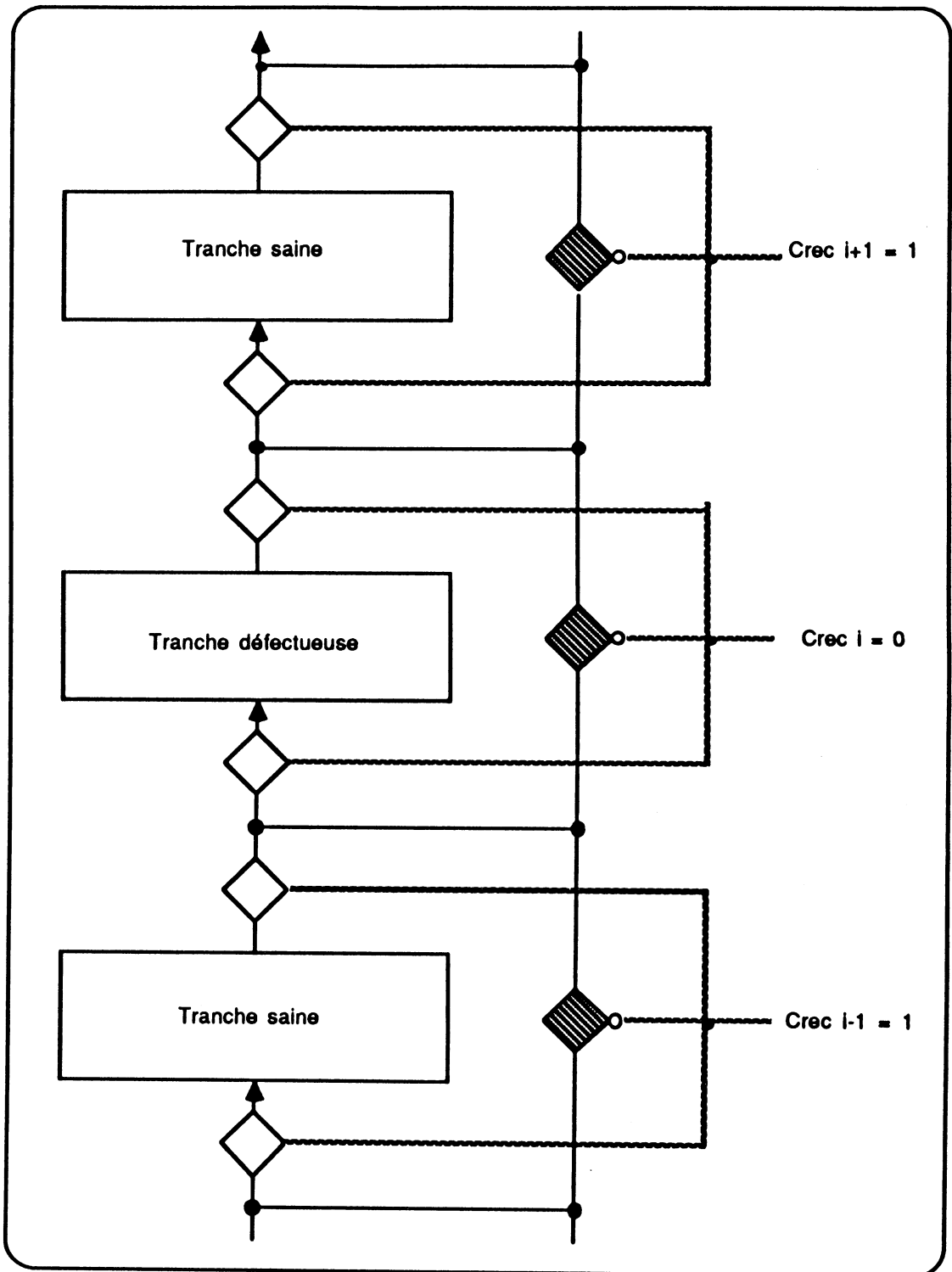
Figure 2.4 : reconfiguration des signaux propagés entre les tranches.
