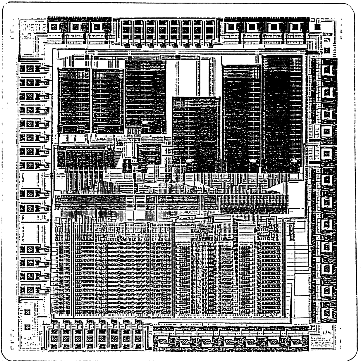
Figure 2.8 : dessin des masques du composant complet.
