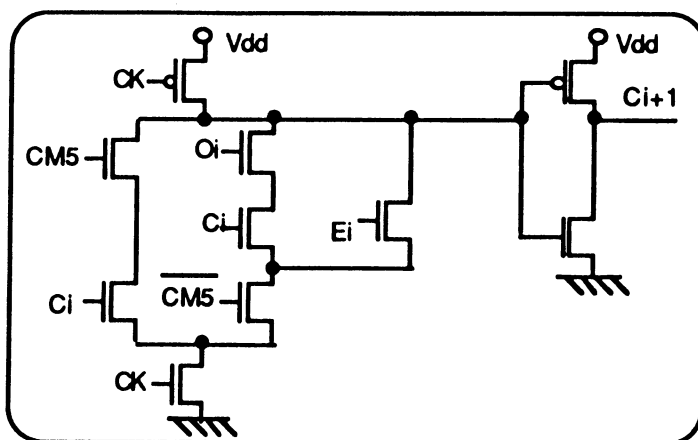
Figure 3.14 : schéma électrique du bloc de la retenue.
