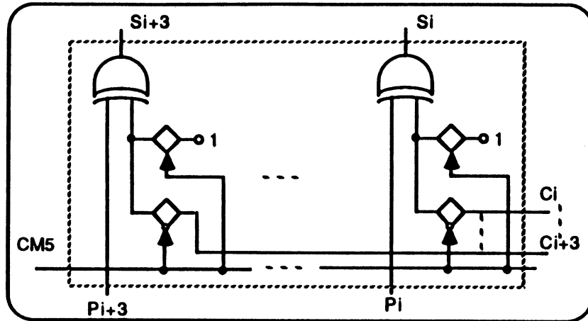
Figure 3.37 : schéma logique du bloc BS.
