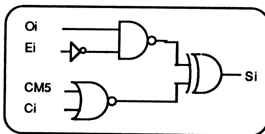
Figure 3.15 : schéma logique du bloc de sortie.
