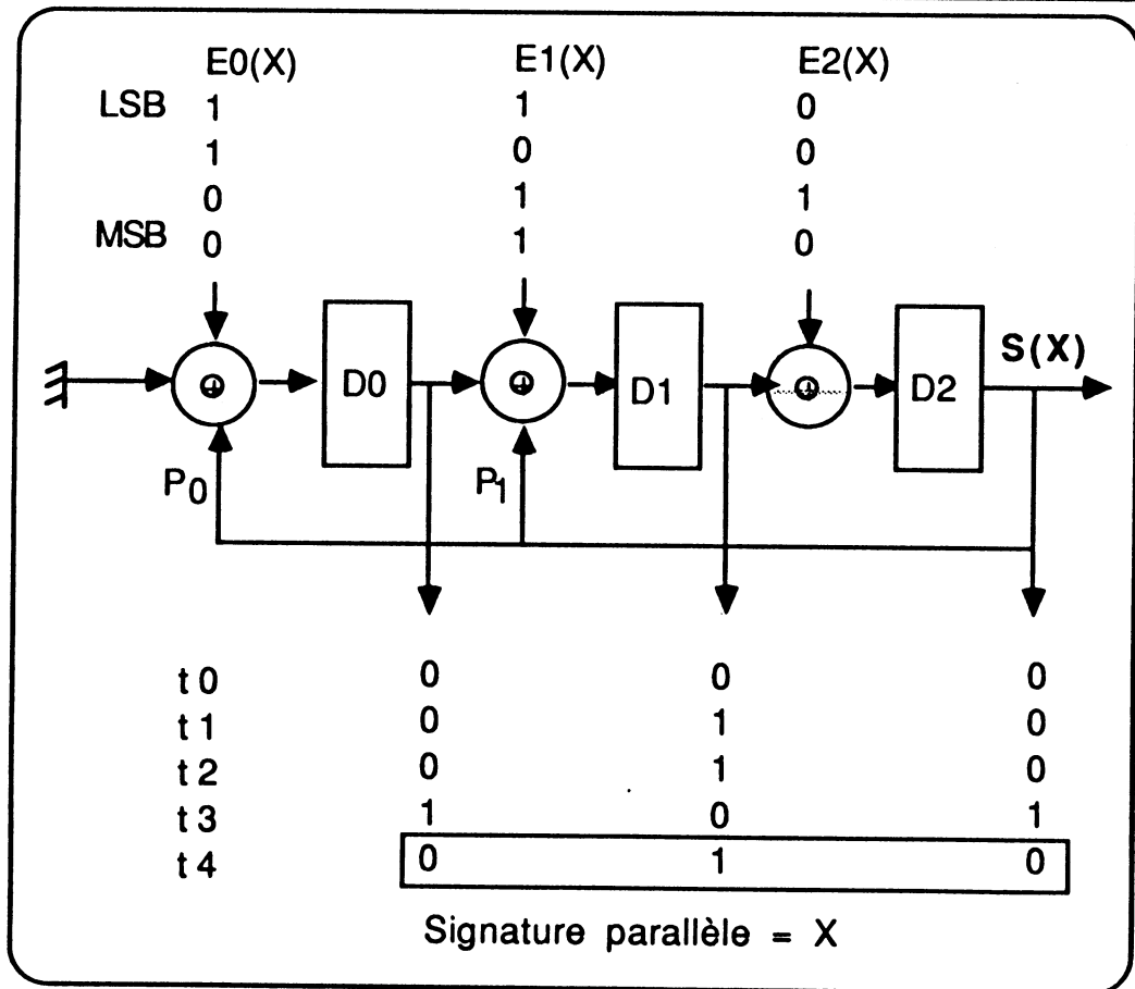
Figure 4.5 : Equivalence entre circuits de signature série et parallèle.
