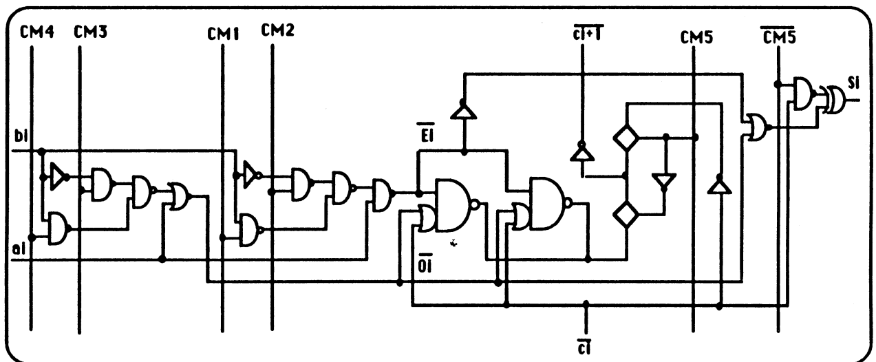
Figure 3.5 : schéma logique d'une tranche de l'UAL.
