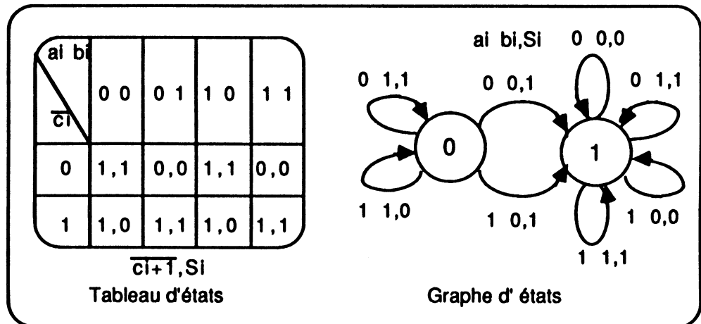
Figure 3.9 : tableau et graphe des états de l'opération INC.
