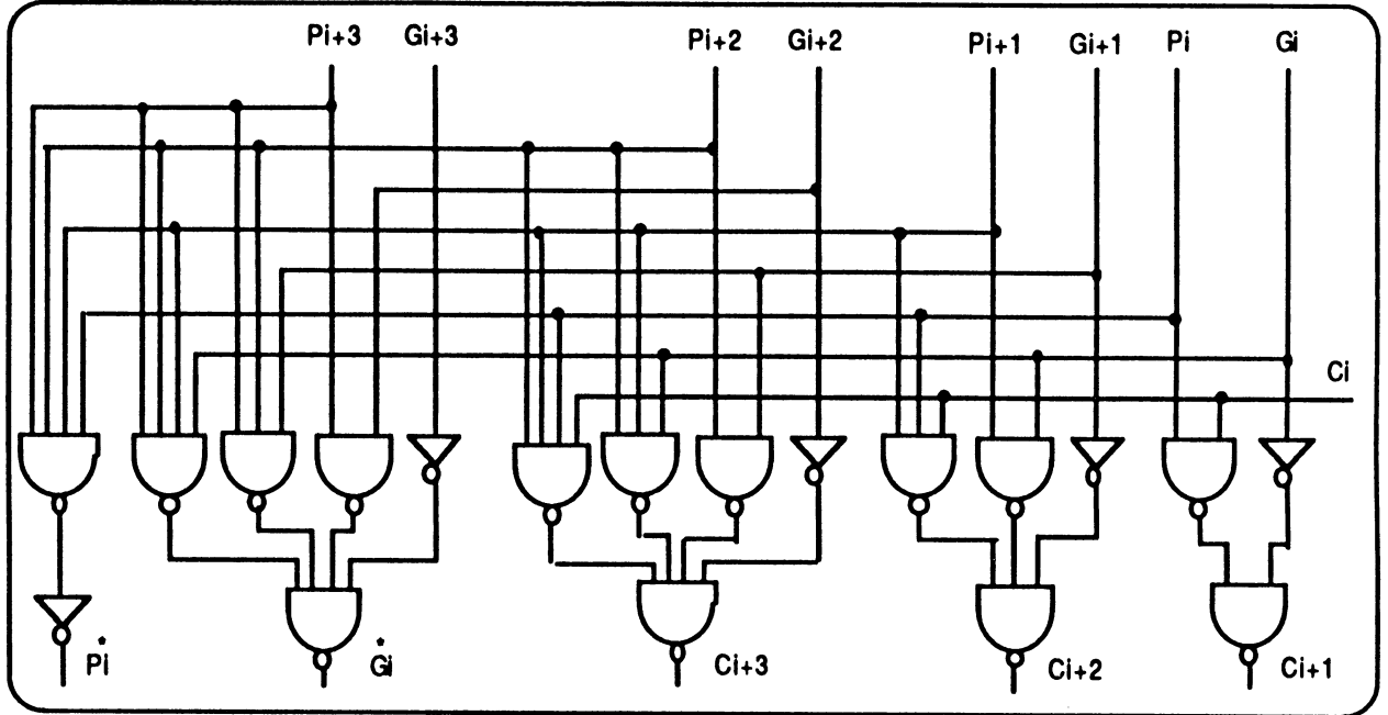
Figure 3.35 : schéma logique du bloc CLA1.
