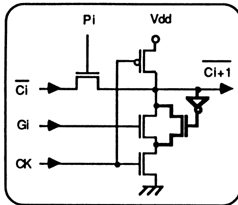
Figure 3.20 : circuit de décharge de la ligne de retenue.
