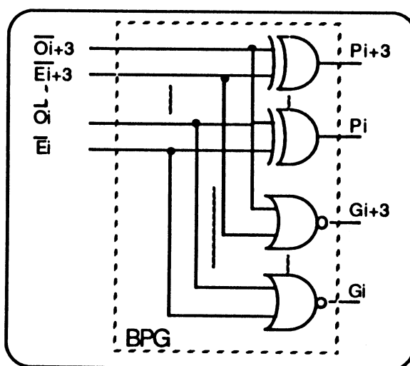
Figure 3.34 : schéma logique du bloc BPG.
