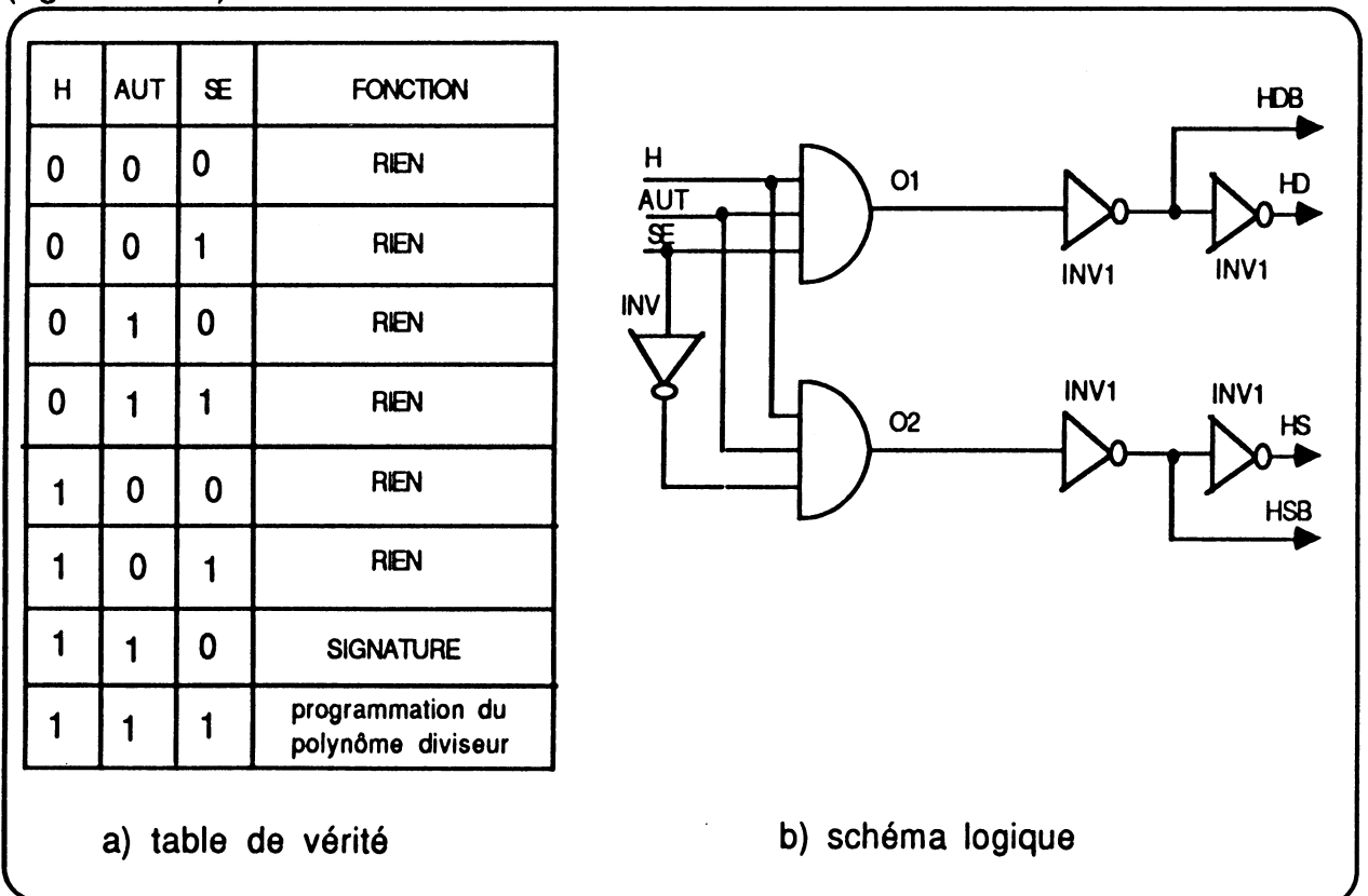
Figure 4.8 : table de vérité et circuit de commande correspondant.
