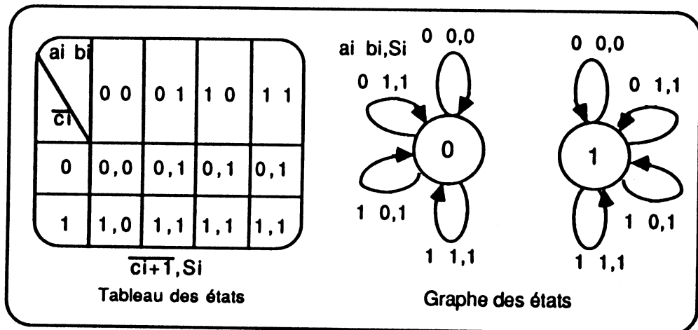
Figure 3.7 : Tableau et graphe des états de l'opération OR.
