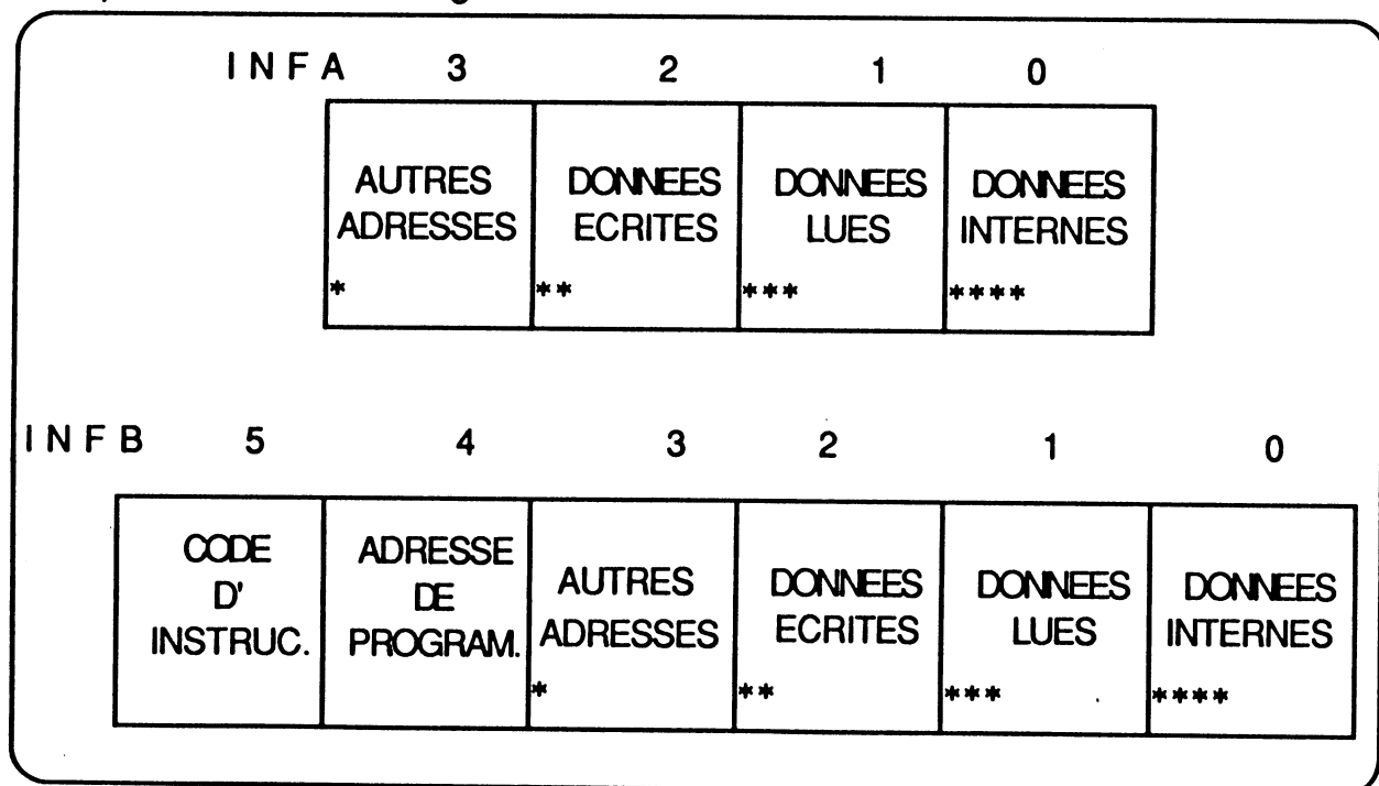
Figure 4.14 : signification des champs de commande INFA et INFB.
