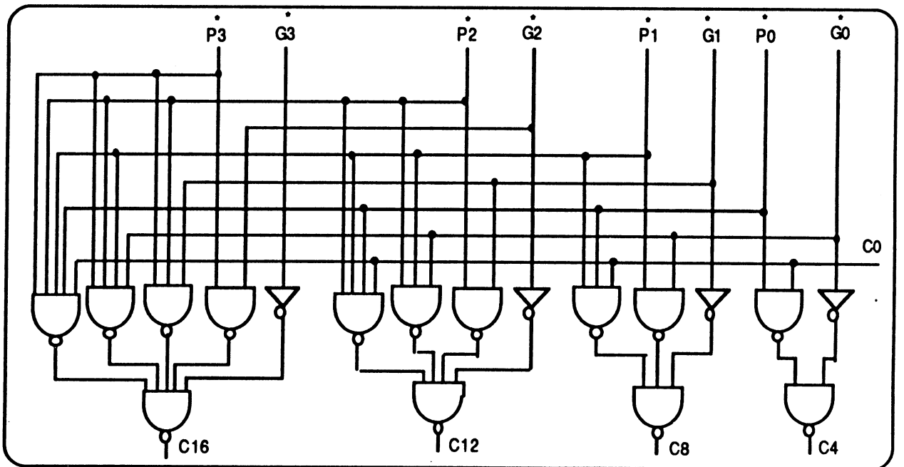
Figure 3.36 : schéma logique du bloc CLA2.
