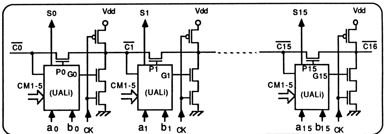
Figure 3.17 : schéma simplifié de l'UAL Manchester.
