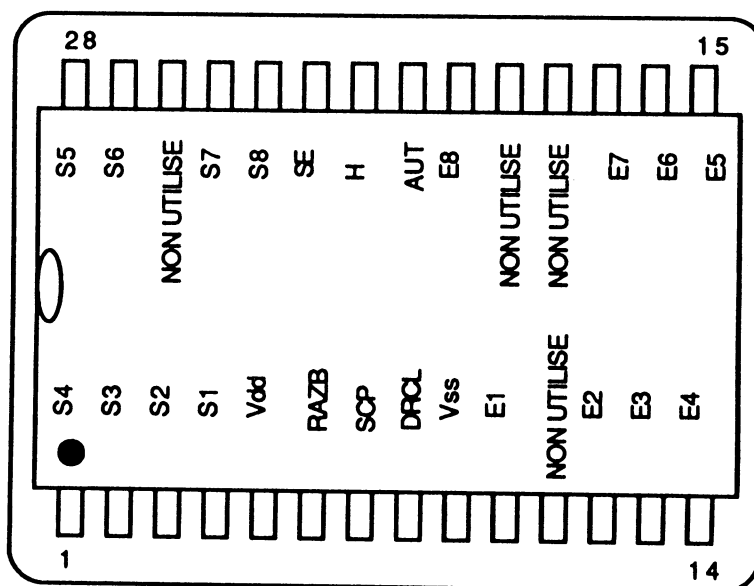
Figure 4.11 : boîtier du circuit de signature universel.
