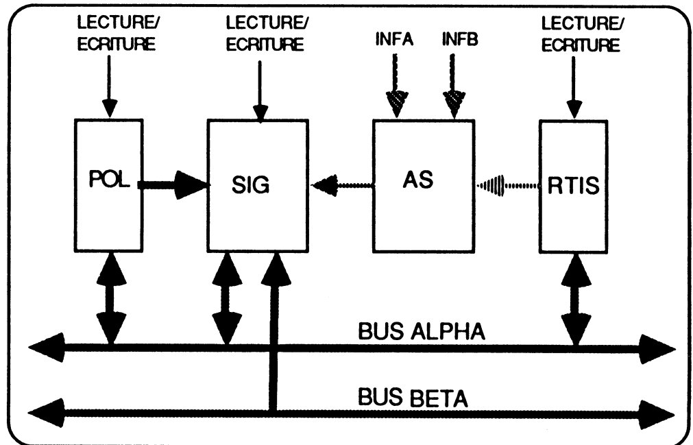
Figure 4.13 : schéma général du dispositif de signature.
