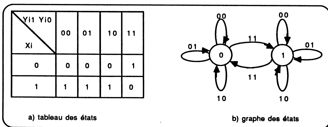
Figure 4.20 : tableau des états et son graphe associé.
