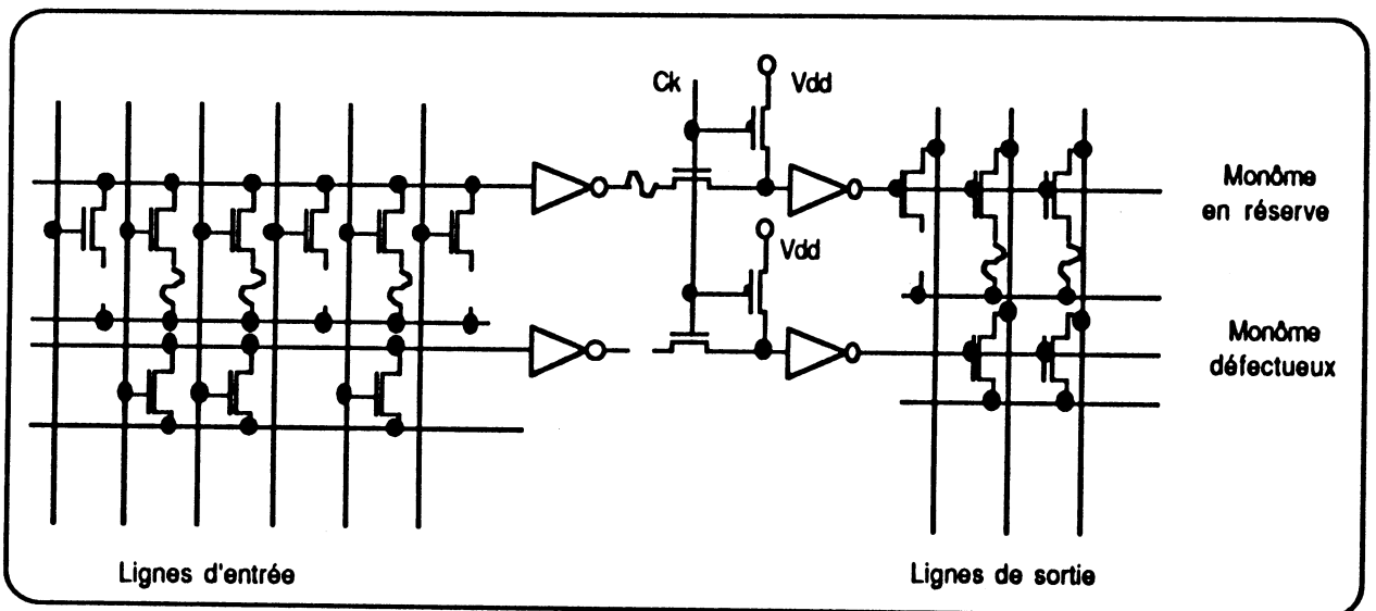
Figure 2.7 : reconfiguration dans un PLA.
