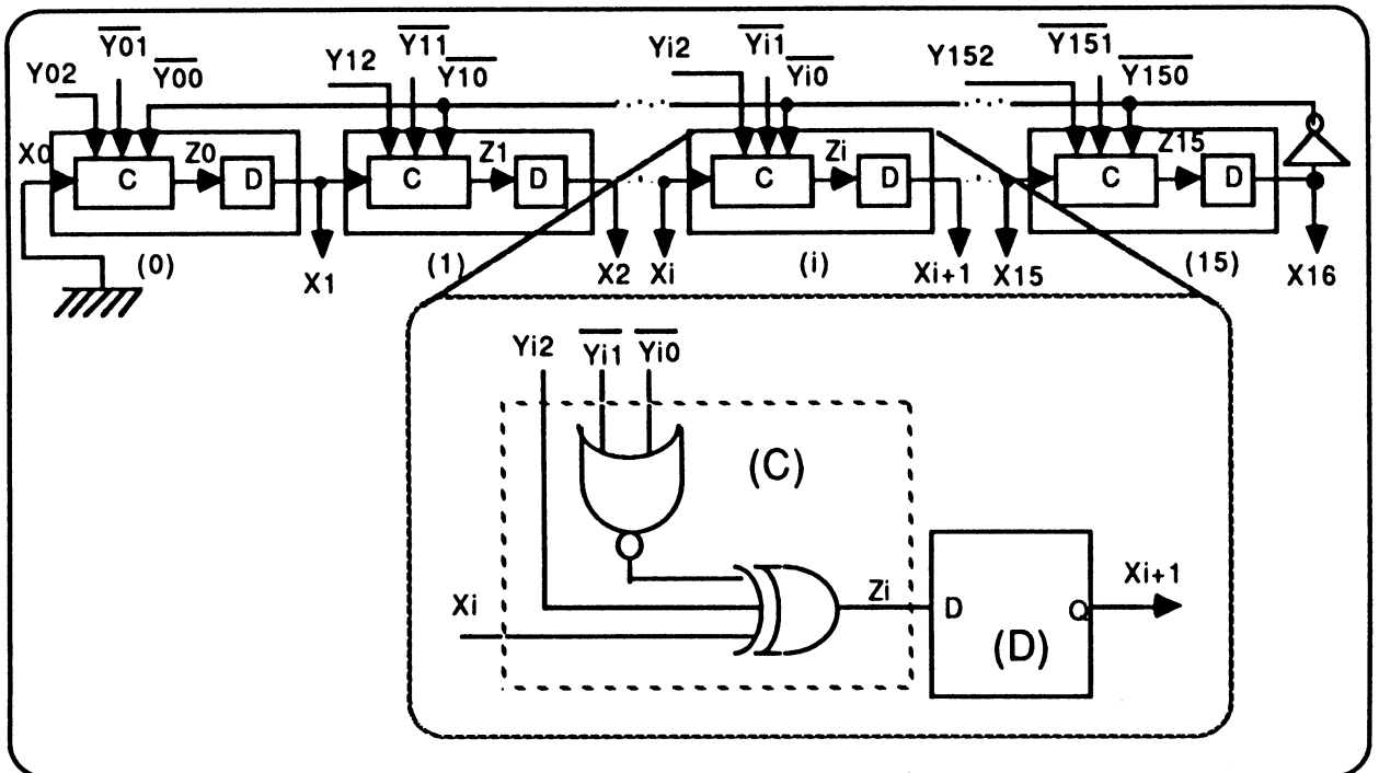
Figure 4.26 : schéma général du circuit non modifié.
