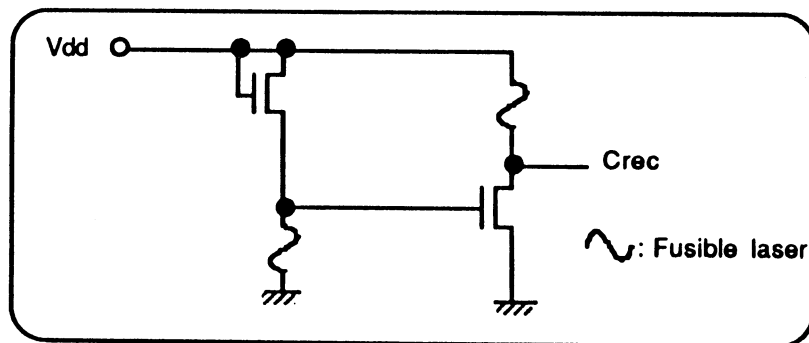
Figure 2.2 : circuit utilisé pour générer le signal Crec.
