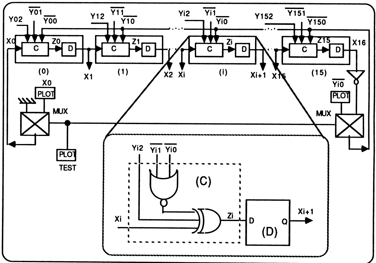
Figure 4.24 : schéma du circuit de signature à entrées parallèles modifié.
