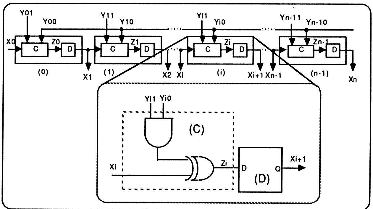
Figure 4.19 : schéma général du circuit de signature à entrée série.
