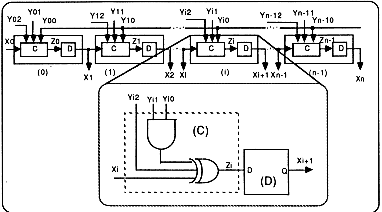
Figure 4.21 : schéma général du circuit de signature à entrées parallèles avec un polynôme diviseur programmable.
