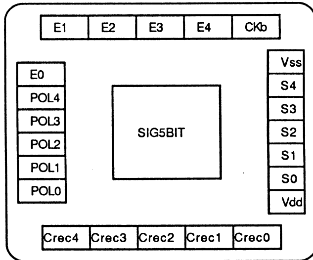
Figure 4.17 : plan de masse du circuit de signature sur 5 bits.
