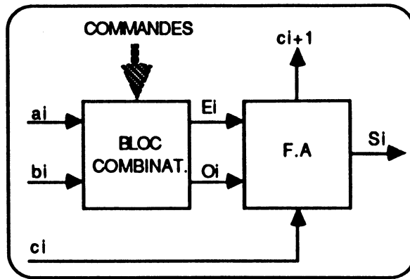
Figure 3. 4 : schéma général d'1 bit de l'UAL.
