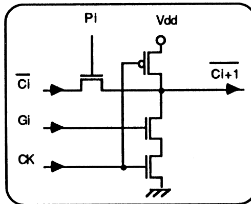
Figure 3.16 : chaîne de retenue Manchester.
