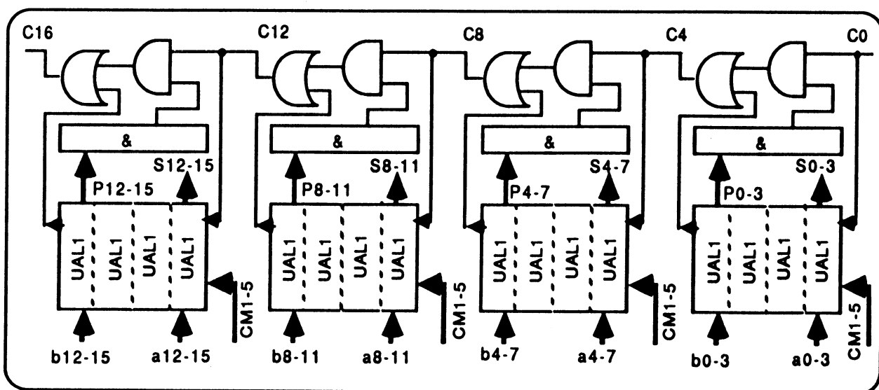
Figure 3.28 : schéma général de l'UAL "Carry-Skip".
