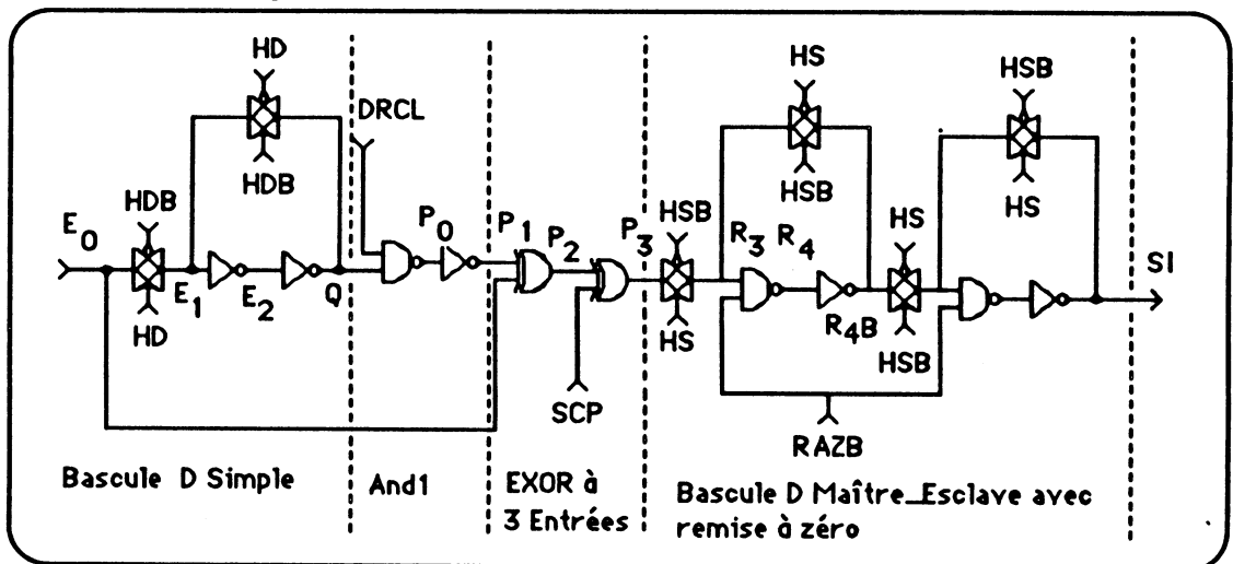
Figure 4.7 : schéma logique de 1 bit du circuit de signature.
