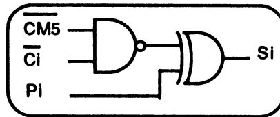
Figure 3.24 : schéma logique du bloc BAD.
