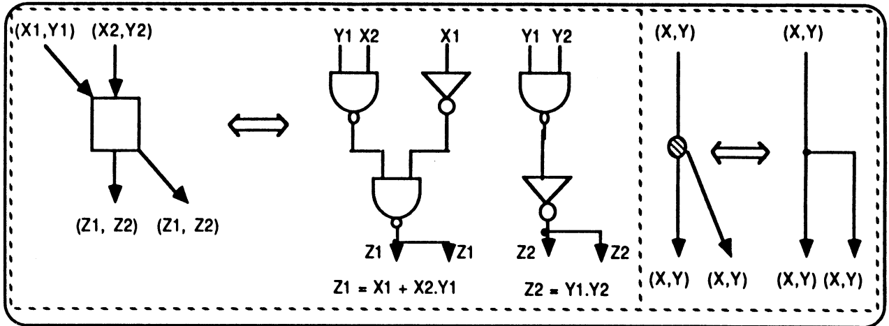
Figure 3.42 : schéma logique de l'opérateur O.
