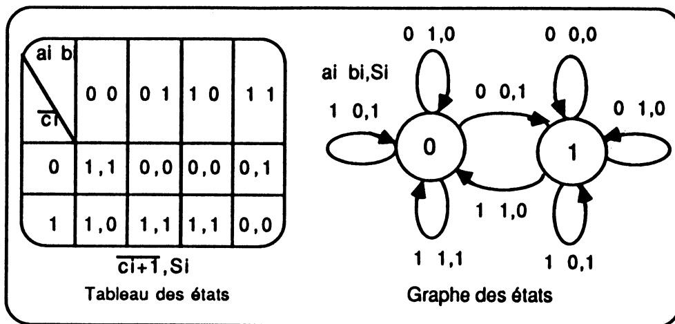
Figure 3.8 : tableau et graphe des états de l'opération ADD.
