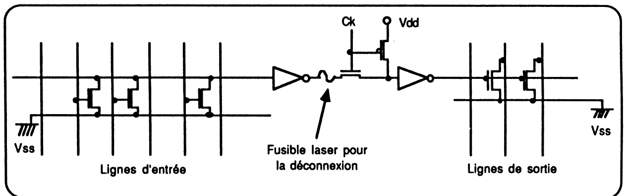
Figure 2.5 : monôme normal d'un PLA reconfigurable.
