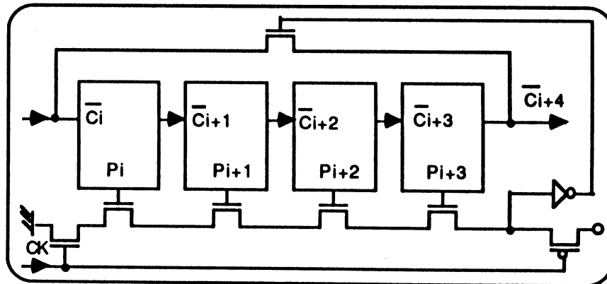
Figure 3.19 : technique d'accélération de la retenue.
