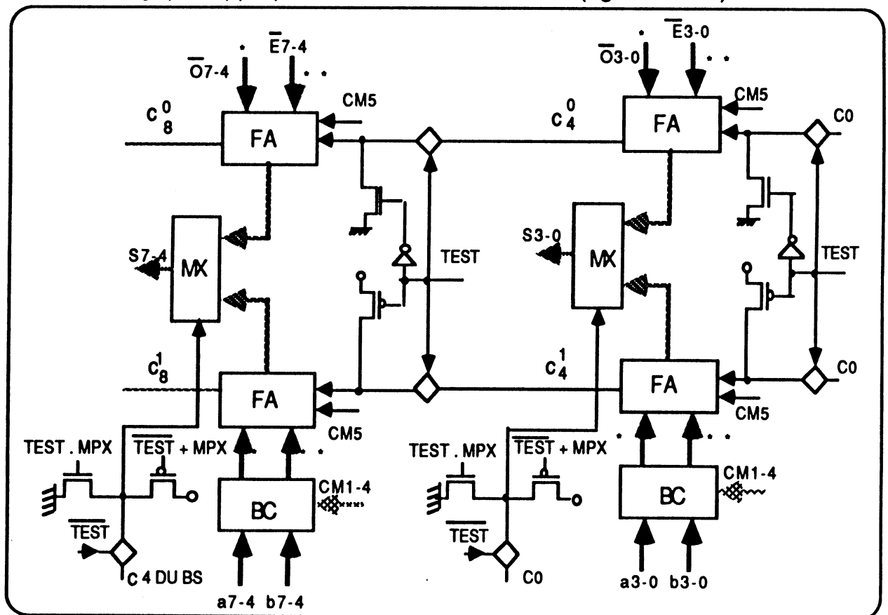
Figure 3. 27 : principe de test de l'UAL.
