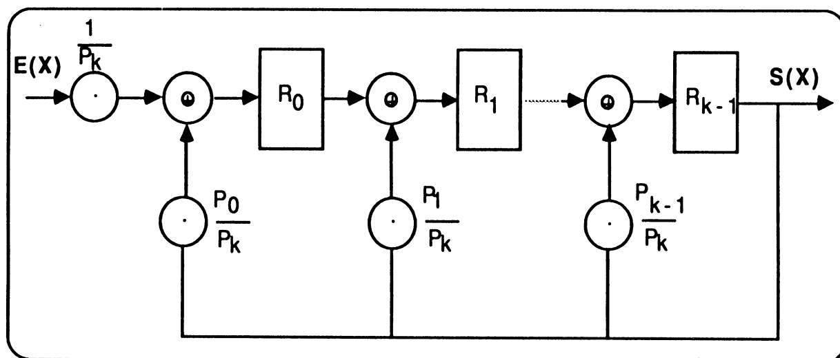
Figure 4.2 : circuit diviseur.
