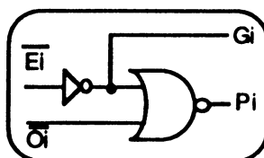
Figure 3.22 : schéma logique du bloc BPG.
