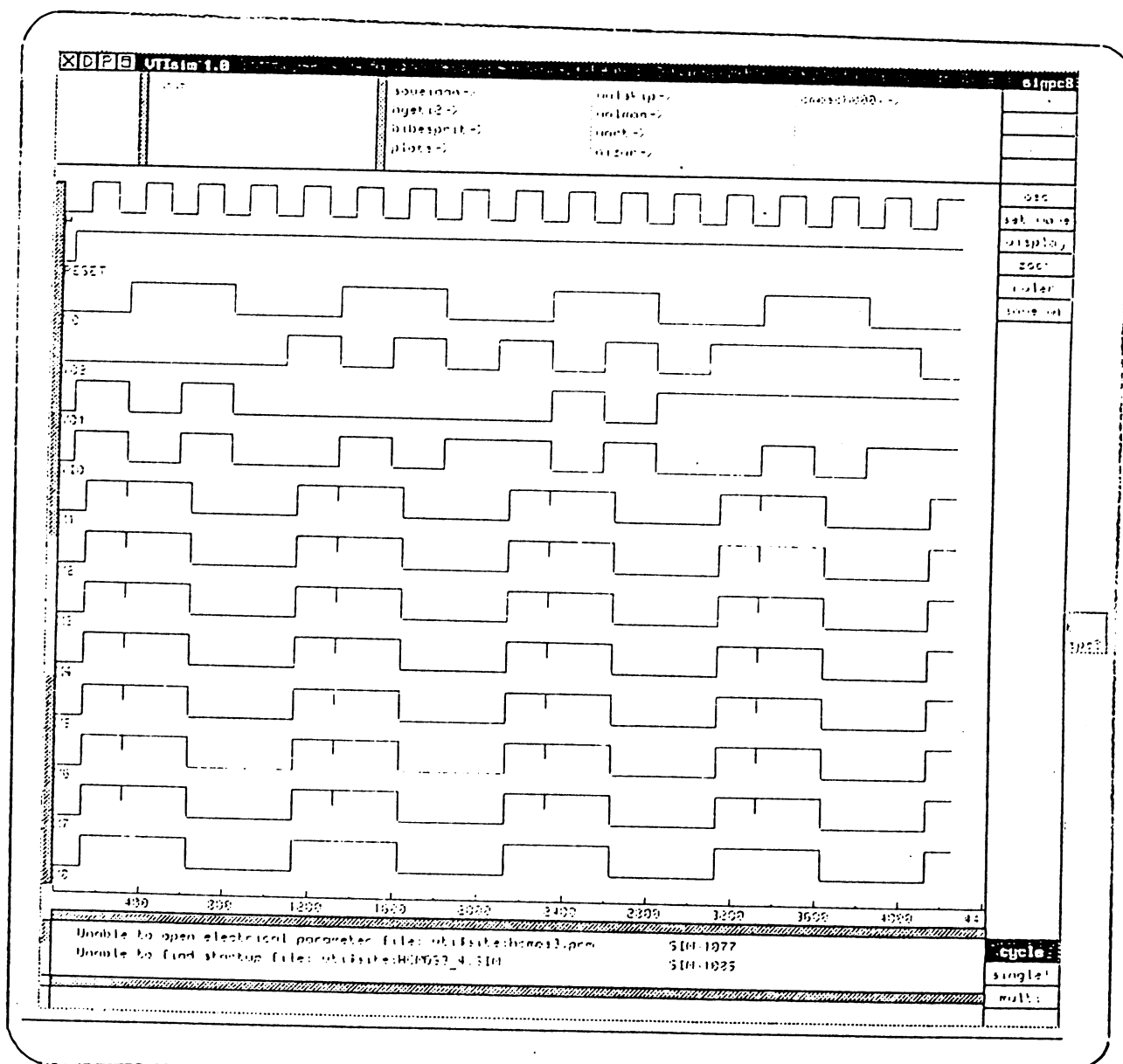
Figure 4.23 : Résultat de la simulation logique.
