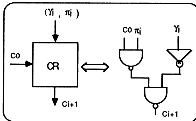
Figure 3.43 : circuit logique du bloc CR.
