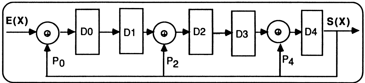
Figure 4.3 : Schéma d'un circuit de signature série
