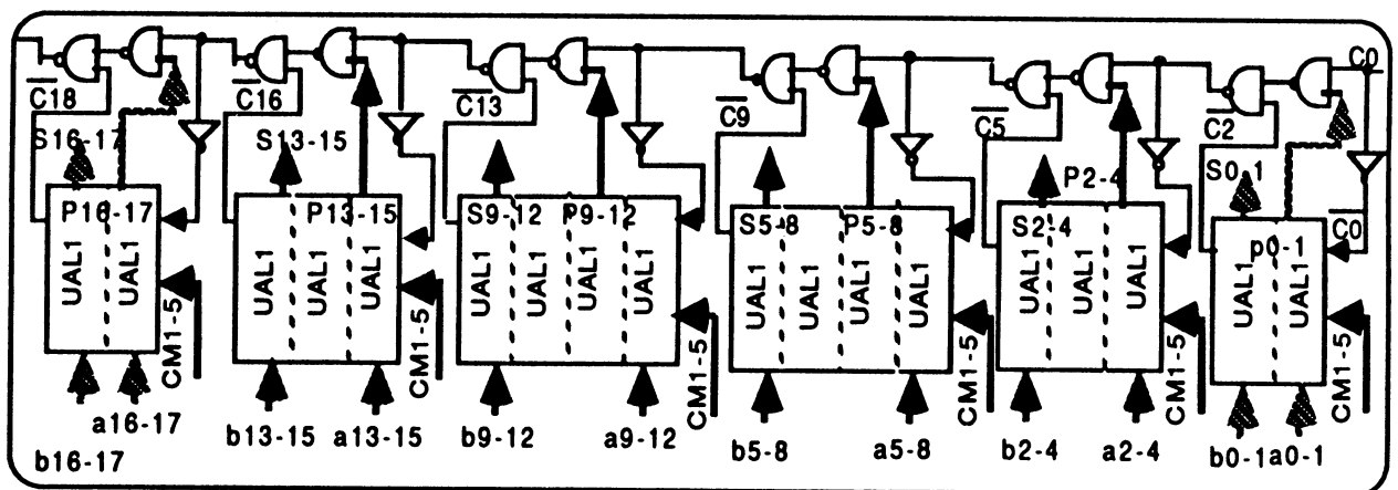
Figure 3.30 : schéma de l'UAL "Carry-Skip" en blocs de tailles distinctes.
