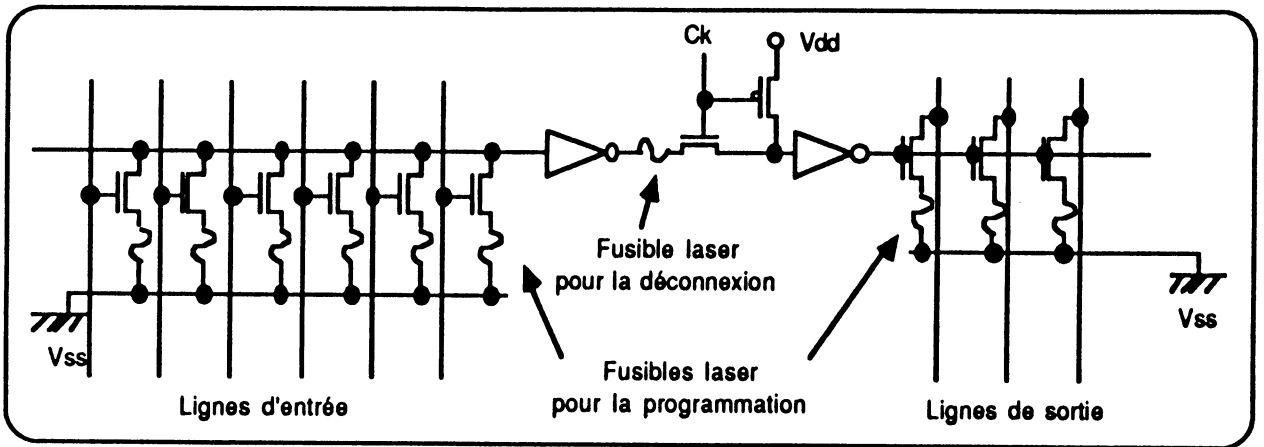
Figure 2.6 : monôme programmable d'un PLA reconfigurable.
