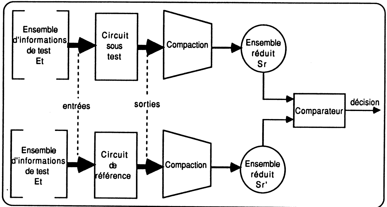
Figure 4.1 : stratégie de test
