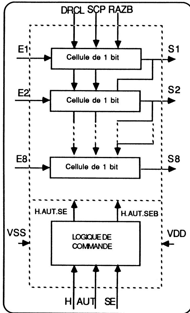
Figure 4.6 : circuit de signature parallèle sur 8 bits.
