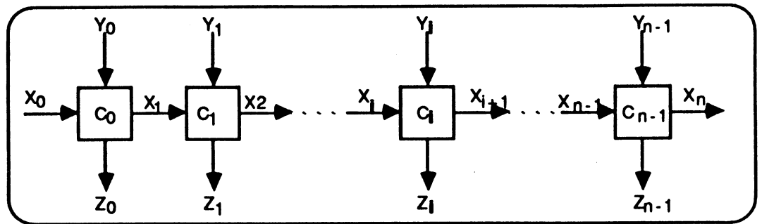
Figure 3.1 : réseau logique itératif
