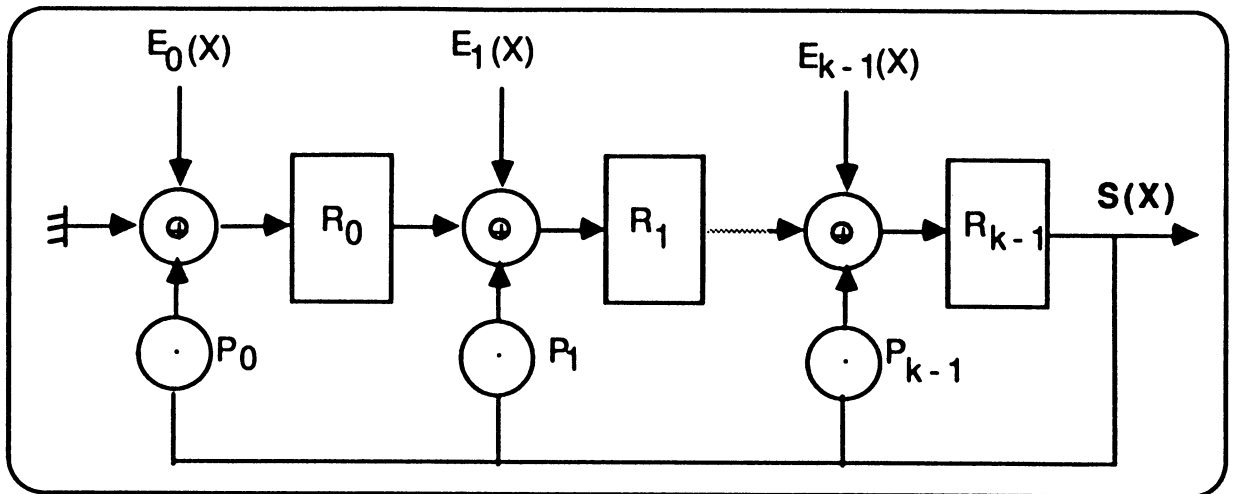
Figure 4.4 : Structure parallèle générale du circuit de signature.
