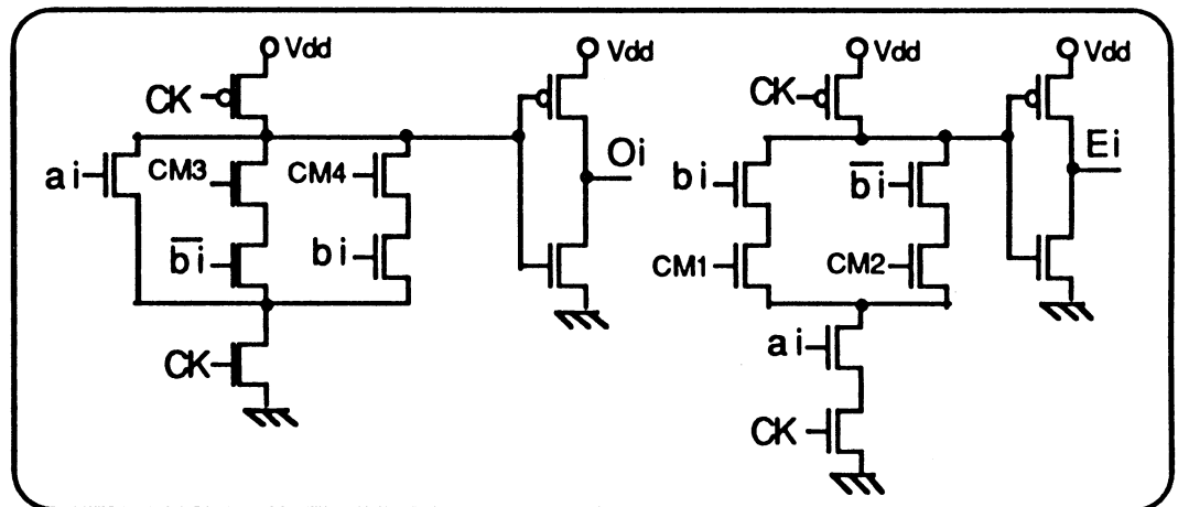
Figure 3.13 : schéma électrique réalisant les deux fonctions O_i et E_i .
