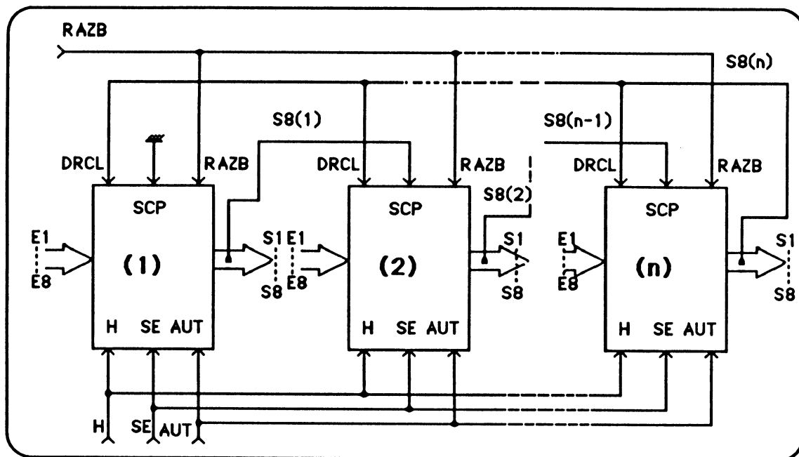
Figure 4.12 : schéma d'application de plusieurs boîtiers.
