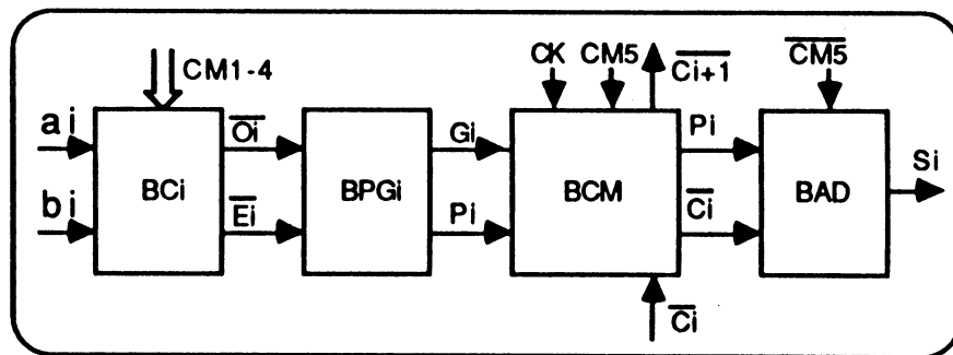
Figure 3.21 : schéma d'une tranche de l'UAL du type Manchester.
