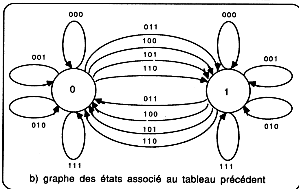
Figure 4.22 : tableau des états et graphe correspondant à la cellule de base d'un circuit de signature à entrées parallèles.
