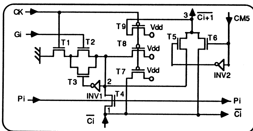
Figure 3.23 : schéma électrique du bloc BCM.
