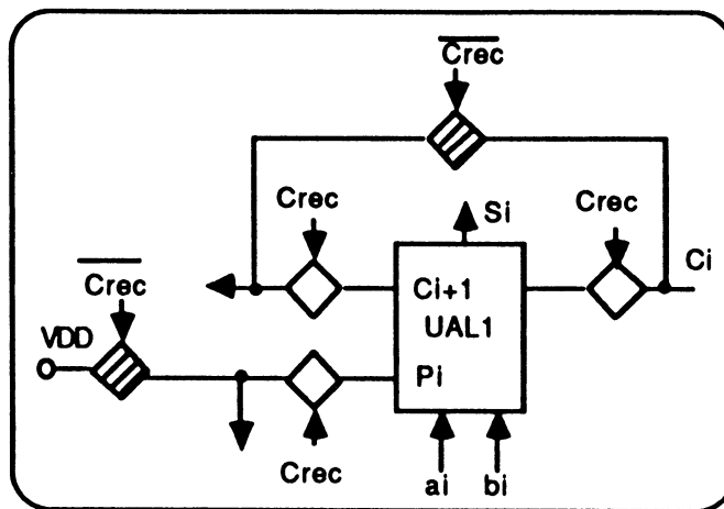
Figure 3.32 : schéma de principe de reconfiguration de l'UAL "Carry-Skip".
