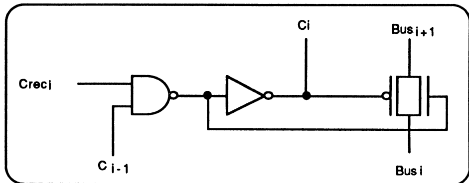
Figure 2.3 : circuit de connexion pour les tranches 1 \leq i \leq 15 .
