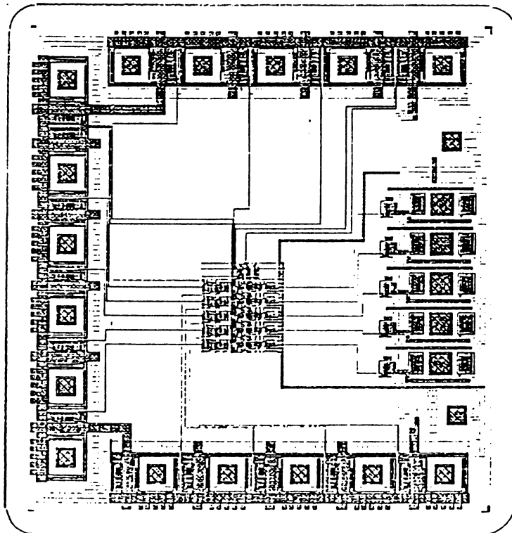
Figure 4.18 : Dessin au micron du circuit de signature sur 5 bits.
