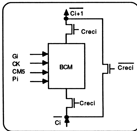
Figure 3.25 : schéma de principe de la reconfiguration.
