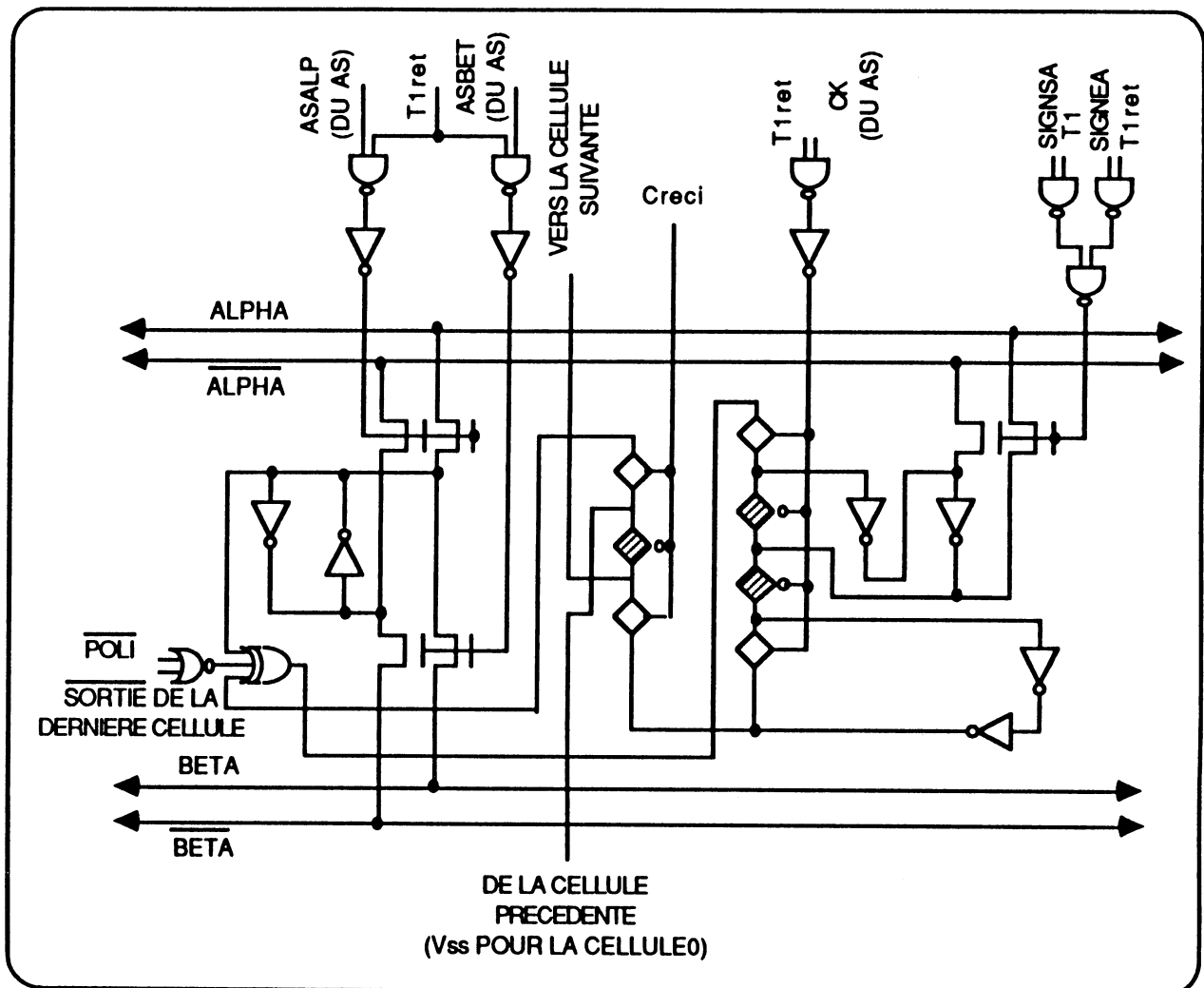
Figure 4.16 : schéma logique d'un bit du registre SIG.
