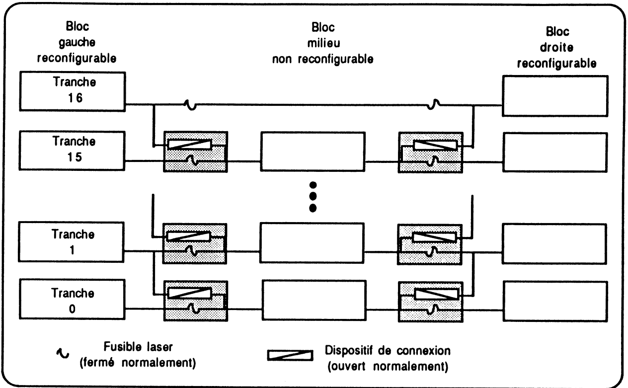
Figure 2.1 : plan général de la partie opérative.
