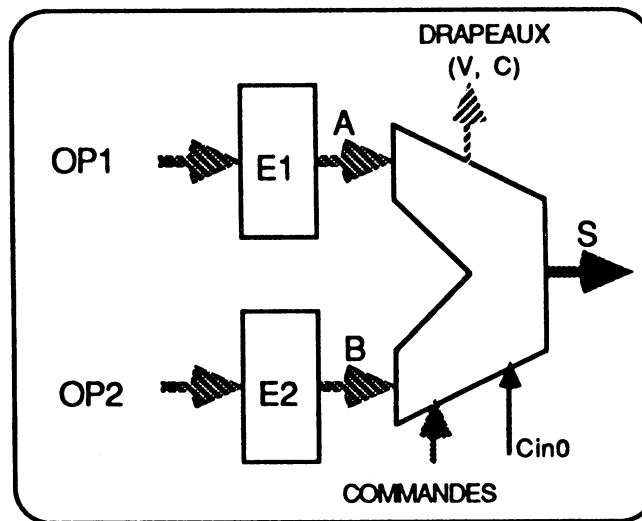
Figure 3.3 : schéma général de l'UAL.
