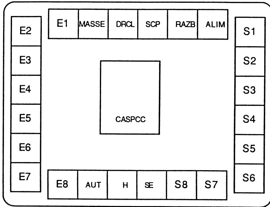
Figure 4.9 : plan de masse du circuit de signature universel.
