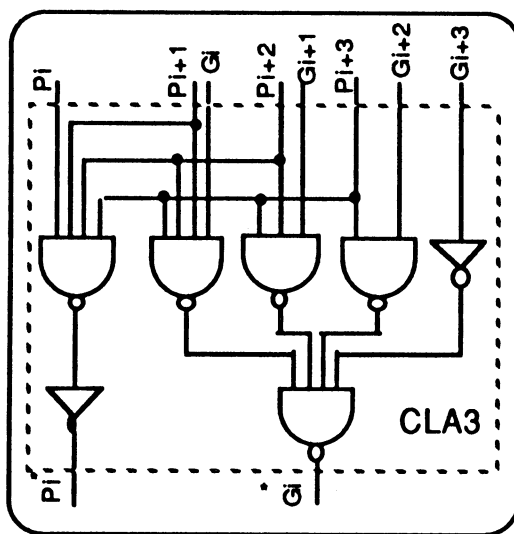
Figure 3.38 : schéma logique du bloc CLA3
