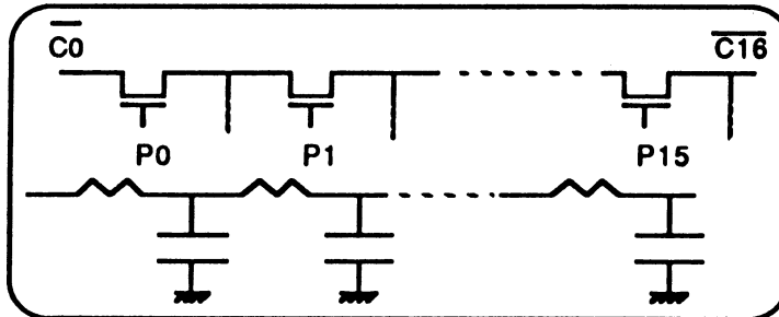
Figure 3.18 : correspondance RC de la chaîne de transistors .
