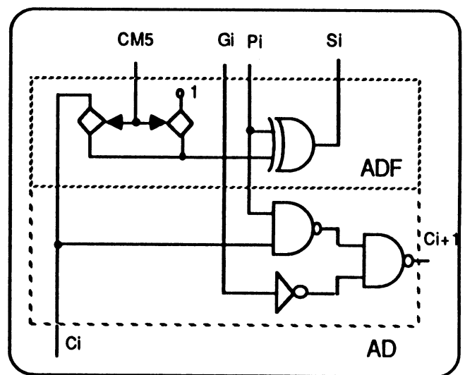
Figure 3.39 : schéma logique du AD et ADF
