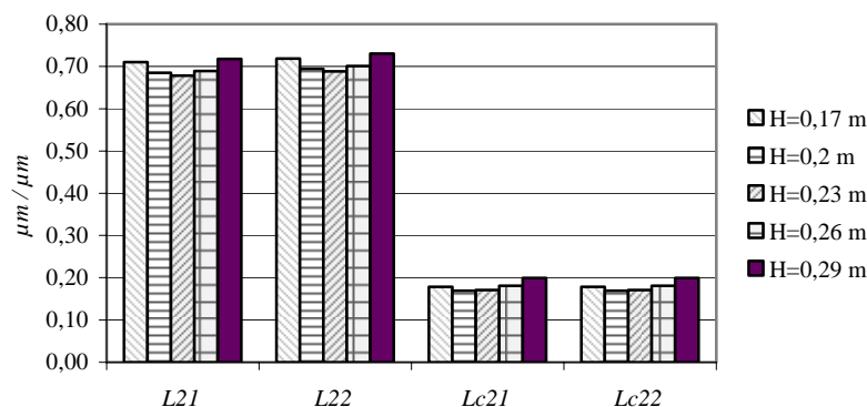
Figure 2.29 – Longueur d'outil optimale. Sensibilité moyenne de la position de l'extrémité de l'outil aux variations des paramètres dimensionnels
