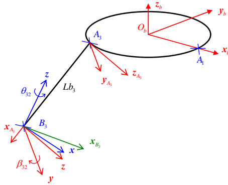
Figure 2.15 – Expression des repères R_{B_i} dans R_{A_i}
