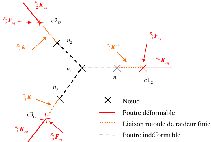
Figure 3.20 – Modélisation de la structure complète du Delta
