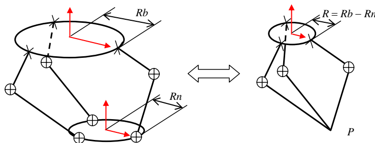
Figure 2.6 – Structure équivalente
