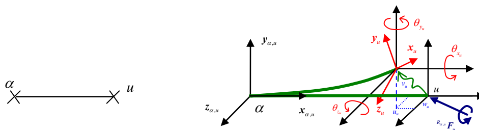
Figure 3.2 – Effort nodal et déplacement nodal
