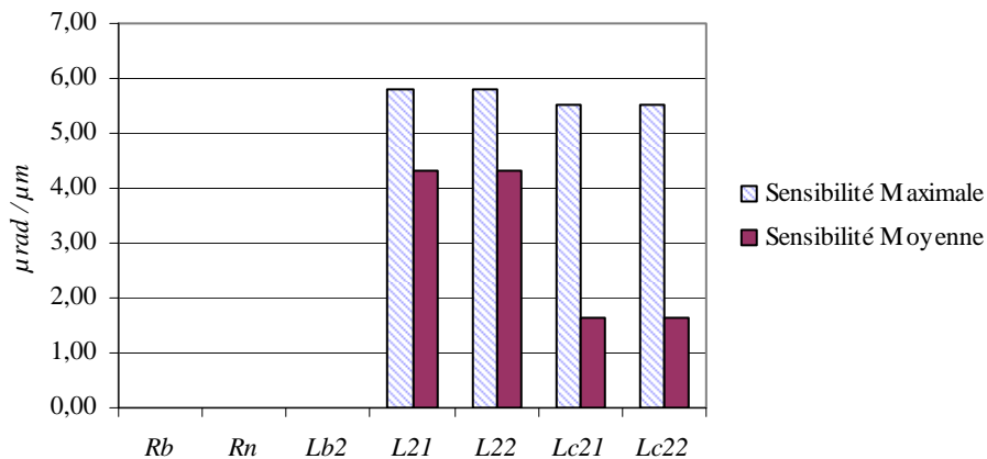
Figure 2.22 – Indice de sensibilité \mu_r . Sensibilité de l'orientation de la nacelle aux paramètres dimensionnels
