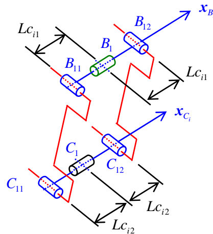
Figure 2.18 – Position des points B_{ij} et C_{ij}
