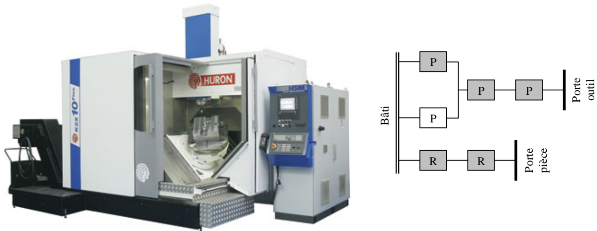
Figure 1.3 – Machine outil K2X 10 Five (HURON) : photo et graphe d'agencement
