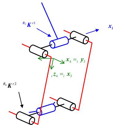
Figure 3.21 – Liaisons rotoïdes passives
