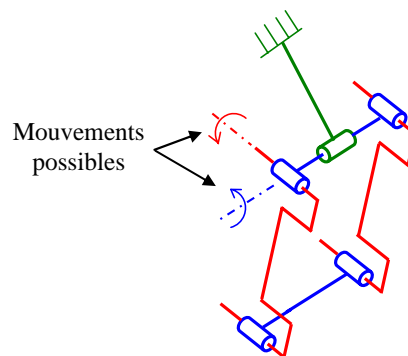
Figure 3.17 – Mobilité d’une chaîne cinématique
