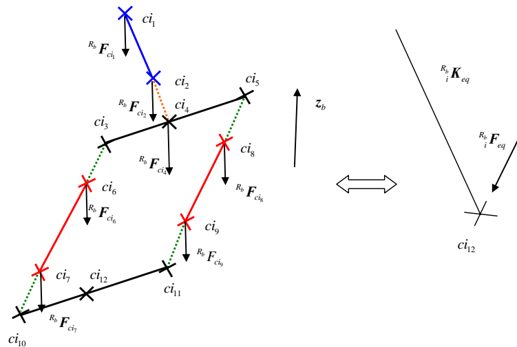
Figure 4.2 – Modélisation du poids propre d'une chaîne cinématique
