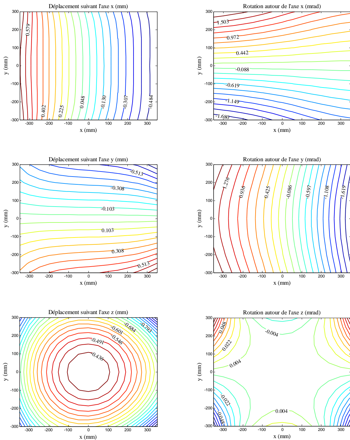
Figure 4.5 – Déplacement sous le poids propre de la structure dans le plan z = -1,2\text{ m}
