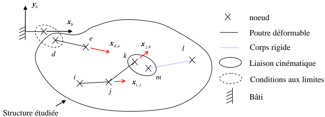
Figure 3.1 – Modélisation partielle d'une structure quelconque
