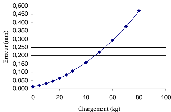
Figure 4.7 – Erreur maximale dans le volume de travail en fonction de la charge sur la nacelle
