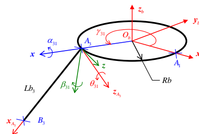
Figure 2.8 – Position des points B_i dans R_b
