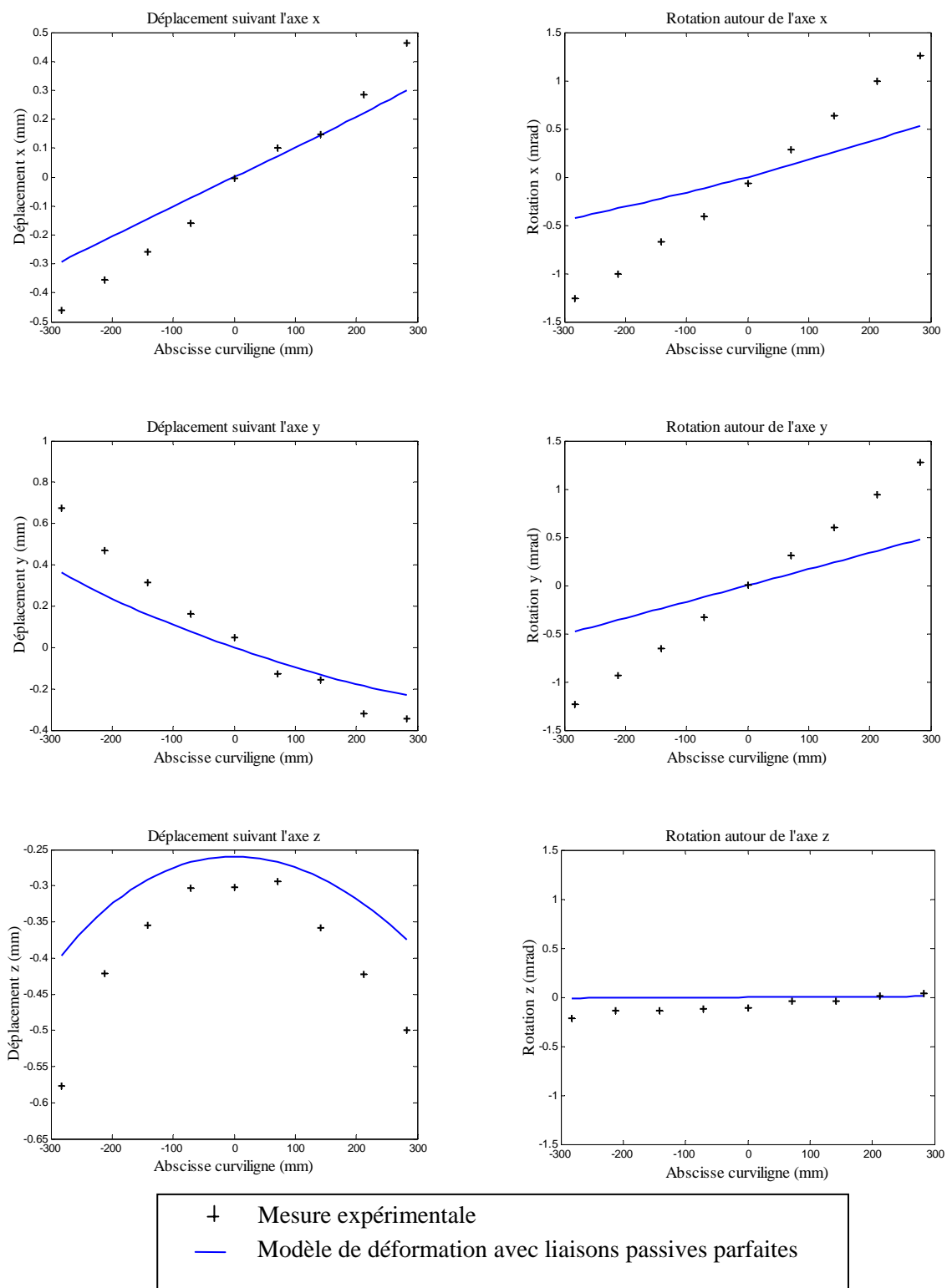
Figure 3.14 – Modèle avec liaisons passives parfaites. Charge de 19,5 kg
