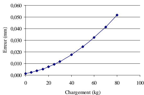
Figure 4.8 – Erreur moyenne dans le volume de travail en fonction de la charge sur la nacelle
