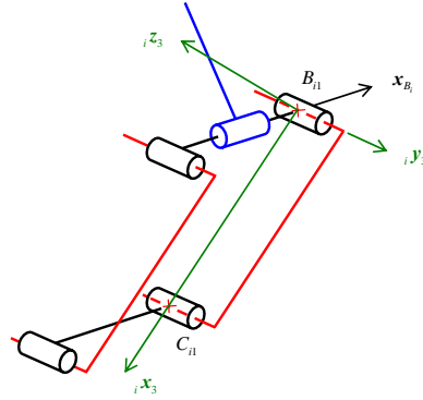
Figure 3.8 – Repère associé au grand côté du parallélogramme
