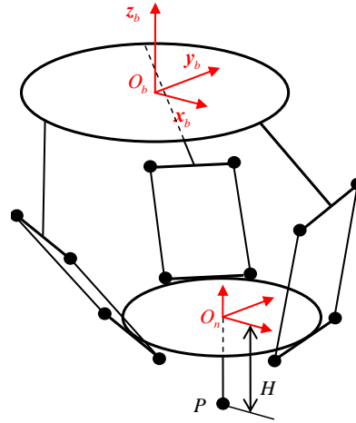
Figure 2.24 – Structure Delta avec un outil
