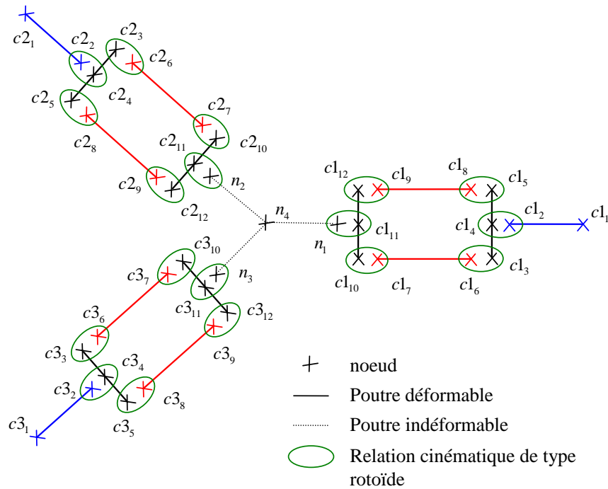
Figure 3.7 – Modélisation de la structure complète
