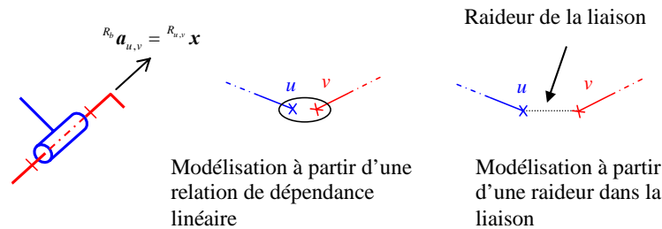
Figure 3.16 – Rigidité d’une liaison rotoïde passive
