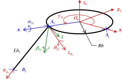
Figure 2.14 – Expression des repères R_{A_i} dans R_b
