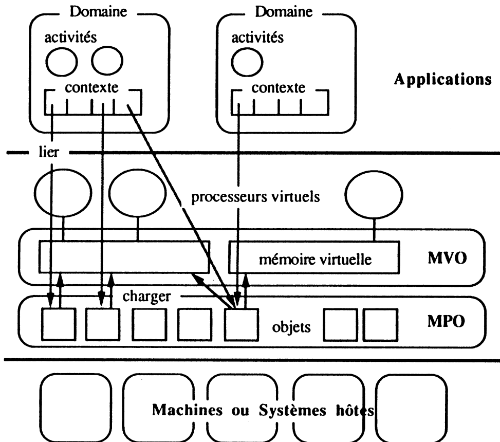
Figure 1. Architecture de la machine virtuelle Guide
