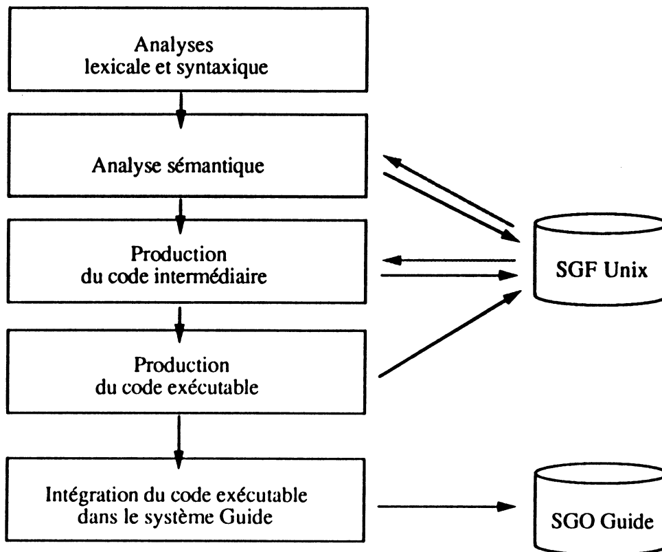
Figure 2. Architecture du compilateur Guide
