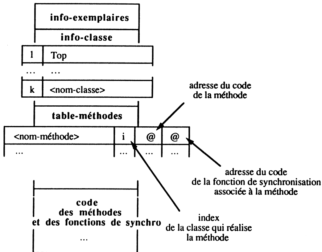
Figure 1. Etat d'un objet classe
