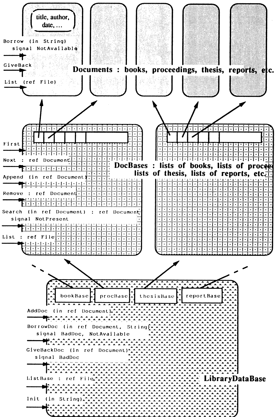
Figure 3. Objets permanents qui constituent l'application Bibliographique
