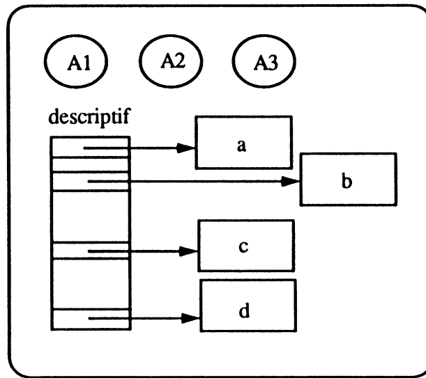
Figure 4. Représentation d'un domaine
