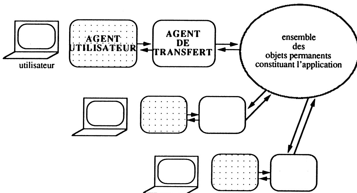
Figure 1. Agents utilisateur et Agents de transfert
