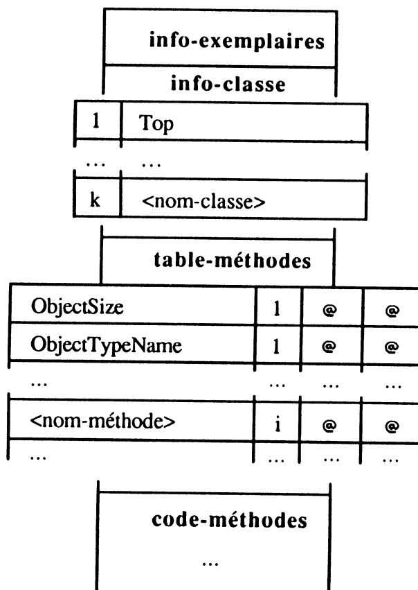
Figure 3. Structure de l'état d'un objet classe
