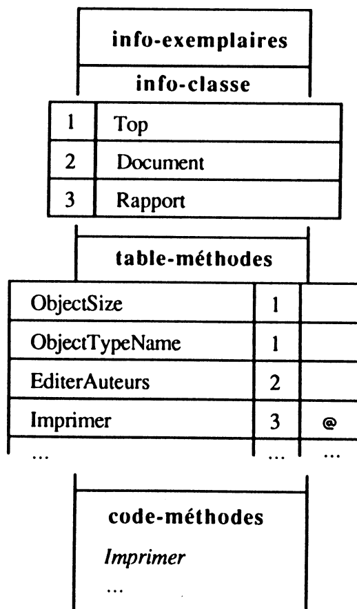
Figure 6. Structure de l'état de l'objet classe Rapport
