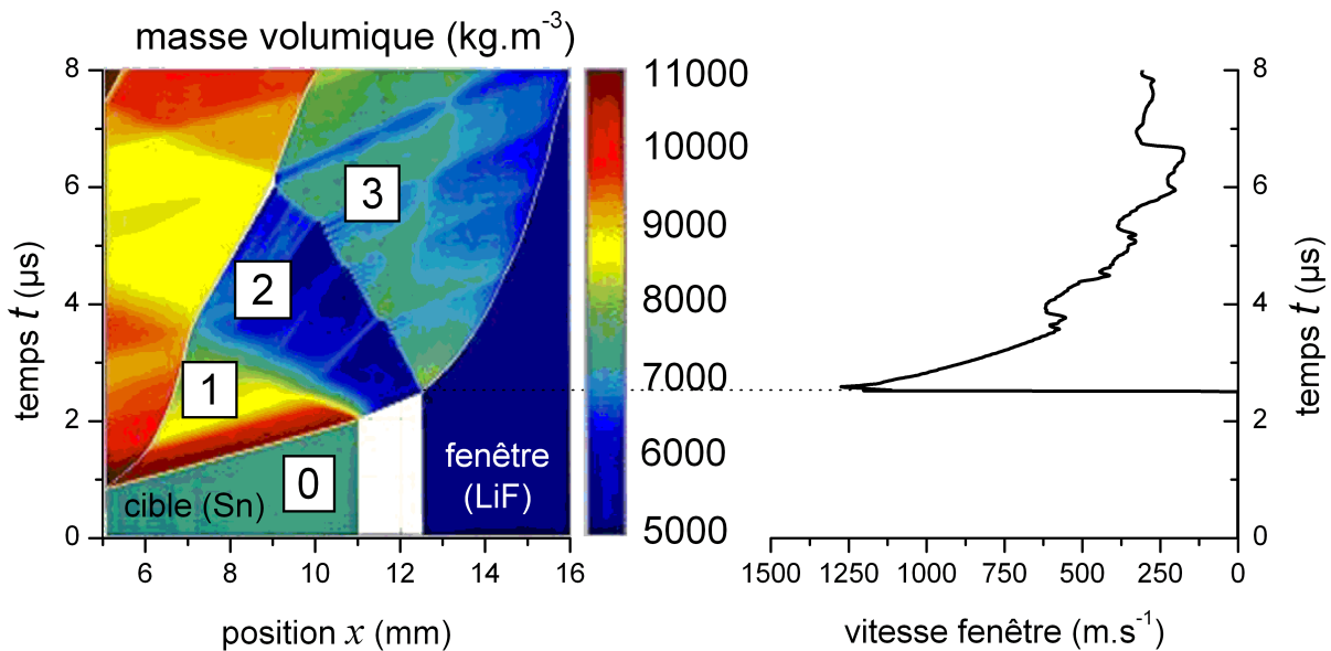
FIG. II.8: (à gauche) Evolution du champ de masse volumique, représenté dans le plan x-t , au cours d'une simulation simple d'un essai de micro-écaillage réalisé par impact de plaque avec une fenêtre détachée. La région 0 correspond à la cible d'étain dans son état solide initial. La zone 1 représente l'état de compression après le passage du front de choc. Dans la région 2, on assiste à l'apparition du micro-écaillage. L'étain est éjecté à grande vitesse et sa masse volumique, qui représente la masse volumique apparente du nuage de fragments, chute en dessous de celle de l'étain liquide intact comprise entre 6500 et 7000 \text{kg.m}^{-3} . Après l'impact sur la fenêtre en LiF, le milieu micro-écaillé est redensifié (zone 3). (à droite) Histoire des vitesses simulées de la surface d'impact de la fenêtre.
