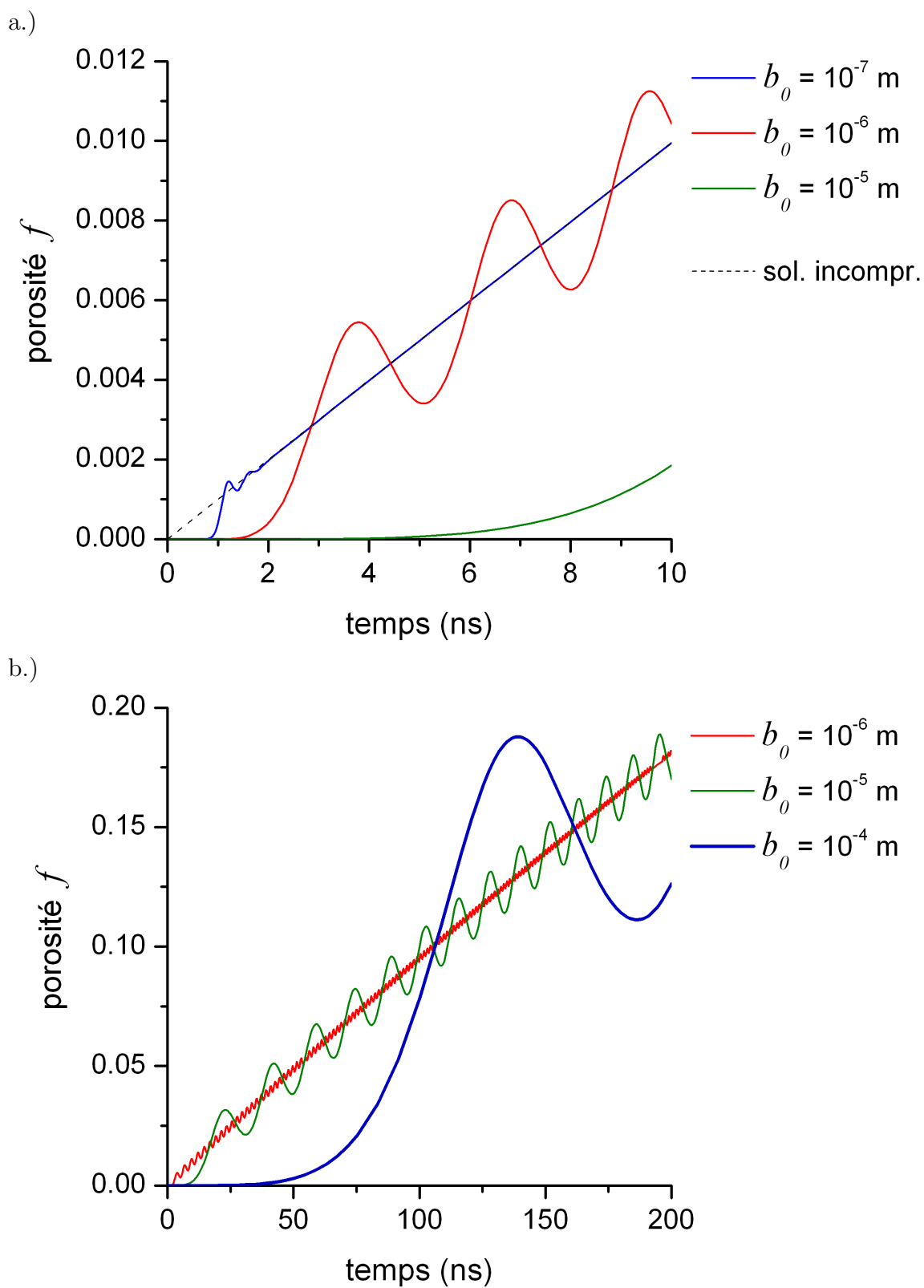
FIG. IV.4: Evolution de la porosité en fonction du rayon b_0 pour deux échelles de temps. Solutions du problème général (dynamique) du problème de sphère creuse pour la phase 1 et le cas de chargement No. 1.
