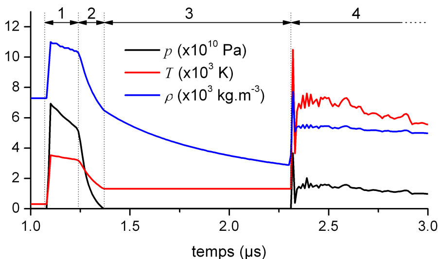
FIG. II.9: Histoire de la pression, de la température et de la masse volumique d'un élément dont la ruine par micro-écaillage est traitée numériquement par une pression nulle imposée
