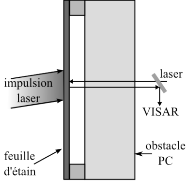
FIG. II.2: Représentation schématique des essais de choc laser avec mesure de la vitesse en face arrière de l'échantillon d'étain par interférométrie VISAR. L'obstacle en polycarbonate (PC) permet de collecter les éjectas, dont l'observation post-choc est présentée au paragraphe 3.2.
