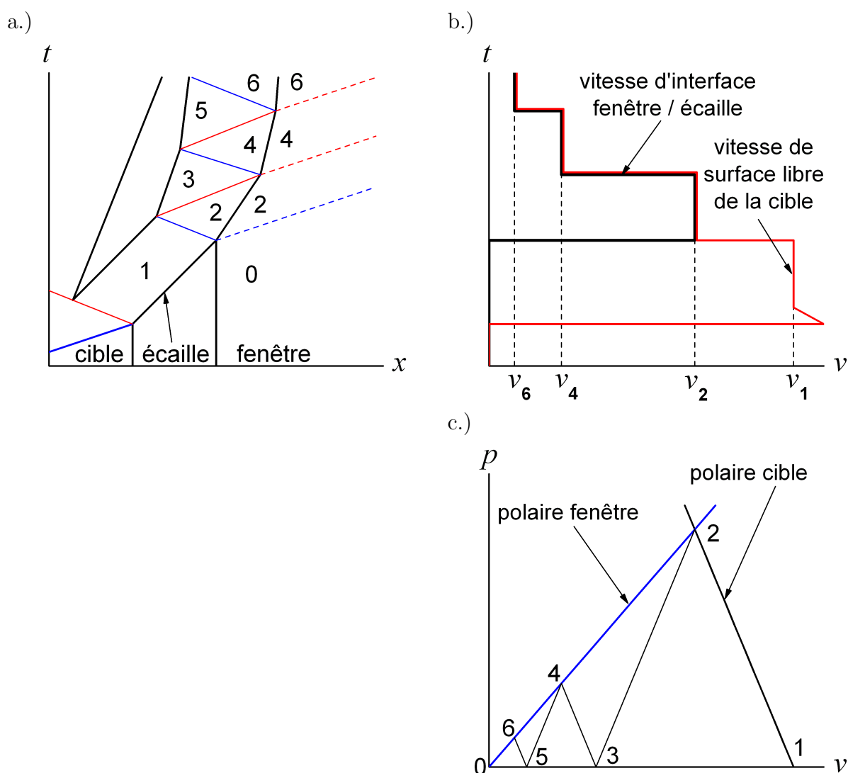
FIG. II.5: Illustration schématique de l'impact d'une écaïlle sur une fenêtre. (a) Diagramme x-t . (b) Histoire des vitesses de la surface libre de la cible et de la surface d'impact de la fenêtre. (c) Diagramme pression p - vitesse v représentant les états de l'écaïlle et de la fenêtre reportés sur le diagramme x-t .
