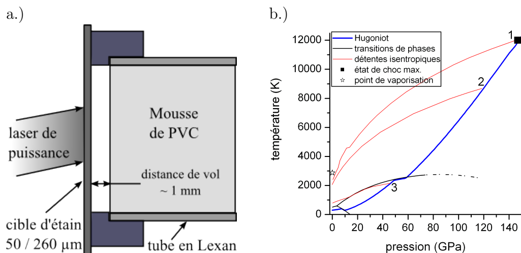
FIG. II.18: (a) Schéma de la configuration expérimentale. (b) États de choc, obtenus par simulation (avec les codes FILM et Hésione), atteints pendant les expériences de récupération par choc laser.
