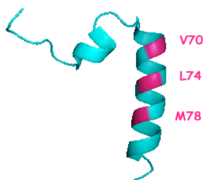
Hélice C terminale PscF : résidus 54 à 85
