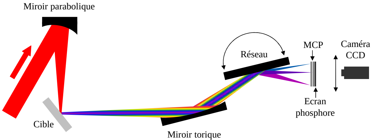
Fig. 7.1: Schéma du dispositif expérimental d'analyse spectrale.
