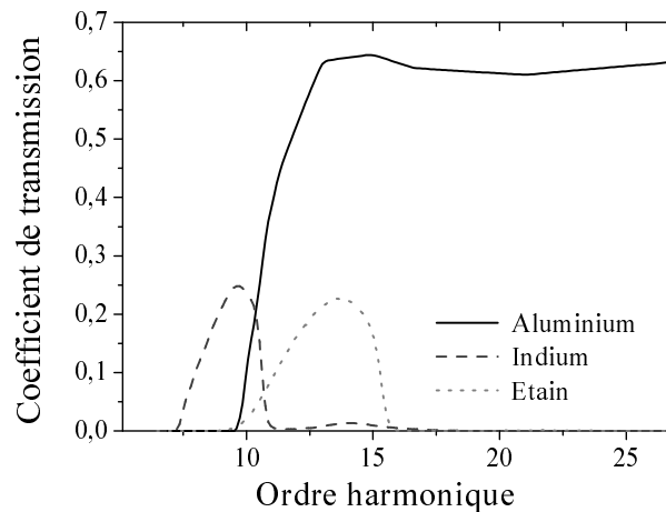
Fig. 7.4: Courbes de transmissions de 3 filtres métalliques. Ces 3 filtres sont des feuilles de 200\text{nm} d'aluminium, d'indium et d'étain, supposées non oxydées. Les données sont extraites de [110].
