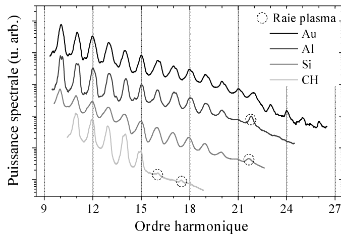
Fig. 8.1: Spectres d'harmoniques de sillage obtenus en utilisant des cibles faites de différents matériaux et un éclairement crête de 3 \times 10^{18} Wcm^{-2} . Les cercles indiquent les positions de différentes raies dues à l'émission incohérente du plasma. Afin de faciliter leur comparaison, les différents spectres ont été décalés selon l'axe des ordonnées
