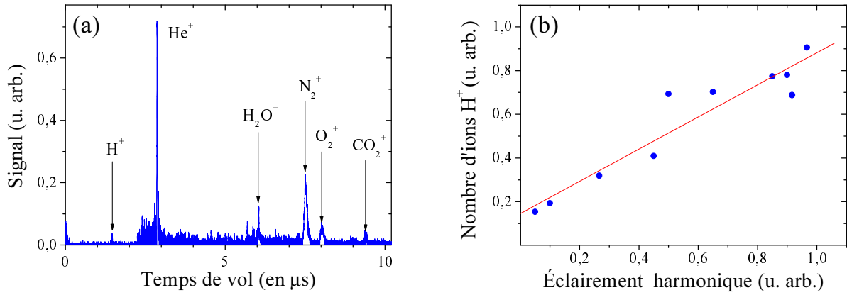
Fig. 10.3: (a) Spectre de temps de vols obtenu pour un filtre d'aluminium de 100nm . Les espèces ioniques associées aux différents pics sont indiquées sur la courbe. (b) Variation avec l'éclairement harmonique du nombre de protons détectés.
