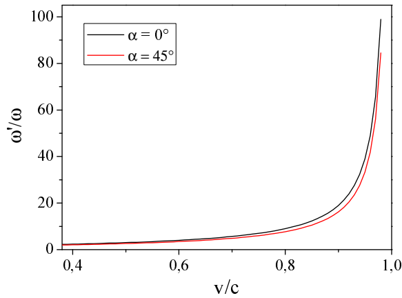
Fig. 6.2: Décalage Doppler calculé pour des angles d'incidence de 0^\circ et 45^\circ .
