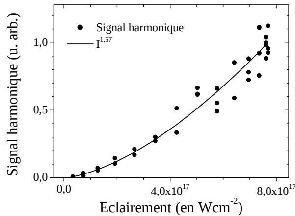
Fig. 8.4: Dépendance en éclairement du signal harmonique intégré spatialement en régime non relativiste ( 3 \times 10^{16} \text{ Wcm}^{-2} < I < 8 \times 10^{17} \text{ Wcm}^{-2} ). Le coefficient de corrélation de la courbe de tendance est de 0.99. Cette courbe a été obtenue en faisant varier la polarisation du laser et en intégrant le profil spatial des harmoniques transmises par un filtre d'étain (harmoniques 10 à 15).
