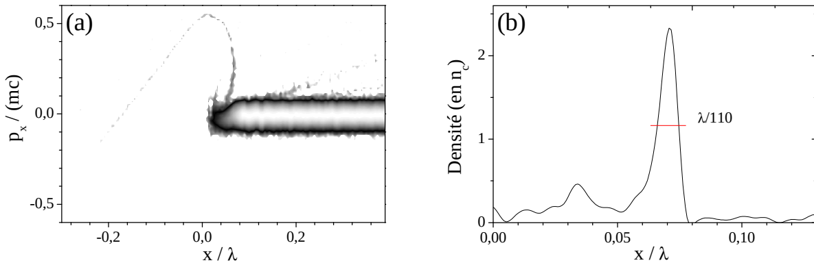
Fig. 5.5: Pic de densité électronique dans l'espace des phases. (a) Espace des phases (x, p_x) à t = 12.96T . On voit une concentration d'électrons énergétiques ( p_x \gtrsim 0.1mc ) en x \approx 0.07\lambda . (b) Somme sur p_x > 0.1mc de la densité électronique de l'espace des phases tracé en (a). Les électrons énergétiques sont concentrés sur une longueur inférieure à un centième de la longueur d'onde laser.
