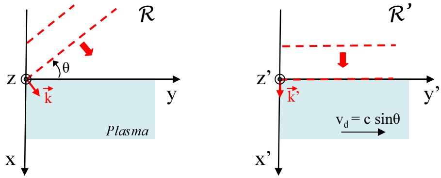
Fig. 3.6: Transformation de Lorentz. Dans le référentiel du laboratoire \mathcal{R} , le vecteur d'onde \vec{k} est dans le plan (x,y) où \vec{x} est un vecteur normal au plasma. Dans le référentiel mobile \mathcal{R}' , le plasma a une vitesse de dérive dans la direction y' et \vec{k}' est normal à la surface de la cible.
