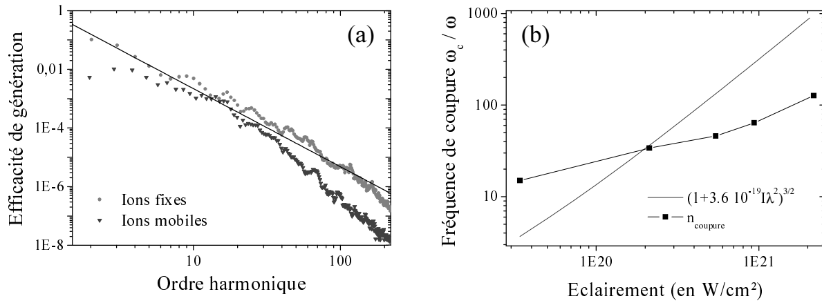
Fig. 6.13: Illustration des limites prédictives du modèle du miroir oscillant. (a) Comparaison des spectres obtenus avec des ions mobiles ou immobiles pour un éclairement I = 3.4 \times 10^{21} \text{ W cm}^{-2} et une longueur de gradient initiale de \lambda/25 . La ligne continue est la fonction \eta_{theo} = n^{-8/3} . (b) Variation de la fréquence de coupure avec l'éclairement dans le cas où les ions sont fixes. La ligne en traits pointillés correspond cette fois à la fonction (1 + 3.6 \times 10^{-19} I \lambda^2)^{3/2} .
