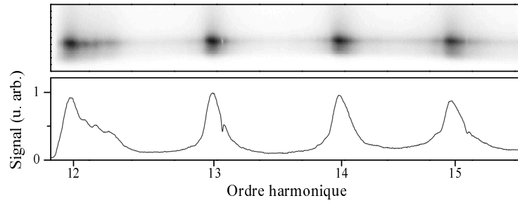
Fig. 5.26: Spectre expérimental des harmoniques 12 à 15 du laser UHI, générées en face arrière d'une feuille d'or de 50\text{nm} pour I = 3 \times 10^{18} \text{Wcm}^{-2} . Les données n'ont pas été corrigées de la transmission du spectromètre.
