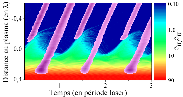
Fig. 4.2: Densité électronique et impulsions attosecondes pour I = 2.6 \times 10^{17} W cm^{-2} . La densité électronique est représentée, en échelle de couleur en fonction du temps et de la direction perpendiculaire à la surface du plasma. Pour obtenir le champ attoseconde en mauve, on a effectué en tout point de l'espace la transformée de Fourier du champ B_z , puis on a appliqué un filtre passe bande sélectionnant les harmoniques 5 à 9, et enfin on a fait une transformée de Fourier inverse.
