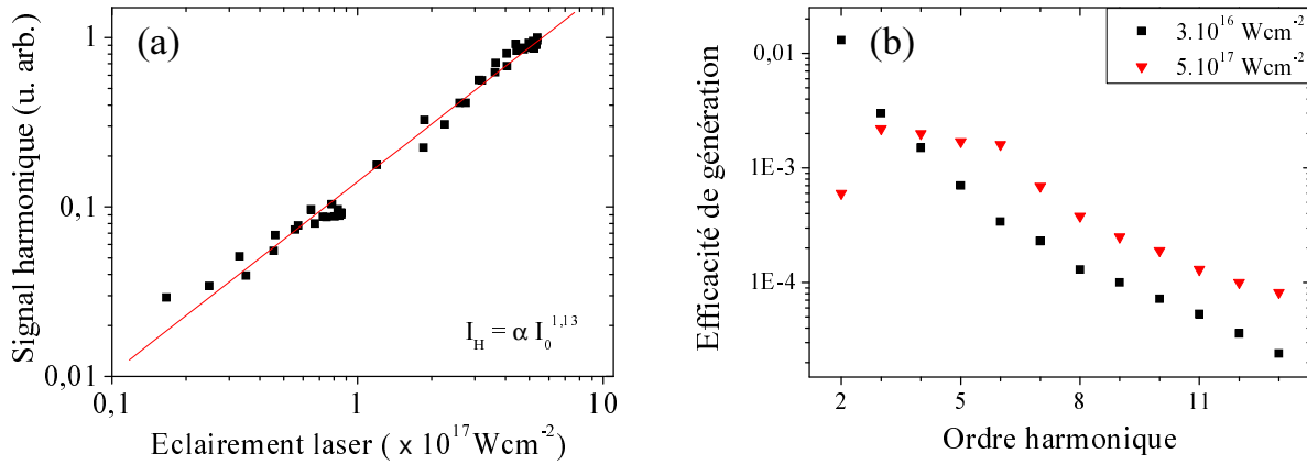
Fig. 5.23: Évolution du signal harmonique avec l'éclairement laser. (a) Deux séries de points sont représentées sur ce panneau, une qui permet d'observer l'évolution du signal jusqu'à 10^{17} \text{ Wcm}^{-2} , l'autre jusqu'à 6 \times 10^{17} \text{ Wcm}^{-2} . Chaque série a été obtenue en mesurant la variation du signal intégré sur les harmoniques 4 à 15, au cours d'une simulation où l'éclairement laser varie dans le temps comme un sinus au carré. La courbe de tendance calculée en utilisant l'ensemble des points montre que le signal harmonique augmente avec le signal incident à la puissance 1.13 \pm 0.02 . (b) Spectres obtenus pour des éclairements de 3 \times 10^{16} \text{ Wcm}^{-2} (carrés noirs) 5 \times 10^{17} \text{ Wcm}^{-2} (triangles rouges). Afin d'alléger la figure, seule l'efficacité de génération crête est représentée.
