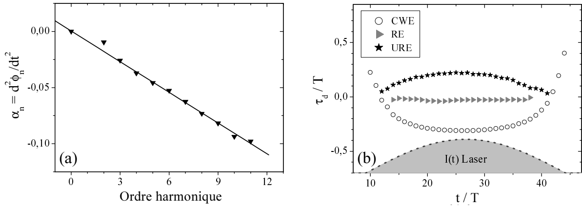
Fig. 9.1: Mise en évidence numérique de la dérive de fréquence des harmoniques individuelles, dans le cas où les ions sont immobiles. (a) Évolution du paramètre \alpha_n = d^2 \Phi_n / dt^2 avec l'ordre harmonique n . (b) Variations de \tau_d(k) = t_d(k) - (t_0 + k) , dans le cas de l'émission cohérente de sillage (CWE), dans celui de l'émission relativiste (RE) et dans celui de l'émission ultra-relativiste I \gg 10^{18} \text{ W cm}^{-2} (URE). La valeur de t_0 est arbitraire et change d'une simulation à l'autre, on ne peut donc comparer que les variations de \tau_d .
