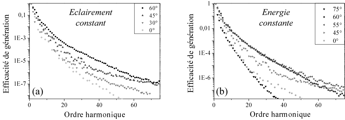
Fig. 6.12: Influence de l'angle d'incidence. (a) Variation de l'angle entre 0° et 60°, à éclairement constant, I = 3.5 \times 10^{19} \text{ W cm}^{-2} . (b) Variation de l'angle entre 0° et 75° à énergie par impulsion constante, I = 3.5(\cos \theta / \cos 45) \times 10^{19} \text{ W cm}^{-2} .
