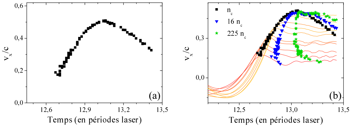
Fig. 5.3: (a) Vitesse de retour dans le plasma des électrons de Brunel v_r(t) , en fonction du temps. Cette vitesse est celle des particules de la figure 5.2, à l'instant où elles retransversent la surface critique ( x = 0 ). (b) Évolution de la vitesse de 10 électrons dans le gradient de densité. Les temps de passage à n_c , 16n_c et 225n_c sont représentés par des points de différentes formes.
