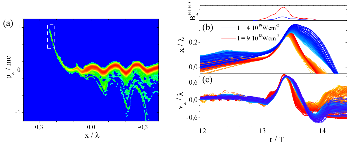
Fig. 9.11: Trajectories des électrons de Brunel relativistes pour deux éclairements différents. (a) Espace des phases (x, p_x) . En x \approx 0.35 , on observe le pic de densité qui est associé aux électrons qui émettent les impulsions relativistes. Le cadre en traits discontinus délimite le domaine de l'espace des phases dans lequel nous avons sélectionné quelques électrons parmi ceux qui forment ce pic. (b) Trajectoires (x, t) des particules sélectionnées en (a). Les deux familles de courbes sont associées à deux éclairements différents. (c) Évolution en fonction du temps de la vitesse des électrons dans la direction spéculaire. Sur le panneau supérieur, on observe les enveloppes des impulsions attosecondes émises dans les deux cas.
