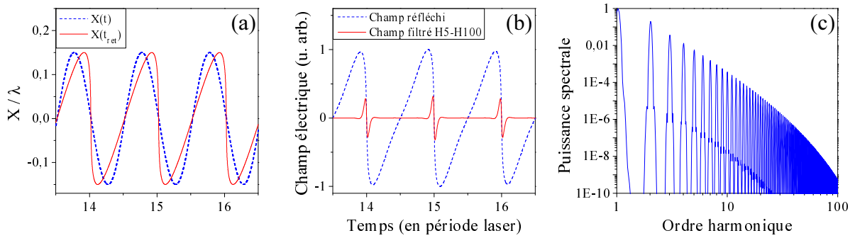
Fig. 6.3: Mouvement de la surface et champ réfléchi. (a) Trajectoires du point de réflexion X(t) = 0,15 \sin(\omega_0 t) et du même point pris aux temps retardés t_{ret} . (b) Champ réfléchi et champ réfléchi filtré entre les harmoniques 5 à 100 (train d'impulsions attosecondes). (c) Spectre du champ réfléchi.
