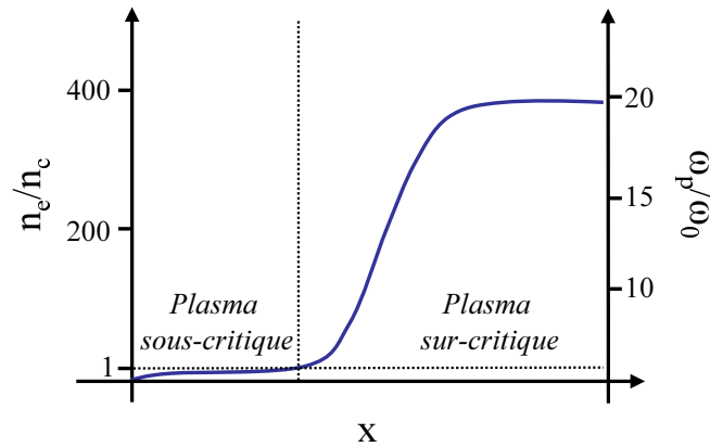
Fig. 1.1: Profil de densité schématique d'un plasma « réaliste ».
