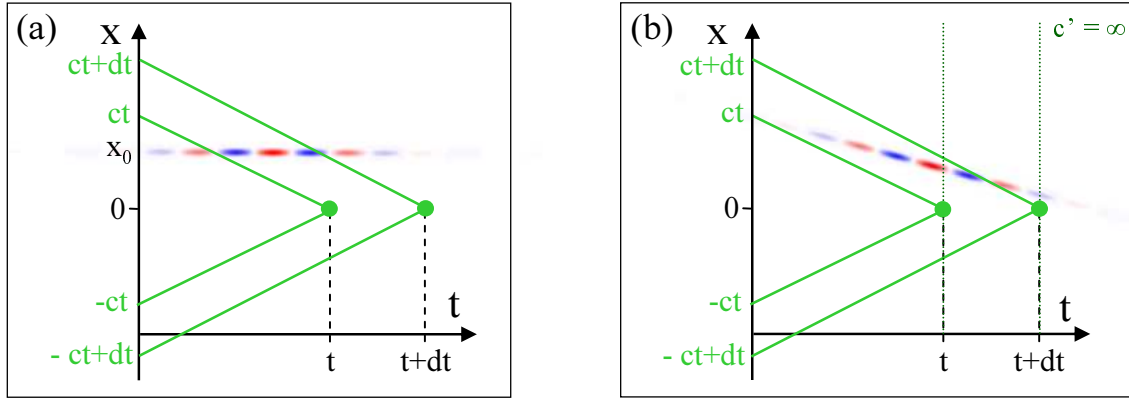
Fig. 1.8: Illustration du calcul de l'intégrale des courants retardés en 1D . En (a) une source harmonique placée en x = x_0 émet pendant 3 périodes optiques. Le courant transverse associé à cette source est tracé en échelle de couleur. En (b) cette source est animée d'une vitesse de l'ordre de c . Les droites en traits continus représentent les chemins d'intégration en (0, t) et (0, t + dt) , celles en pointillés correspondent au cas où on considère que l'information se déplace à vitesse infinie.
