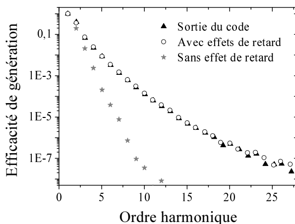
Fig. 6.6: Spectres calculés à partir du courant transverse avec et sans effets de retard. Afin de rendre la figure plus lisible, seuls les points aux fréquences harmoniques sont représentés. La courbe qui tient compte des effets de retard (cercles blancs), reproduit parfaitement le spectre calculé directement à partir du champ E_y fourni par le code (triangles noirs). Lorsque ces effets sont supprimés (étoiles grises), on ne distingue plus d'harmonique au delà de l'ordre 10 (le niveau du bruit numérique est de l'ordre de 5 \times 10^{-9} ).
