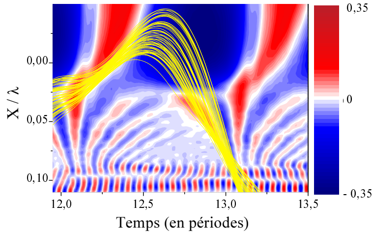
Fig. 5.17: Excitation d'oscillations plasmas par le pic de densité formé par les électrons de Brunel. On observe les trajectoires des électrons énergétiques qui forment des pics de densité, tracées sur une carte de champ E_x . On voit que ces électrons excitent des oscillations plasmas dans le gradient de densité pour t \gtrsim 13T (les oscillations entre t \approx 12T et t \approx 13T ont été excitées par les électrons de Brunel revenus lors du cycle laser précédent).
