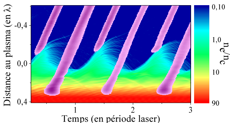
Fig. 4.2: Densité électronique et impulsions attosecondes pour I = 2.6 \times 10^{17} \text{Wcm}^{-2} . La densité électronique est représentée, en échelle de couleur en fonction du temps et de la direction perpendiculaire à la surface du plasma. Pour obtenir le champ attoseconde en mauve, on a effectué en tout point de l'espace la transformée de Fourier du champ B_z , puis on a appliqué un filtre passe bande sélectionnant les harmoniques 5 à 9, et enfin on a fait une transformée de Fourier inverse.
