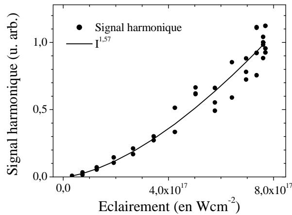
Fig. 8.4: Dépendance en éclairement du signal harmonique intégré spatialement en régime non relativiste ( 3 \times 10^{16} Wcm^{-2} < I < 8 \times 10^{17} Wcm^{-2} ). Le coefficient de corrélation de la courbe de tendance est de 0.99. Cette courbe a été obtenue en faisant varier la polarisation du laser et en intégrant le profil spatial des harmoniques transmises par un filtre d'étain (harmoniques 10 à 15).
