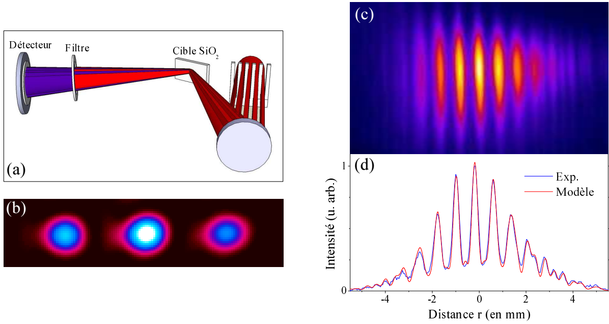
Fig. 9.13: Interférences à trois sources harmoniques. (a) Schéma expérimental simplifié (les lames de silice traitées anti-reflet ont été omises). (b) Image de la distribution d'intensité au foyer. (c) Figures d'interférences obtenues au niveau des galettes à 38cm de la source, pour une superposition des harmoniques 8 à 10 (filtre d'indium). Le faisceau laser est ouvert à f/17 . (d) Profils des franges. La courbe expérimentale a été extraite de (c), la courbe théorique a été obtenue pour \Delta\Phi_n = 0.23n \text{ rad} .
