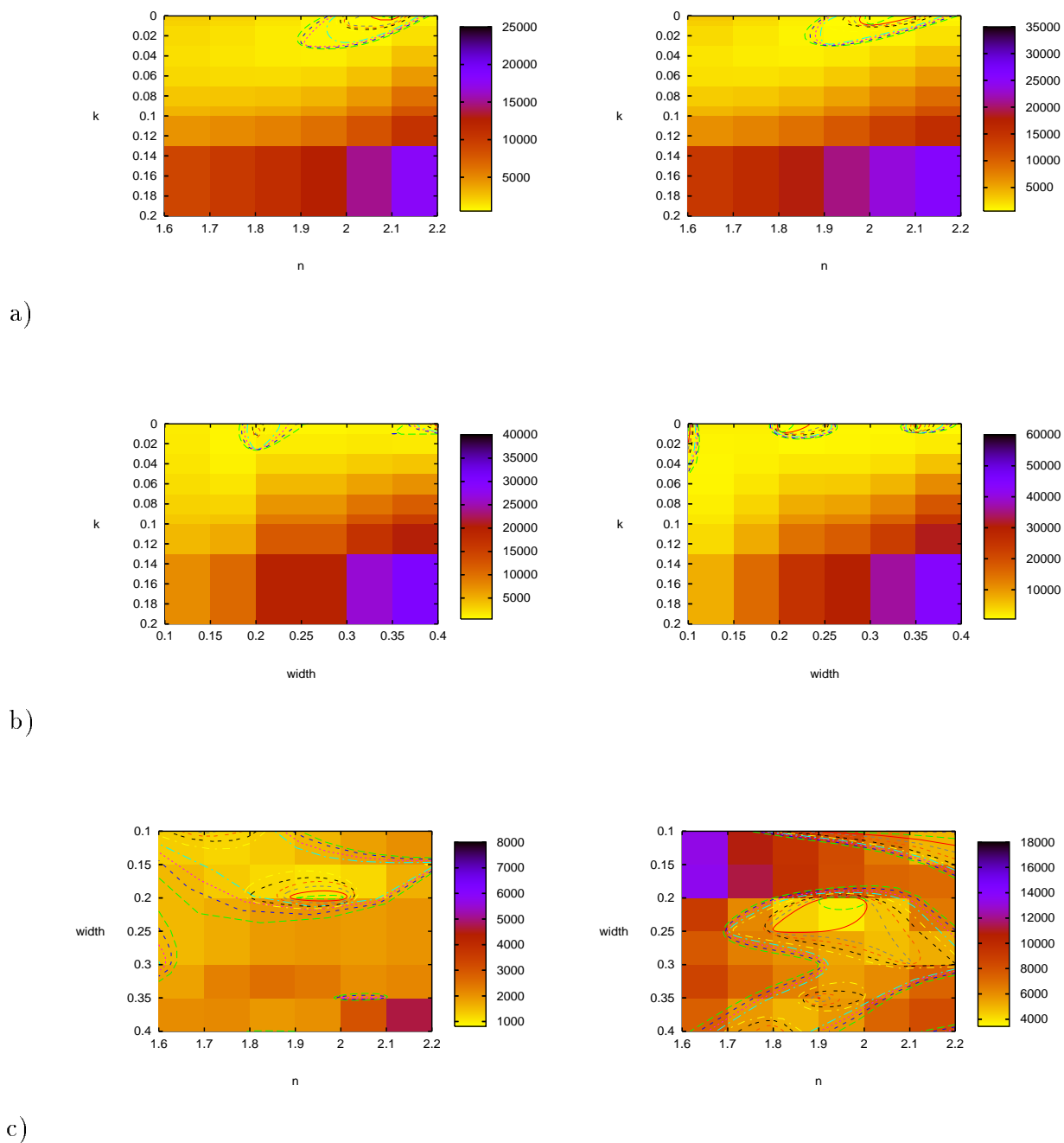
FIG. 3.11 – Cartes de \chi^2 calculées pour les billes recouvertes d'un manteau de graphite en fonction de deux des trois paramètres du manteau. A gauche, calculs pour les données à 632,8 nm ; à droite, calculs pour les données à 543,5 nm. a) carte en fonction de la partie réelle et imaginaire de l'indice optique (épaisseur fixée à 200 nm) b) carte en fonction de la partie imaginaire de l'indice optique et de l'épaisseur du manteau (partie réelle fixée à 2) c) carte en fonction de la partie réelle de l'indice optique et de l'épaisseur du manteau (partie imaginaire fixée à 0,03)
