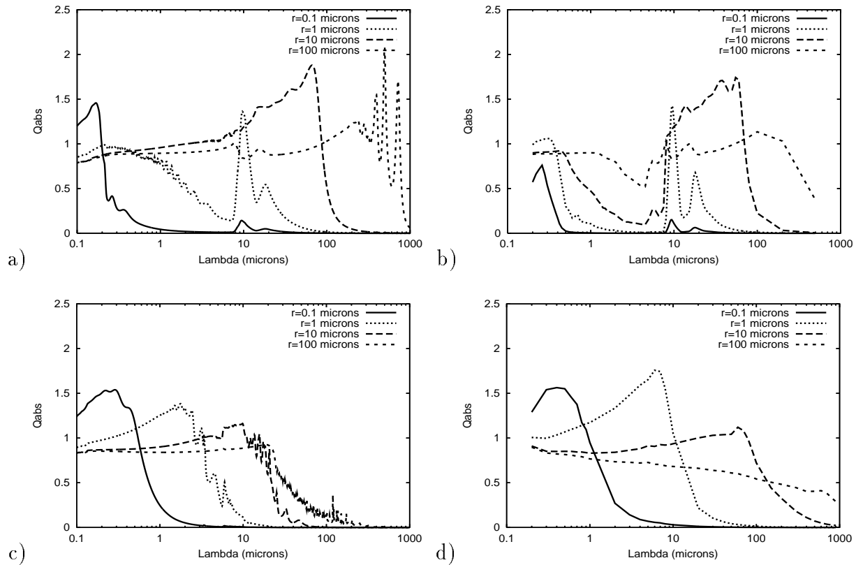
FIG. 5.10 – Comparaison des coefficients d'absorption, Q_{abs} , pour des sphères en fonction de la longueur d'onde et du rayon effectif des particules. Les matériaux considérés correspondent respectivement à a) silicates interstellaires de Draine et Lee (1984), b) pyroxène amorphe de Dorschner et al. (1995), c) matériaux organiques de Li et Greenberg (1997) et d) carbone amorphe de Edoh (1983)
