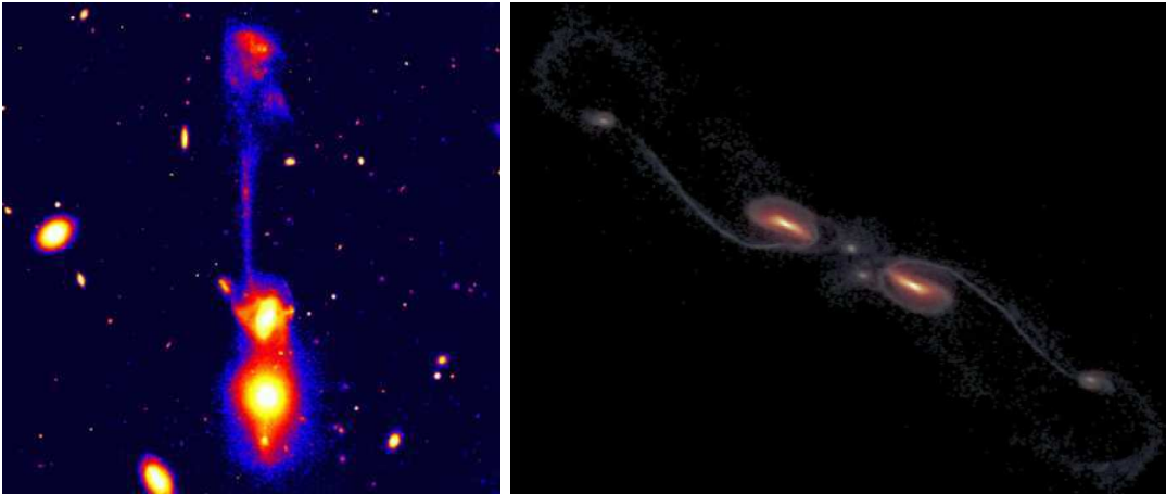
FIGURE 4.6 – Gauche : Observation de ARP 105, une naine de marée s’est formée à l’extrémité de la queue de marée. Droite : Simulation de formation de galaxies naines de marée en gravitation modifiée, le potentiel MOND créé par les galaxies est suffisamment important pour retenir et accumuler le gaz dans les naines.
