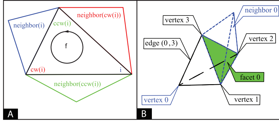
FIG. 3.1: Les conventions des triangulations de CGAL en dimension 2 (A) et en dimension 3 (B) : Les sommets sont numérotés dans l'ordre direct, et chaque voisin est opposé au sommet du même indice[CGAL 07]. la fonction ccw(i) retourne le numéro suivant de i dans le sens direct de l'orientation, et la fonction cw(i) retourne le numéro suivant dans le sens opposé.
