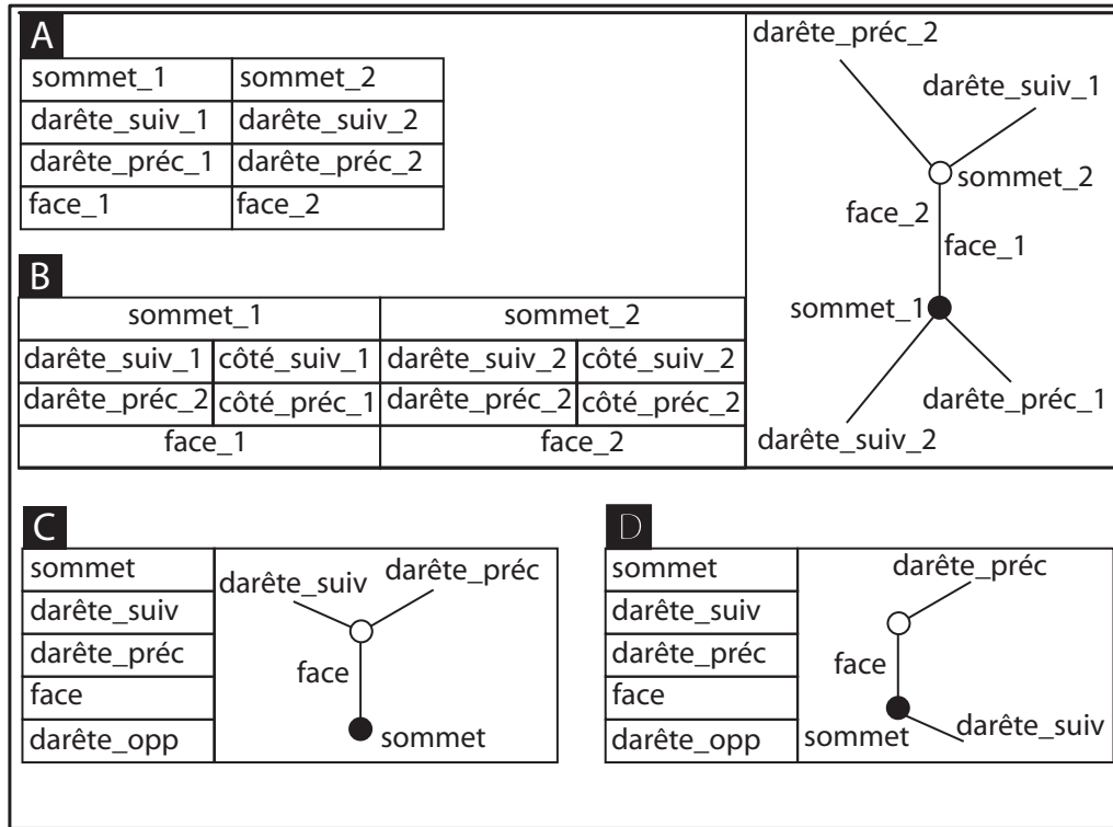
FIG. 2.4: La modélisation de l'arête dans les structures de données à base d'arêtes proposées par Kevin Weiler[Weil 85] : (A) La structure de l' arête ailée de Baugmart[Baum 75] (B) La version modifiée de l' arête ailée en ajoutant un entier à la référence de l'arête indiquant de quel côté de l'arête on est arrivé (C) La structure à base de demi-arêtes Sommet-Arête où la demi-arête est identifiée par son sommet de référence (D) La structure à base de demi-arêtes Face-Arête où la demi-arête est identifiée par sa face de référence.
