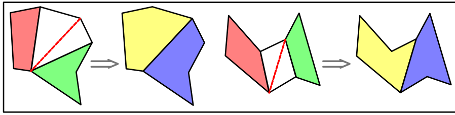
FIG. 4.9: Si deux quadrangles sont voisins à un autre quadrangle, et si ces deux quadrangles sont incidents à un sommet de la diagonale, les trois quadrangles peuvent être convertis en deux pentagones.
