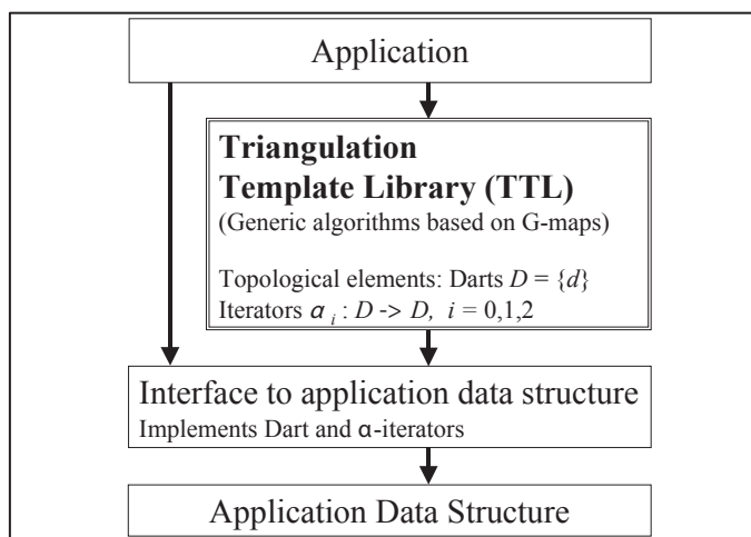
FIG. 2.8: La conception de la Template Triangulations Library proposée par Øyvind Hjellevind [Hjel 00].
