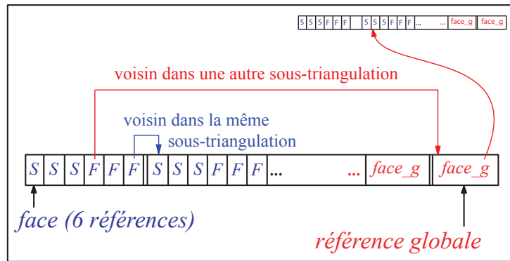
FIG. 5.1: Un seul tableau de taille 2m triangles suffit pour représenter à la fois les faces de la sous-triangulation, en partant de la gauche ; et les références externes de cette même sous-triangulation vers les autres sous-triangulations en partant de la droite.
