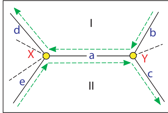
FIG. 2.1: La structure de l'arête ailée : L'objet de base est l'arête. Pour représenter l'arête a , ces informations sont utiles : (i) Les sommets de cette arête X et Y (ii) Les deux faces incidentes I et II (iii) Les prédécesseurs et les successeurs pour cette arête dans les deux faces : b , c , d , et e .
