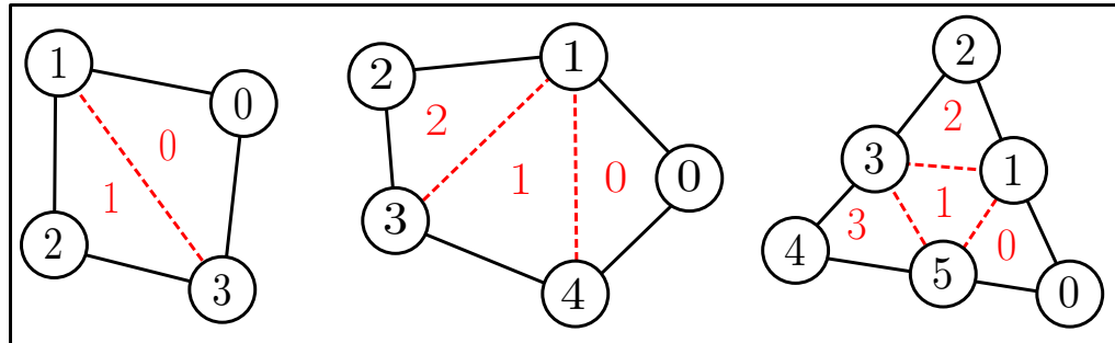
FIG. 4.3: Les diagonales des petites micro-triangulations peuvent être codées implicitement en fixant un ordre conventionnel relatif à la diagonale. La diagonale du quadrangle relie les sommets 1 et 3. Celles du pentagone relient les sommets 1 à 3, et 1 à 4. Et les diagonales de l'hexagone relient les sommets 1, 3 et 5. Les triangles internes peuvent aussi être implicitement numérotés sans ambiguïté.
