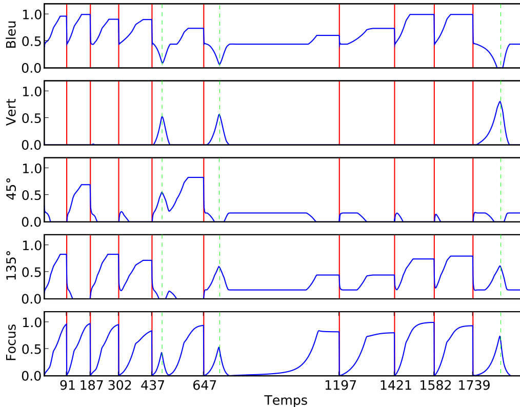
FIG. 4.15 – Les quatre premiers graphiques représentent l'activité des quatre cellules des cartes FEATURE MAPS respectivement sélectives aux attributs bleu , vert , 45° et 135° , au cours du temps. Les barres verticales rouges représentent les instants d'exécution des saccades et les barres vertes en pointillés représentent les instants de déploiement covert de l'attention. Ces quatre graphiques accompagnés du dernier graphique représentant l'évolution temporelle de l'activité moyenne normalisée dans la carte FOCUS fournissent de bons indicateurs pour estimer le comportement du mécanisme, à la fois sur le fait d'avoir sélectionné une cible et sur la nature de la cible sélectionnée.
