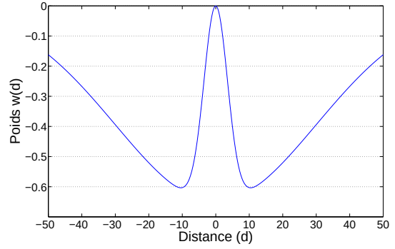
FIG. 2.16 – a) Architecture du système. La carte INPUT excite la carte FOCUS dont les unités ont des projections latérales en différence de gaussiennes. b) Les poids des projections, définis par les équations 2.10, sont uniquement inhibiteurs.
