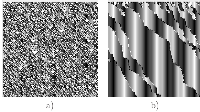
FIG. 2.6 – a) Évolution de la règle 30 en évaluation synchrone b) Lorsqu'on utilise un schéma d'évaluation asynchrone, le comportement est complètement différent.
