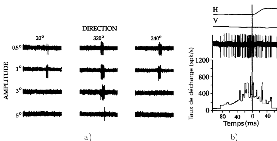
FIG. 3.9 – a) Certaines cellules dont l'activité est corrélée à l'exécution d'une saccade déchargent une bouffée d'activité peu de temps avant un mouvement d'une amplitude et d'une direction données. b) D'autres cellules motrices ont une activité qui croît progressivement jusqu'à l'exécution d'une saccade. Adapté de [Sparks et al., 1976]
