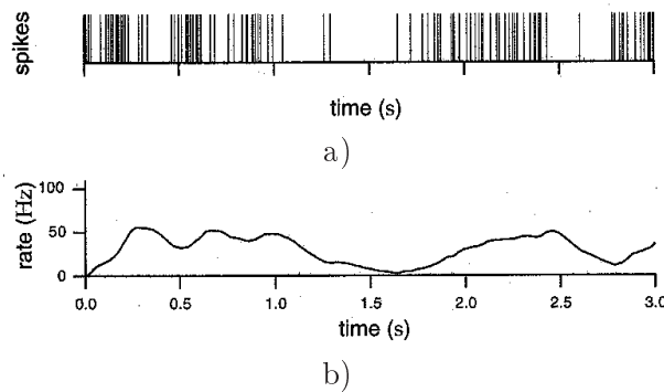
FIG. 2.2 – a) Enregistrement d'un train de spikes émis par un neurone du singe. Les spikes correspondent à des croissances rapides et brutales du potentiel membranaire du neurone, qui se propagent efficacement le long de l'axone. b) Une façon commode de représenter les trains de spikes est de calculer la fréquence de décharge d'un neurone, évaluée par le nombre de spikes émis par seconde. Adapté de [Dayan et Abbott, 2001]
