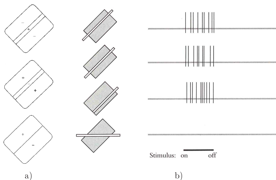
FIG. 3.14 – a) Trois exemples de champ récepteur d'une cellule simple. La cellule décharge d'autant plus que la région excitatrice (+) est illuminée et que la région inhibitrice (-) ne l'est pas b) Pour une cellule complexe, une stimulation longue et fine (rectangle blanc) évoque une réponse forte (le diagramme à droite représente la décharge d'une cellule en fonction de la présence ou non de la stimulation), quelle que soit sa position dans le champ récepteur (rectangle gris) et évoque une réponse faible ou nulle dès lors qu'elle a une orientation non optimale. Adapté de [Hubel, 1988]
