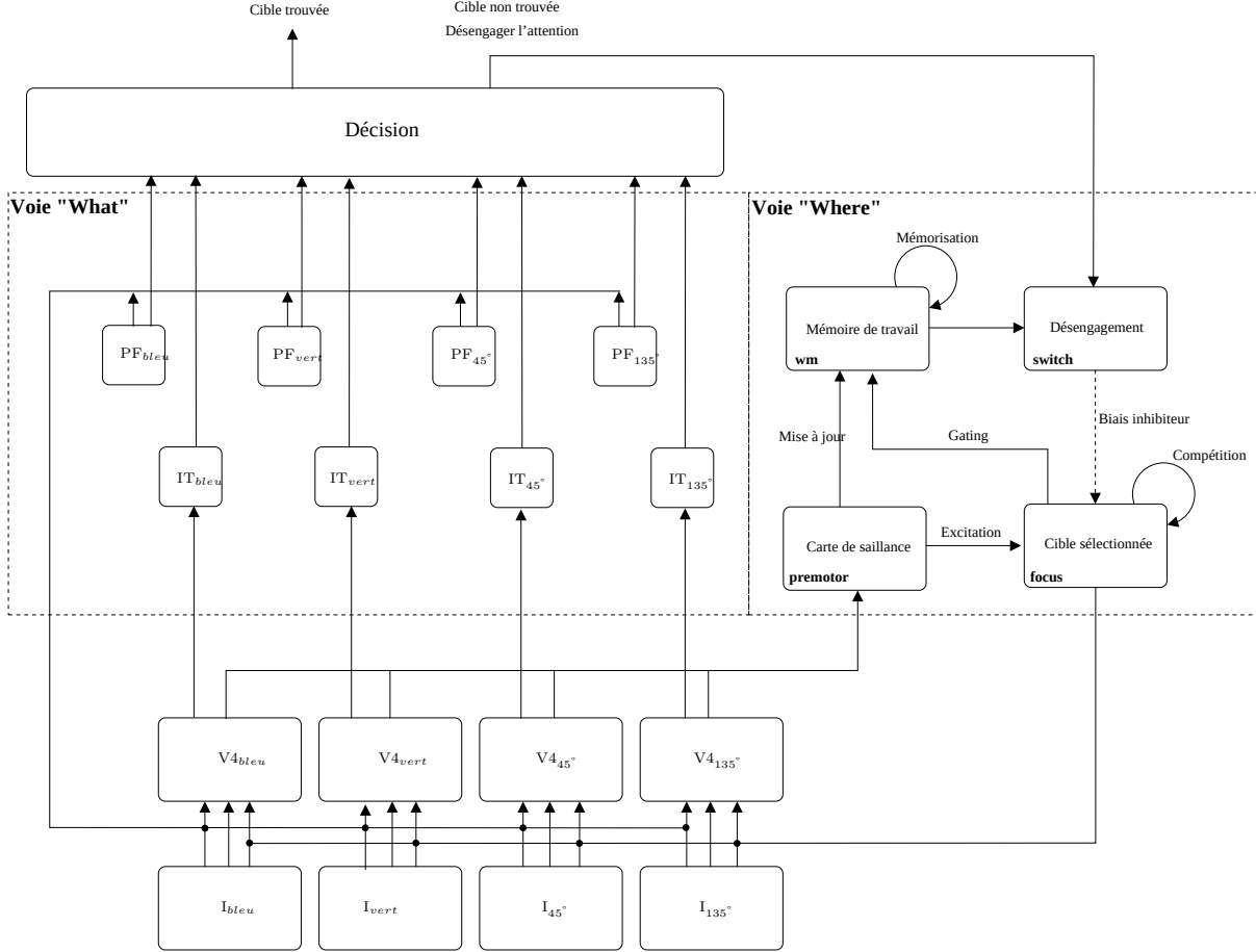
FIG. 2.22 – Mécanisme de déploiement covert de l'attention visuelle. A la voie "Where" détaillée dans les paragraphes précédents, on adjoint des mécanismes qui permettent de moduler la carte de saillance PREMOTOR en fonction des attributs visuels recherchés. L'entrée visuelle est filtrée selon plusieurs dimensions. Le résultat de ces filtres définit l'activité des unités des cartes I_* . Ces cartes excitent les cartes V4_* qui servent de niveau intermédiaire dans le système. Ces cartes ont des afférences de l'entrée visuelle, des unités représentant les attributs à rechercher PF_* ainsi que de la carte de sélection spatiale FOCUS. Toutes les équations d'évolution des unités ainsi que les paramètres du modèle sont disponibles dans les annexes A.1 et A.2
