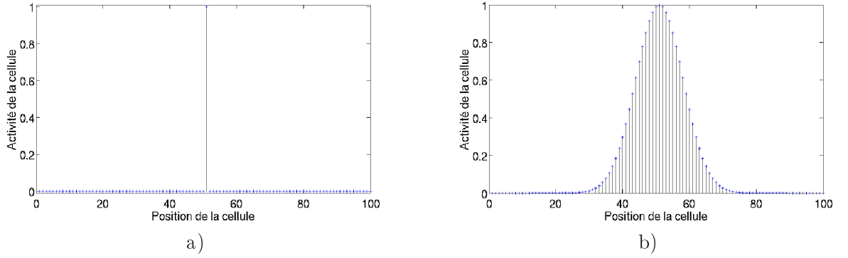
FIG. 2.7 – a) Réponse de la population localisée encodant la valeur 1.5 avec une très petite variance \sigma = 10^{-11} . Dans un codage localisé, au plus une cellule est active lorsque la population encode une valeur. Ici, seule la cellule 50 est active. b) Réponse de la population distribuée encodant la valeur 1.5 avec une variance plus grande \sigma = 0.1 . La variance est définie dans l'espace d'entrée. Puisque l'espace encodé est [1.0; 2.0] , elle correspond avec une variance de 0.1N = 10 cellules dans l'espace neuronal.
