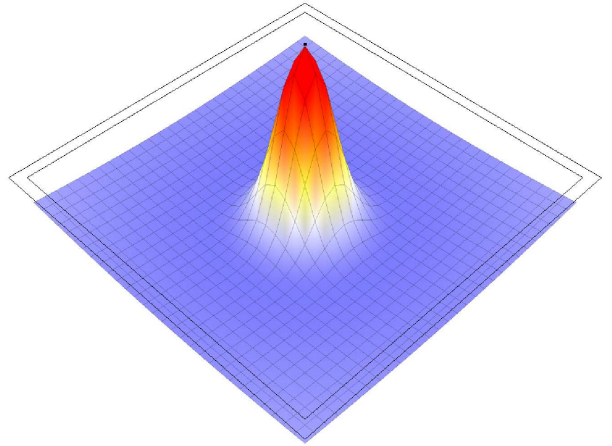
FIG. C.1 – Le script permet de créer une carte de 30 \times 30 cellules. Les connexions latérales dans la carte sont définis par une différence gaussienne, illustrée à droite.
