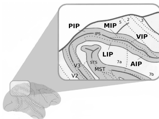
FIG. 3.17 – Illustration des principales aires visuelles avoisinants le sillon intrapariétal. On trouvera plus de détails sur ces aires dans le texte. VIP : Ventral Intraparietal area ; MIP : Medial Intraparietal area ; AIP : Anterior Intraparietal area. PIP : Posterior Intraparietal area ; LIP : Lateral Intraparietal area. Adapté de [Cavada, 2001]
