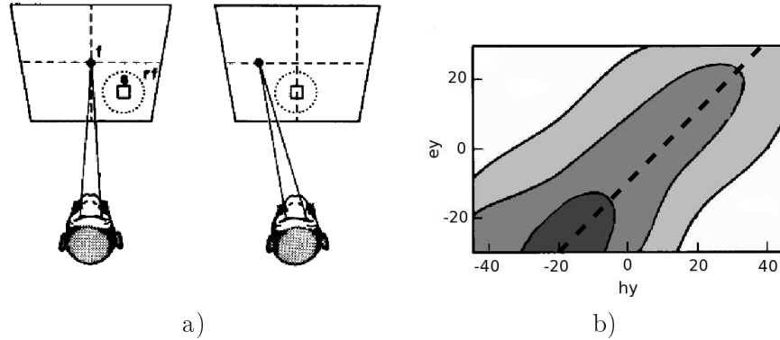
FIG. 3.18 – a) Pour observer les propriétés de champ de gains, on présente à un singe, qui maintient son regard sur le point de fixation f , un stimulus en périphérie. Pendant cette tâche, l'activité des neurones de 7a ou LIP est enregistrée. b) Lorsqu'on trace l'activité (en niveau de gris, du blanc au noir pour des activités croissantes) des cellules enregistrées en fonction de la position verticale de l'œil ey et de la position verticale de la cible par rapport à la tête hy , on observe deux propriétés : les champs récepteurs sont rétinotopiques (il y a une région de l'espace visuel, fixe par rapport à l'œil, dans laquelle les cellules déchargent maximale-ment) et leur activité est modulée par la position de l'œil. Adapté de [Andersen et al., 1985]
