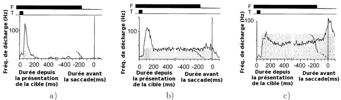
FIG. 3.23 – Quelques exemples d'activités de cellules de FEF. a) Une cellule visuelle phasique qui décharge à la présentation d'un stimulus dans son champ récepteur puis est silencieuse b) Une cellule visuelle tonique qui décharge une bouffée d'activité à la présentation d'un stimulus dans son champ récepteur suivie d'une décharge tonique pendant le délai précédant l'exécution d'une saccade vers cette cible mémorisée c) Une cellule dont l'activité croît significativement à l'exécution d'une saccade vers une cible mémorisée. Adapté de [Hanes et al., 1998]
