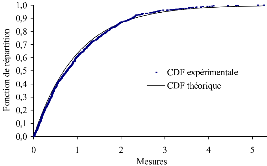
FIG. 2.1: Exemple de fonctions de répartition théorique et expérimentale.
