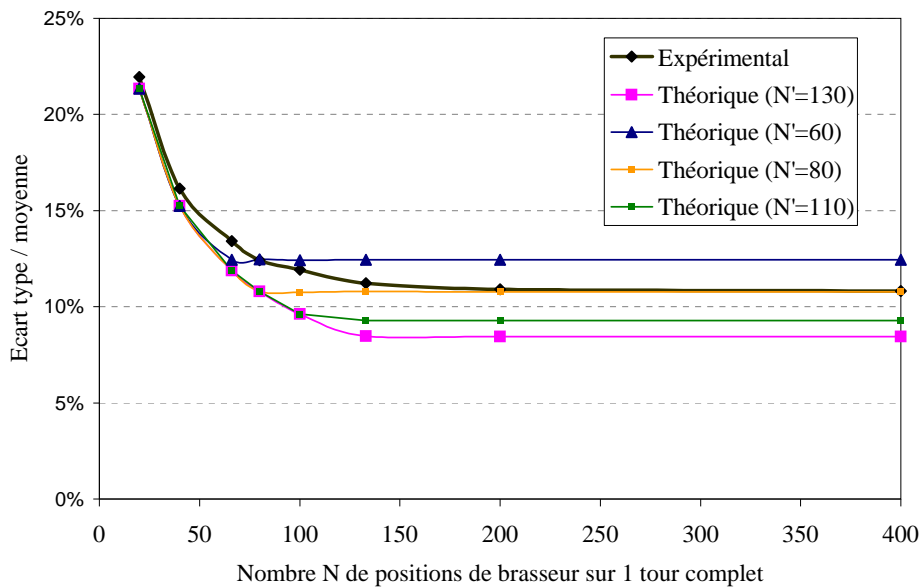
FIG. 7.14: Comparaison des ratios \sigma_{\mu_x} / \mu_x théoriques et expérimentaux dans le cas d'un brassage mécanique, en fonction de plusieurs évolutions théoriques selon le nombre N' de positions de brasseur indépendantes parmi N = 400 positions sur un tour complet.
