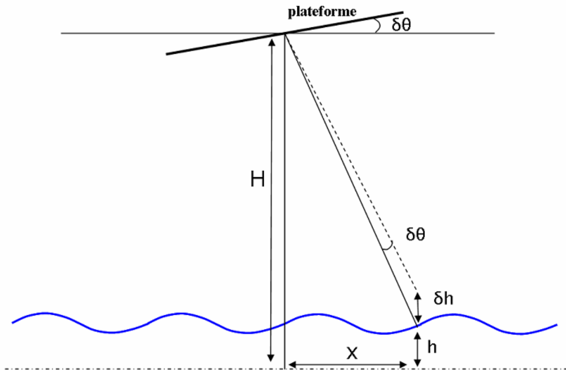
Figure B.4 : Erreurs de mesure dues au roulis \delta\theta de la plateforme
