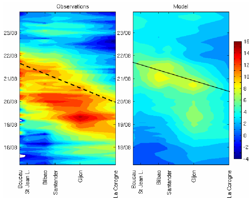
Figure G.10 : Zoom de la Figure G.9 sur la cote nord espagnole autour du 19 août.
