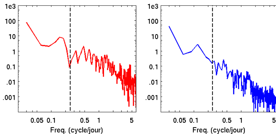
Figure G.13 : Spectres associées à l'écart type d'ensemble en élévation de surface pour le Point 1 (gauche) et le Point 2 (droite). Abscisse : fréquence (cycle/jour), ordonnée : puissance ( cm^2 ). Les tirets verticaux représentent la limite de représentativité de la simulation de référence avec sorties moyennées sur 2 jours (0.25 cycle/jour).
