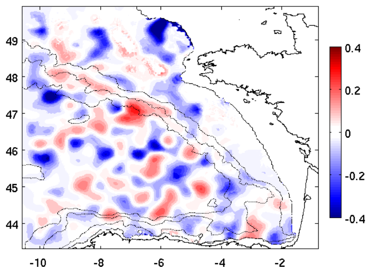
Figure F.7 : différence de température ( ^{\circ}\text{C} ) à 100m entre le champ de référence et le champ perturbé.
