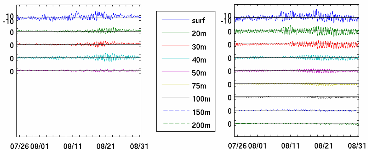
Figure G.7 : Séries temporelles de courant zonal à différentes profondeurs ( cm.s^{-1} ) au Point 1 (gauche) et au Point 2 (droite).
