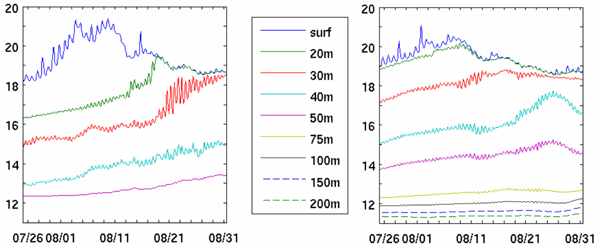
Figure G.5 : Séries temporelles de la température ( ^{\circ}\text{C} ) au Point 1 (gauche) et au Point 2 (droite) pour différentes profondeurs et en surface.
