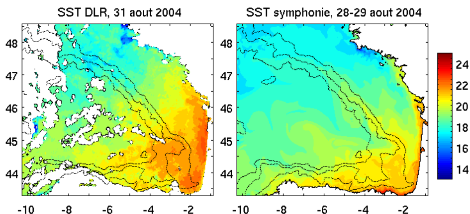
Figure D.45 : SST ( ^{\circ}\text{C} ) vues par AVHRR (gauche) et par le modèle Symphonie (droite). Les lignes isobathes 200, 2000 et 4000m sont notées. Elles ne sont qu'indicatives pour les données DLR en raison d'approximation dans la projection horizontale.
