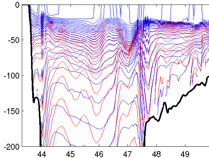
Figure F.6 : Niveaux verticaux (1 sur 3, m) en fonction de la latitude à 6.9^{\circ}\text{O} pour la grille z(\sigma_{\rho}) de référence (bleu) et la grille perturbée (rouge)
