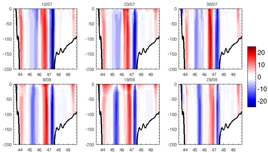
Figure D.36 : évolution temporelle du courant zonal ( cm.s^{-1} ) dans les 200 premiers mètres à 6.7^{\circ}O
