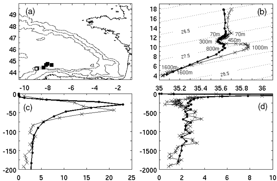
Figure D.54 : (a) localisation des relevés du flotteur Argo (carrés) sur la zone d'étude, (b) diagramme \theta -S ( ^{\circ}\text{C} , psu) relatif à la mesure effectuée sur le carré blanc en (a), le 12 juillet 2004, avec profondeurs des masses d'eau caractéristiques, pour le modèle (trait épais avec ronds) et les observations (trait fin avec croix), avec valeurs constantes de l'anomalie de densité potentielle \sigma_0 (tous les 1 \text{ g.m}^{-3} , tirets), (c) fréquence de Brunt-Väisälä ( 10^{-3} \text{ s}^{-1} ) pour le modèle (trait épais avec ronds) et les observations (trait fin avec croix), dans les 200 premiers mètres, (d) comme (c) mais dans les 2000 premiers mètres.
