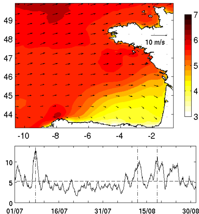
Figure D.12 : (haut) Carte de la norme moyenne du vent à 10m ( m.s^{-1} ) du modèle Aladin pour juillet et août 2004, avec vecteurs associés. (bas) Série temporelle de la moyenne spatiale instantanée de la norme de vent à 10m ( m.s^{-1} ) au cours de la simulation (trait plein), avec la moyenne temporelle associée ( 5.3 m.s^{-1} , en tirets). Les 3 épisodes dépressionnaires sont notés (traits mixtes verticaux).
