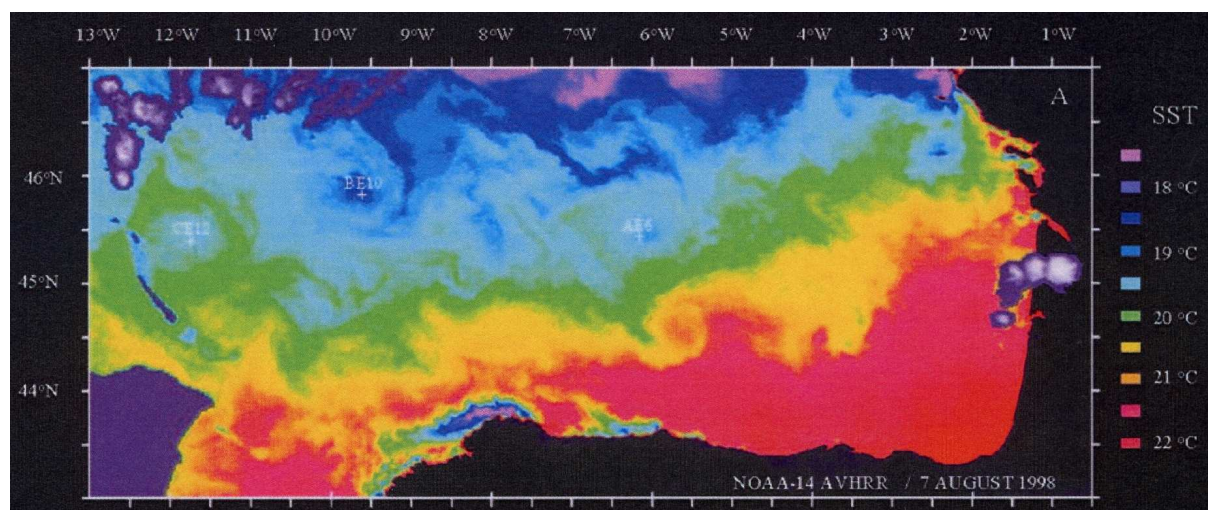
Figure D.8 : (haut) mécanisme simplifié de l'upwelling (Image NOAA), (bas) température de surface du Golfe de Gascogne vu par AVHRR le 7 août 1998.
