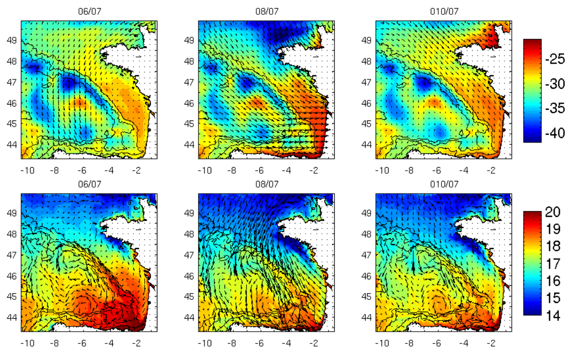
Figure D.37 : Haut : élévation de surface (cm) et stress de vent ( N.m^{-2} , flèche de référence 0.1 N.m^{-2} ). Bas : SST ( ^{\circ}C ) et courant de surface ( cm.s^{-1} , flèche de référence 0.1 cm.s^{-1} ). De gauche à droite : sortie du modèle précédent l'épisode, durant l'épisode, et suivant l'épisode.
