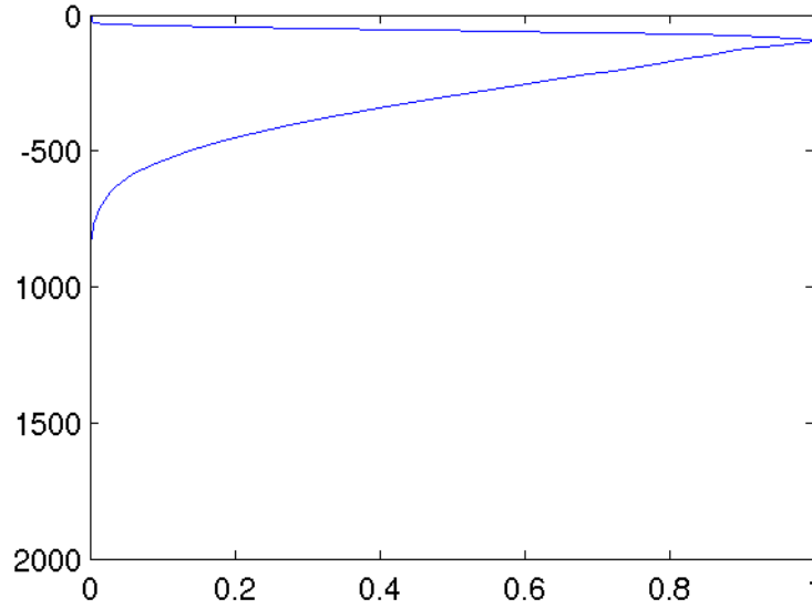
Figure F.5 : fonction g selon la profondeur à -6.7^\circ , 46.1^\circ N
