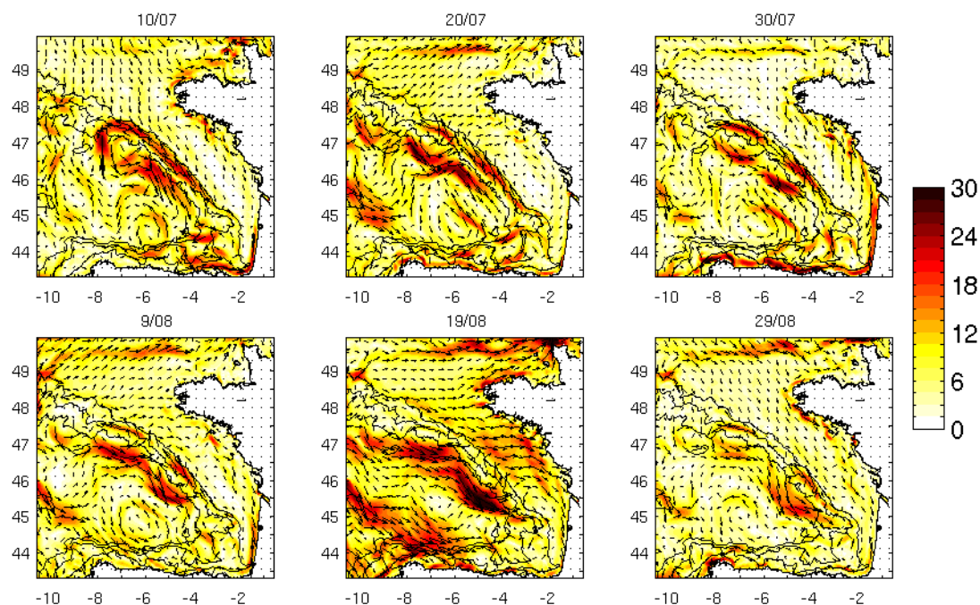
Figure D.32 : Evolution des courants de surface ( \text{cm.s}^{-1} ) au cours de la simulation. La flèche de référence sur le continent représente 10 \text{cm.s}^{-1} . Les isobathes 200, 2000 et 4000m sont indiqués.
