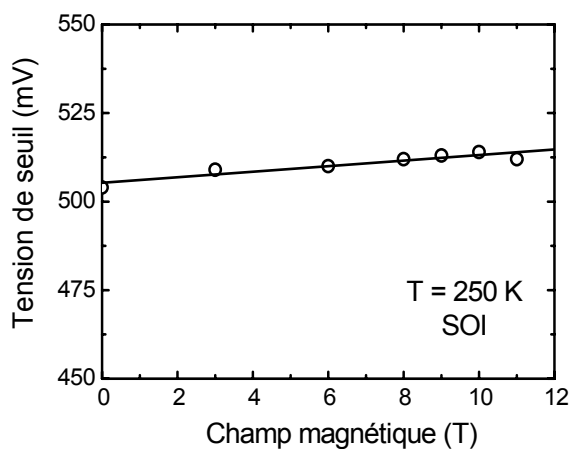
Figure IV-55 : Evolution de la tension de seuil, déterminée à I_D = cte = 10^{-7} W/L , en fonction du champ magnétique.
