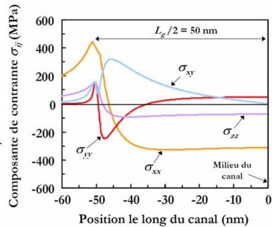
Figure II-73 : Profil spatial des composantes \sigma_{ij} du tenseur des contraintes dans le canal d'un transistor FDSOI, juste dessous la grille. La position de référence à 0 nm correspond au milieu du canal. Tirée de [GUILLA 04a, 05b]
