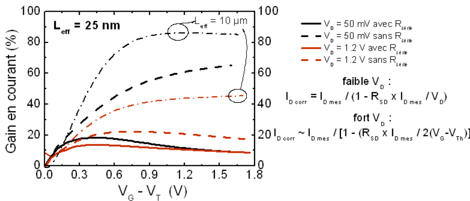
Figures V-45 : Evolution du gain en courant avec V_G - V_T pour deux longueurs de grille différentes (10 \mu m et 25nm) et pour deux conditions de polarisation sur le drain (régime linéaire et de saturation). L'effet des R_{série} est illustré sur la figure du bas sur le transistor ultracourt.
