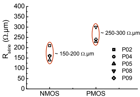
Figure VI-15 : R_{\text{série}} des N&PMOSFET
