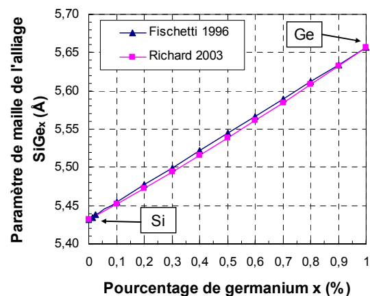
Figure II-49 : Relation entre la proportion de germanium dans l'alliage SiGe et son paramètre de maille correspondant.
