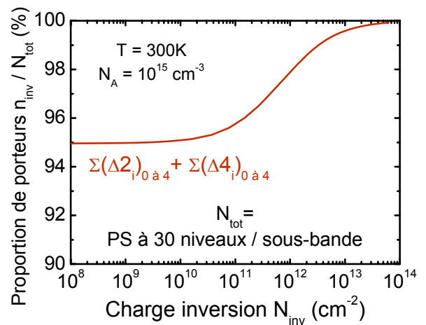
Figure V-37 : Proportion de porteurs pris en compte par une simulation intégrant 5 niveaux par vallée par rapport à une simulation à 30 niveaux par vallée.
