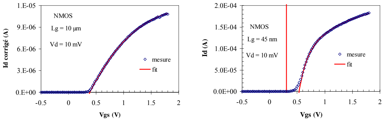
Figures IV-18 : Exemple de fit avec la méthode de la dérivée seconde de l'inverse du courant de drain pour deux longueurs de grille effectives (10 \mu\text{m} et 45 nm). Les courants ont été préalablement corrigés des fuites de grille. On peut noter qu'avec cette méthode la tension de seuil de seuil est légèrement sur-estimée.
