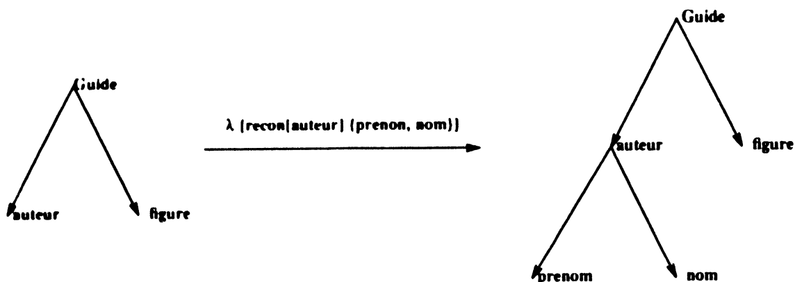
Fig. 2.14 : Opération "modification" avec reconnaissance d'une valeur.
