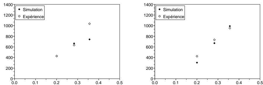
FIG. C.28 – Maximum de la force d'impact ( daN ) entre le confinement droit et les assemblages combustibles en fonction du niveau d'excitation ( g ) EDF3 à gauche et FRA3 à droite, en eau pour un confinement de 1.5\text{ mm} , comparaison expérience/simulation
