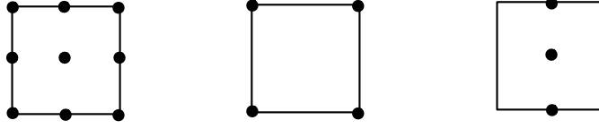
FIG. III.10 – Mailles 2D pour la discrétisation du fluide (gauche), de la pression (milieu) et de la structure (droite)
