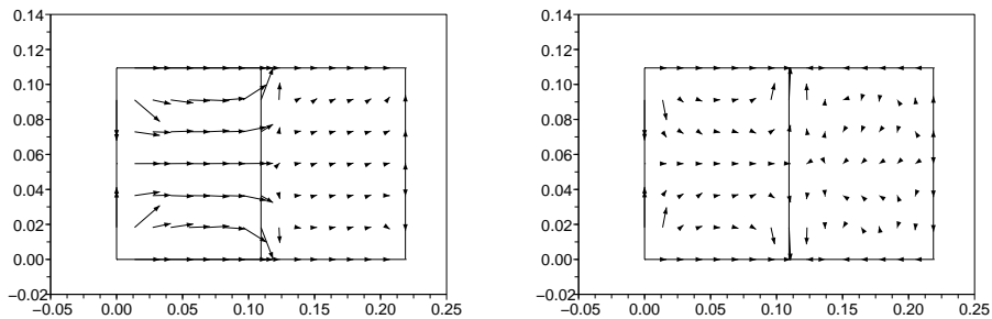
FIG. III.14 – Estimation numérique du champ de vitesse du fluide dans le plan médian, à t = 0.09 s (gauche) et t = 0.15 s (droite)
