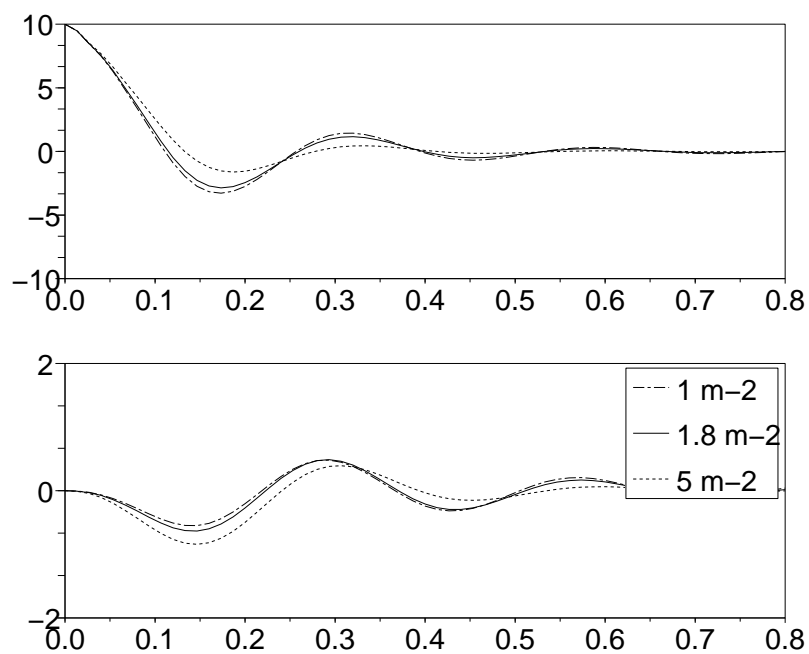
FIG. III.18 – Déplacements ( mm ) en fonction du temps ( s ) des troisièmes grilles des assemblages combustibles gauche (haut) et droite (bas) en eau sous écoulement à 2.4 \text{ m/s} pour une amplitude de lâcher de 10 \text{ mm} , pour plusieurs valeurs de C_N
