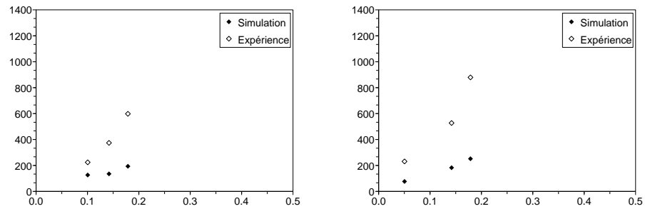
FIG. C.23 – Maximum de la force d'impact ( daN ) entre le confinement gauche et les assemblages combustibles en fonction du niveau d'excitation ( g ) EDF3 à gauche et FRA3 à droite, en air, comparaison expérience/simulation
