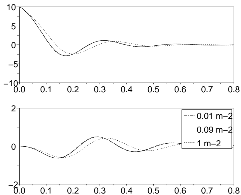
FIG. III.17 – Déplacements ( mm ) en fonction du temps ( s ) des troisièmes grilles des assemblages combustibles gauche (haut) et droite (bas) en eau sous écoulement à 2.4 \text{ m/s} pour une amplitude de lâcher de 10 \text{ mm} , pour plusieurs valeurs de C_T
