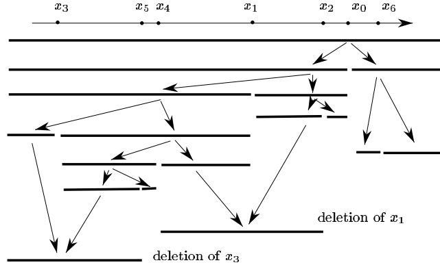
FIG. I.4 – l'histoire des suppressions
