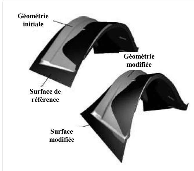
FIG. 1.12 – La modification de la géométrie avec le contrôle de la surface.
