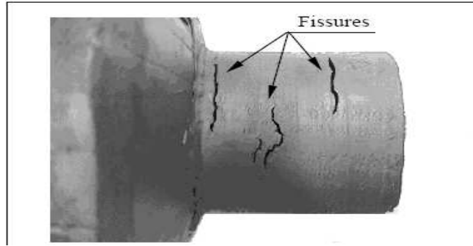
FIG. 1.33 – Fissuration externe durant l’extrusion.
