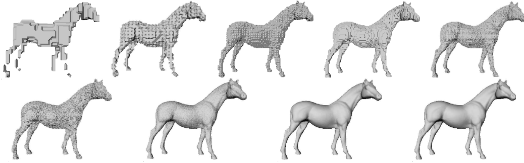
Figure I.5: Décompression d'un modèle de cheval échantillonné sur une grille régulière de taille 257^3 . Les premières images correspondent aux raffinements de la multitriangulation, suivi des raffinements de la géométrie.
