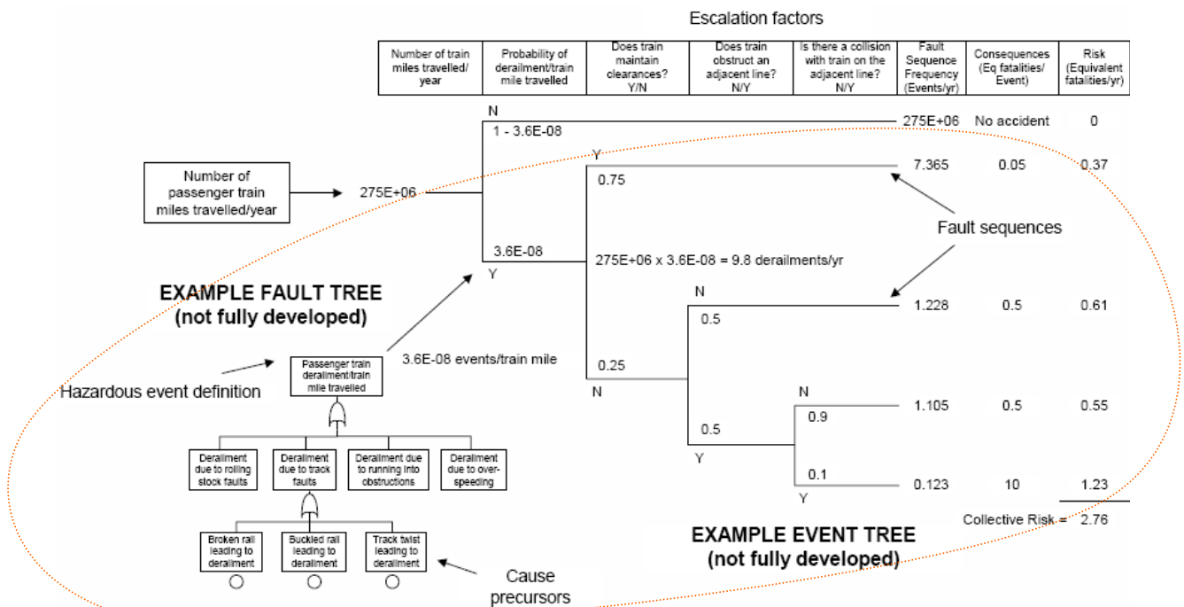
FIG. 4: Ebauche d'un nœud papillon – déraillement d'un train de transport de passagers [Rausand, 04]
