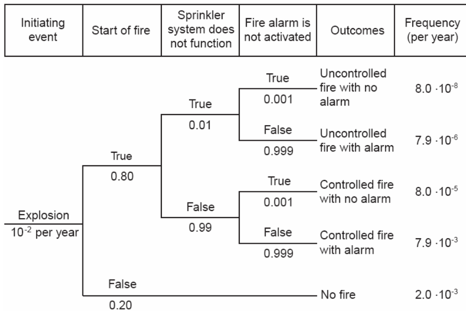
FIG. 2: Arbre d'événement d'un système anti-incendie [Rausand, 04]
