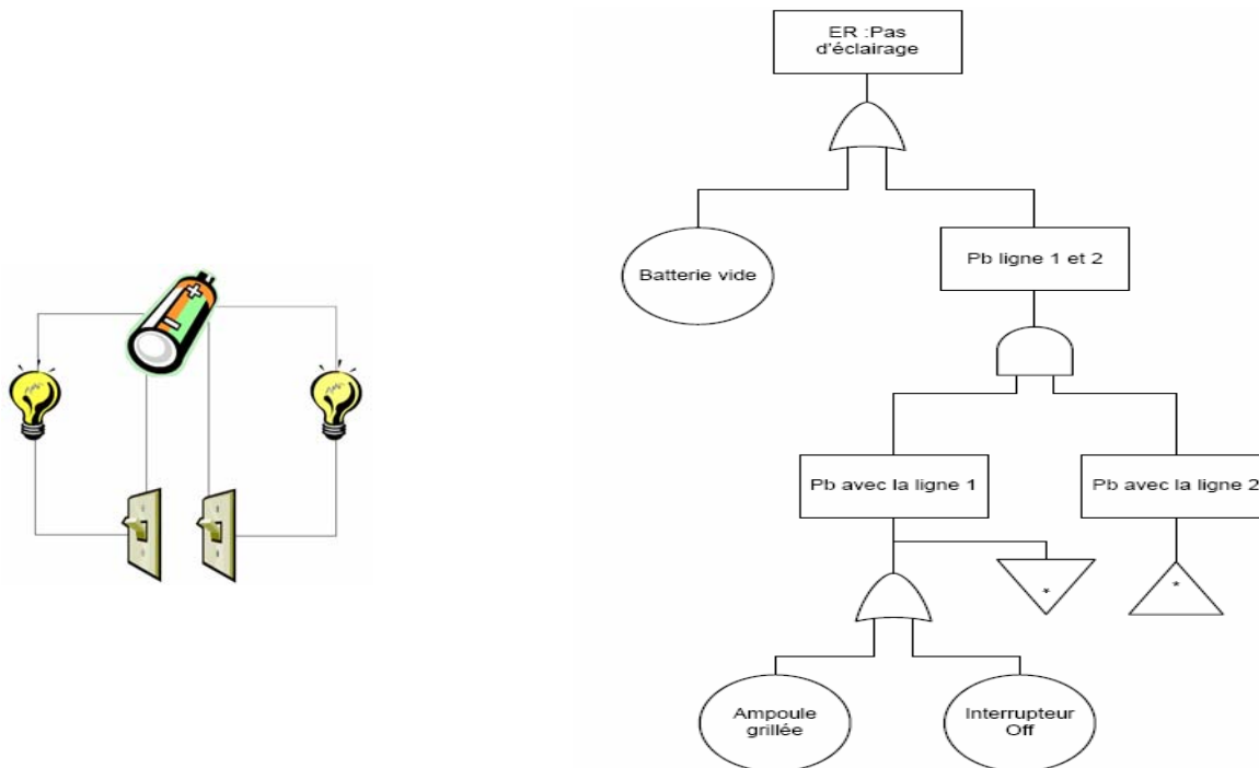
FIG. 1 : Exemple d'un arbre de défaillance
