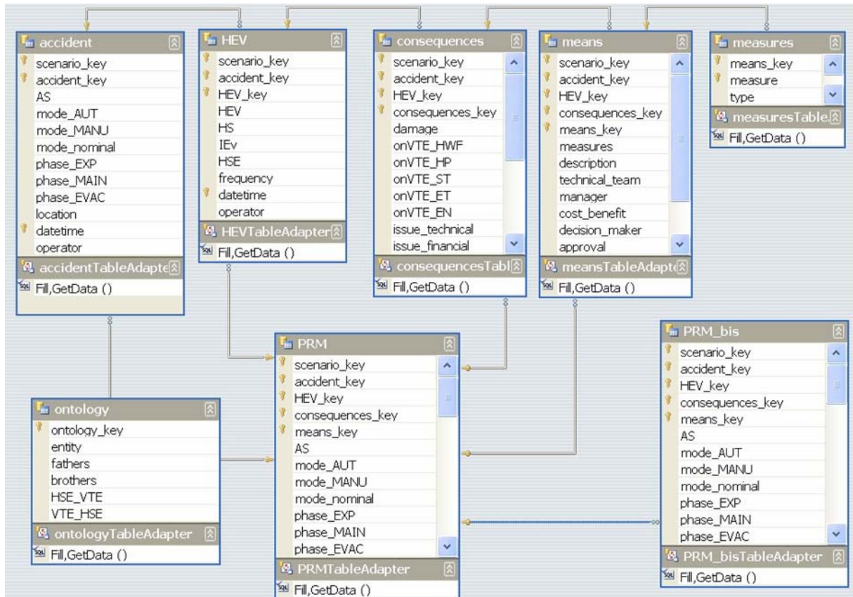
FIG. 2: Modèle de données de la base de données SIAD
