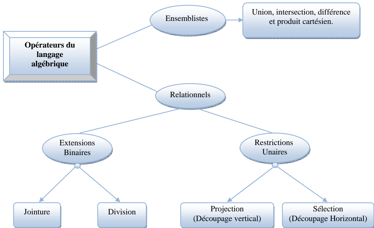
FIG. 4: Opérateurs du langage algébrique
