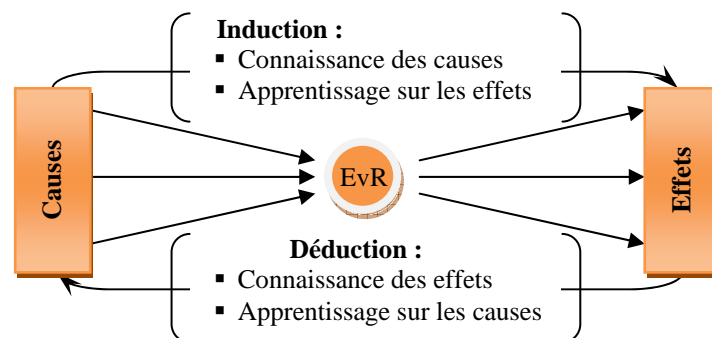
FIG. 1: Raisonnement causal : Induction et Déduction
