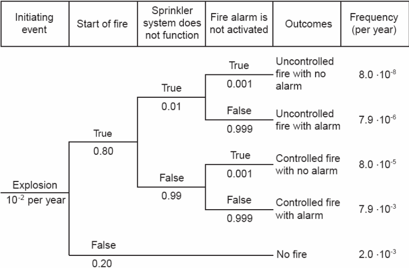
FIG. 2: Arbre d'évènement d'un système anti-incendie (Rausand & Hoyland, 2004)
