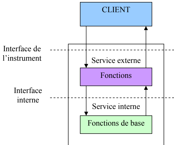
Figure 1.8 : Modèle client/serveur
