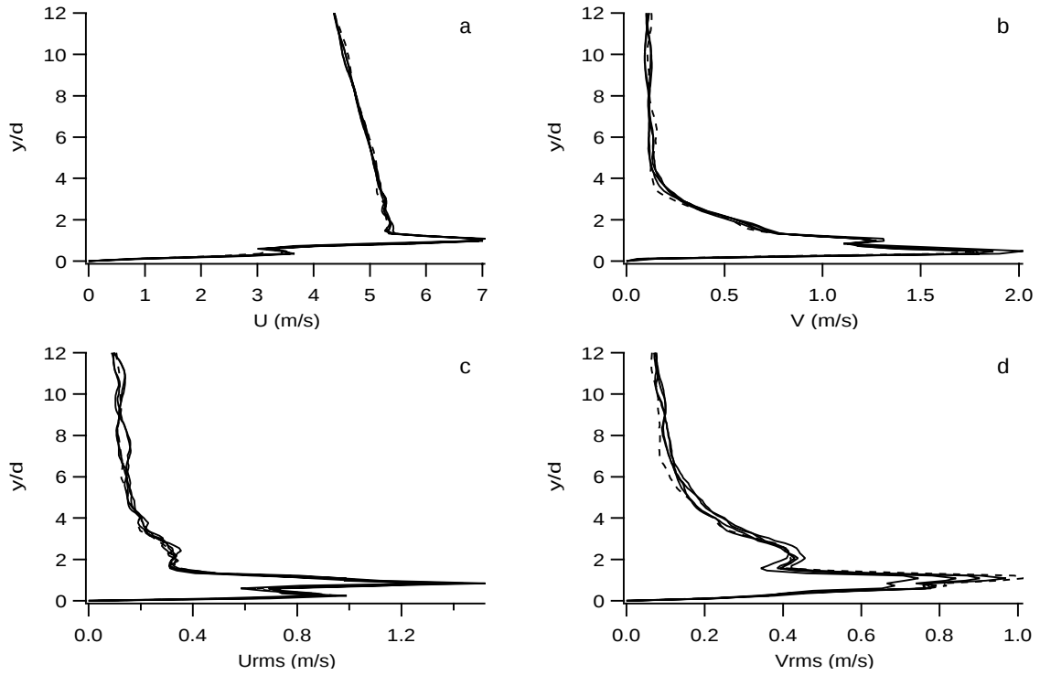
FIG. 4.7 - Comparaisons des calculs incluant dans le domaine périodique 1 trou (cas 4, ---) ou 4 trous (cas 7, —). Profils de vitesses 2.92 d en aval du centre de la perforation, côté injection. a. Vitesse longitudinale moyenne U . b. Vitesse verticale moyenne V . c. Vitesse longitudinale fluctuante U_{rms} . d. Vitesse verticale fluctuante V_{rms} .
