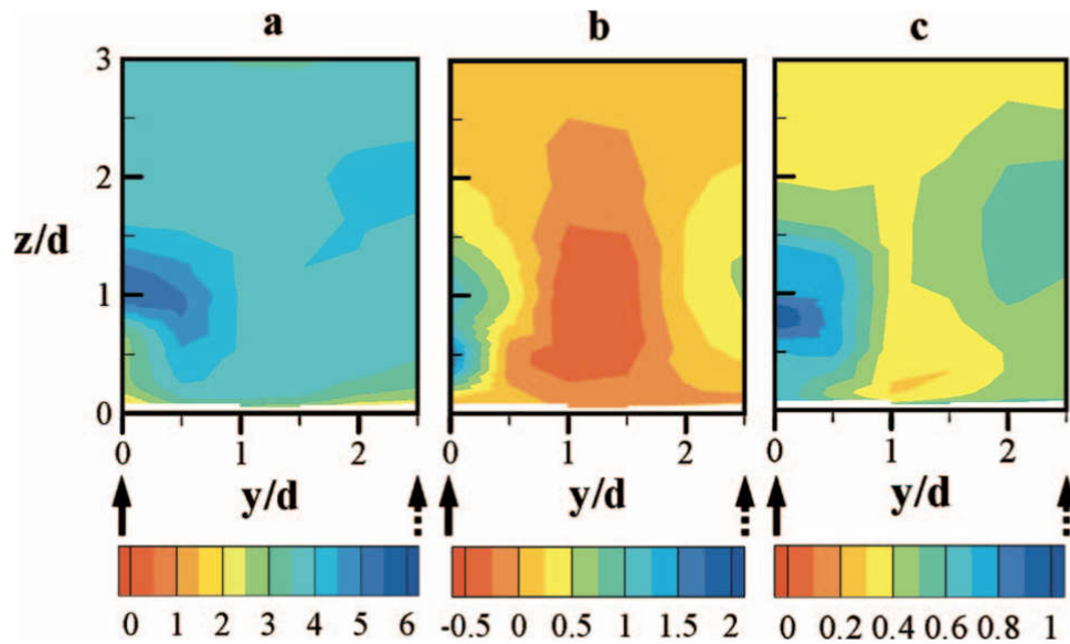
FIG. 2.14 - Plan perpendiculaire à l'écoulement, 3d en aval du centre d'un jet de la rangée 15. a) Vitesse longitudinale moyenne. b) Vitesse verticale moyenne. c) Intensité de turbulence. Grandeurs adimensionnées par la vitesse de l'écoulement principal. D'après Scrittore et al. (2007) .
