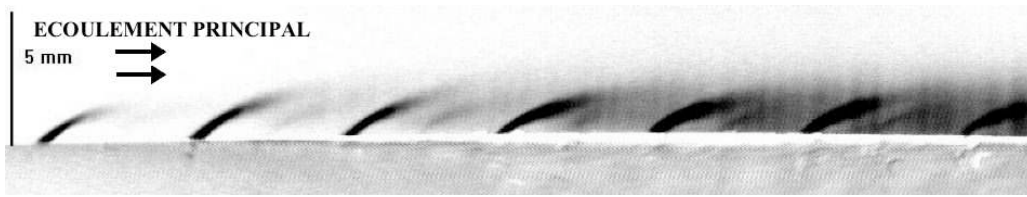
FIG. 2.4 - Image d'un film de refroidissement. Visualisation par fumée issue de la thèse de Rouvreau (2001) .
