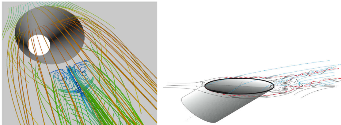
FIG. 2.19 - Mesures au niveau de la troisi me rang e d'une plaque multi-perfor e : structure de l' coulement. Gauche : tubes de courant color s par le module de vitesse. Droite : sch ma d'interpr tation. D'apr s Gustafsson (2001) .
