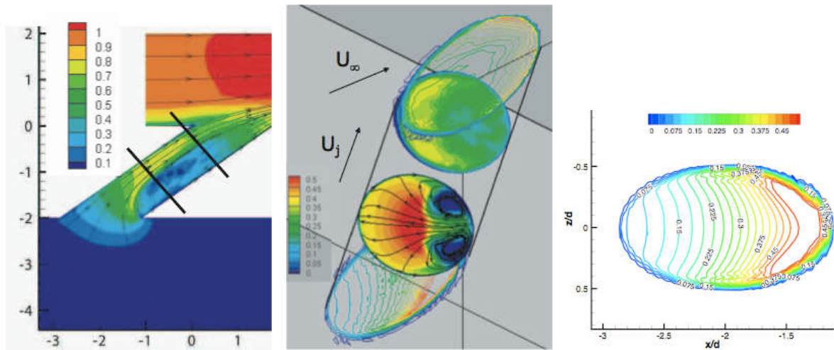
FIG. 2.22 - Vue de l'écoulement moyen dans la perforation, d'après Peet (2006) . Gauche : champ de module vitesse et lignes de courant. Centre : champs de vitesse verticale et lignes de courant. Droite : plan d'entrée du trou, champ de vitesse verticale.
