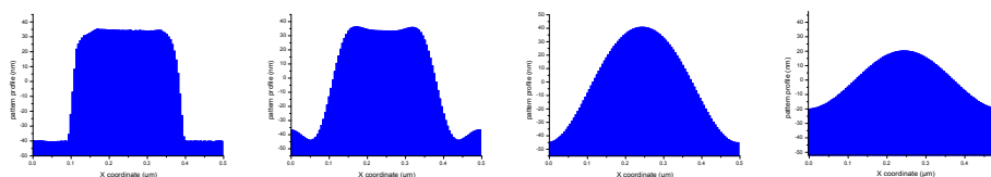
Fig. 8.3: Déformation d'un créneau de résine PS130K durant son élévation de température. Mesures réalisées par AFM.
