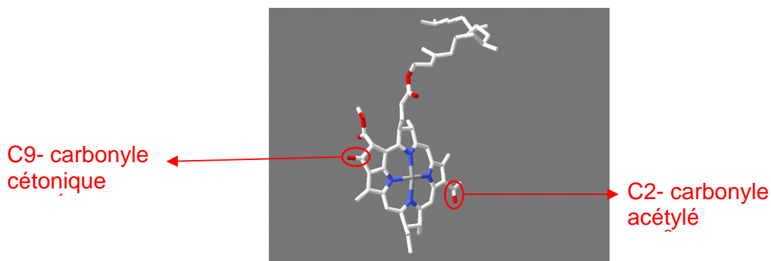
Figure 2.12 : Structure moléculaire de la bactériochlorophylle a. Les groupements carbonyles cétonique (C9, nomenclature de Fischer ou C13 1 , nomenclature de IUPAC-IUB depuis 1988) et acétylé (C2 ou C3 2 ) sont entourés en rouge.
