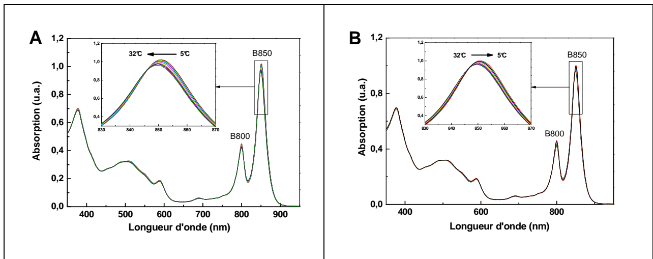
Figure 2-7 : Evolution du spectre d'absorption de la protéine LH2 de Rb. sphaeroides DD13-wt en fonction de la température. A : Phase de chauffe : de 5 à 32 °C en 180 min ; B : Phase de refroidissement : de 32 à 5 °C en 360 min.
