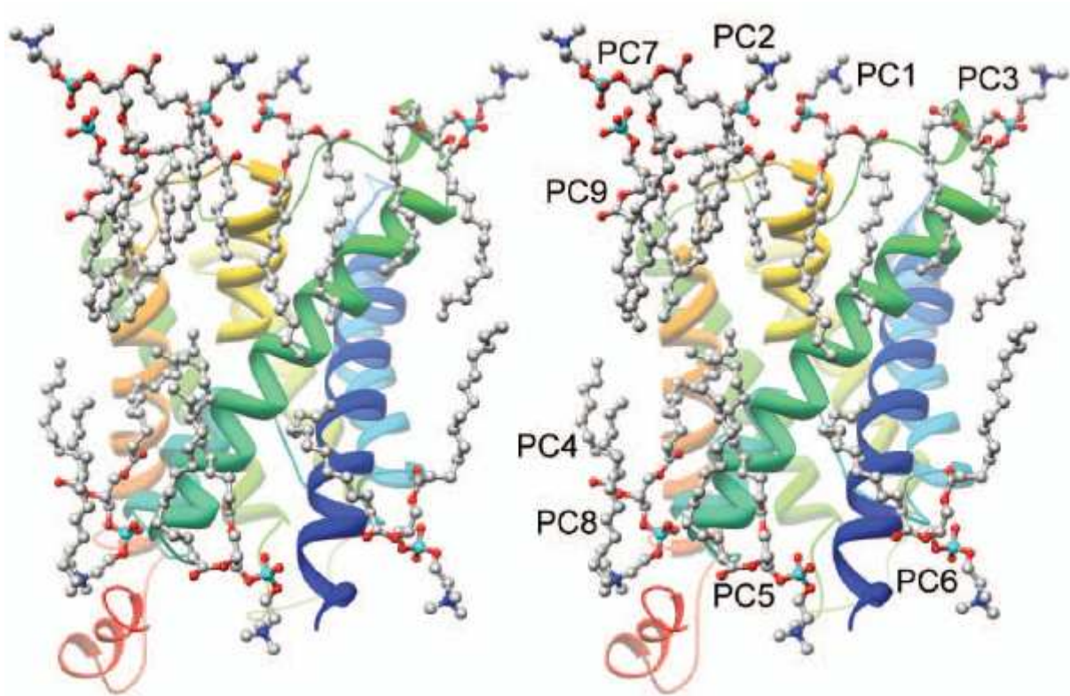
Figure 1-3 : Lipides en interaction avec un monomère d'aquaporine AQP0 dans un cristal 2D (vue en stéréo). PC1 à PC7 sont les lipides formant un anneau en contact direct avec la protéine, à la différence de PC8 et PC9. Les hélices H1 à H6 du monomère AQP0 sont en couleur (Gonen et al., 2005)
