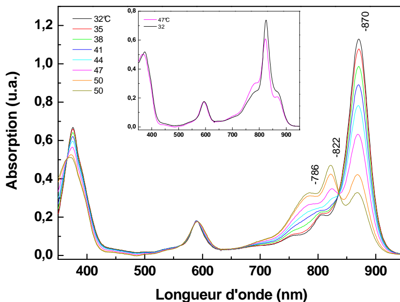
Figure 3-4 : Effet de la température sur le spectre d'absorption du complexe RC-LH1 de G9+ purifié en détergent DDM ( 32 < T < 50^{\circ}\text{C} et 650 < \lambda < 950\text{ nm} )
