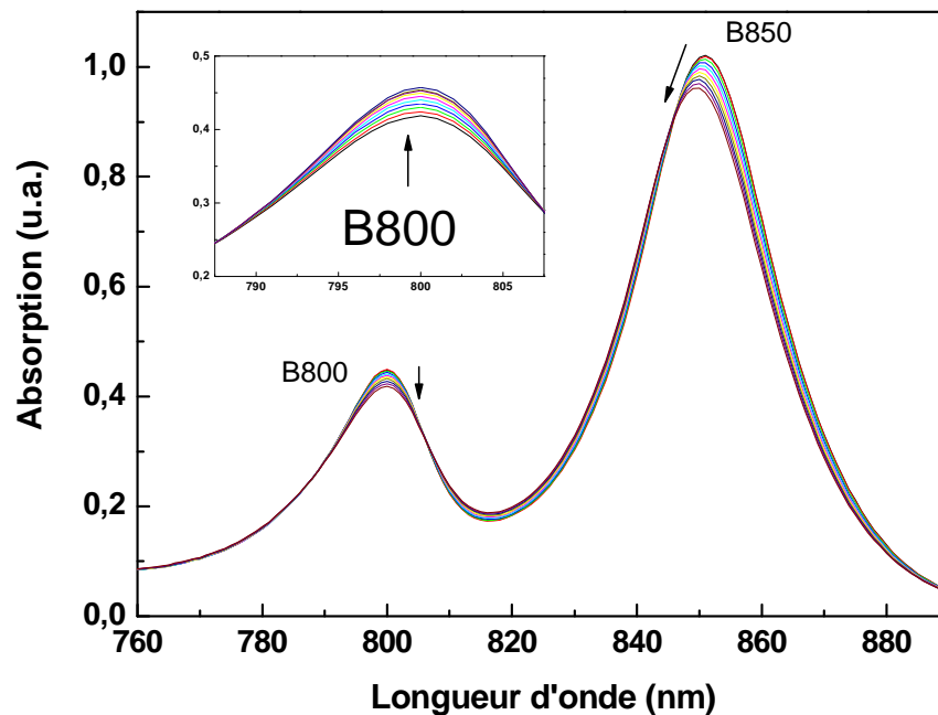
Figure 2-9 : Evolution du spectre d'absorption de la protéine LH2 dans le proche infrarouge en fonction de la température (de 5 à 32 °C). Insertion : évolution du maximum d'absorption du B800 en fonction de la température (de 32 à 5 °C). Les flèches noires représentent une augmentation ou une diminution des maximums d'absorption.
