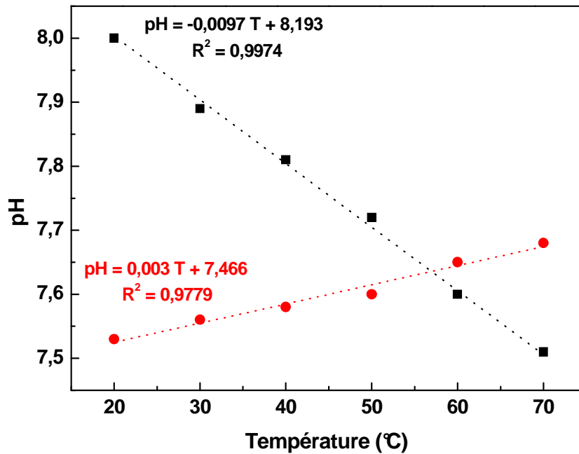
Figure 5-1 : Evolution du pH des tampons Tris-HCl 20 mM (-■-) et phosphate de potassium 50 mM (-●-) en fonction de la température. La régression linéaire indique que le pH du tampon phosphate change d'environ 0,003 unité de pH/°C, valeur négligeable pour les expériences.
