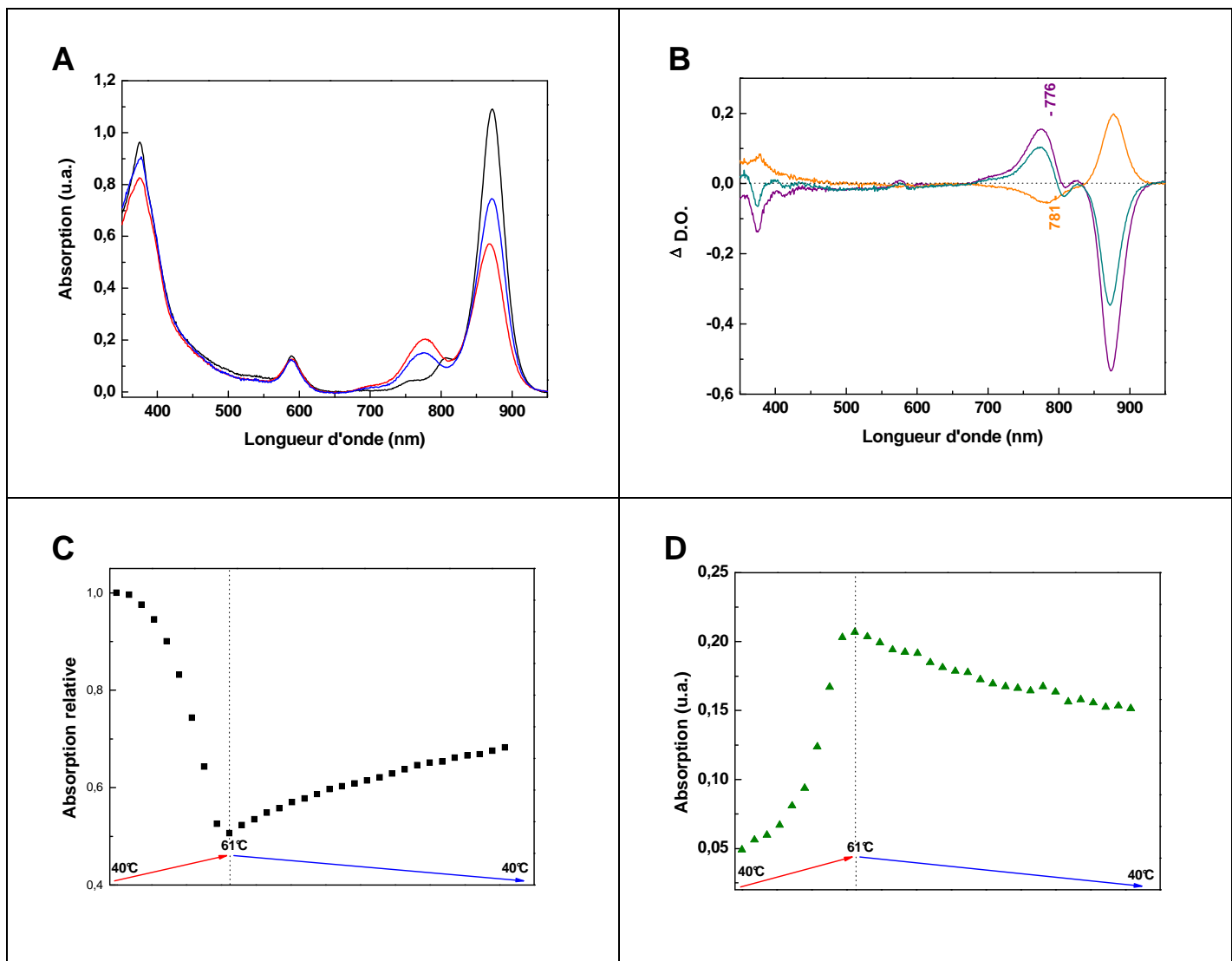
Figure 3-13 : Dissociation-réassociation de la protéine LH1 chez Rsp. rubrum G9 entre 40 et 61 °C à pH 8,5. A) Spectres d'absorption à 40 °C (—), température initiale ; à 61 °C (---), fin de phase de chauffe ; et à 40 °C (—), fin de phase de refroidissement. B) Soustractions des spectres d'absorption : (—) : 40 °C initial - 67 °C ; (—) : 40 °C fin - 67 °C ; (—) : 40 °C initial - 40 °C fin. C) Evolution des maximums d'absorption de la transition Qy des Bchl a (—■—) D) Evolution de l'absorption à 777 nm (—▼—)
