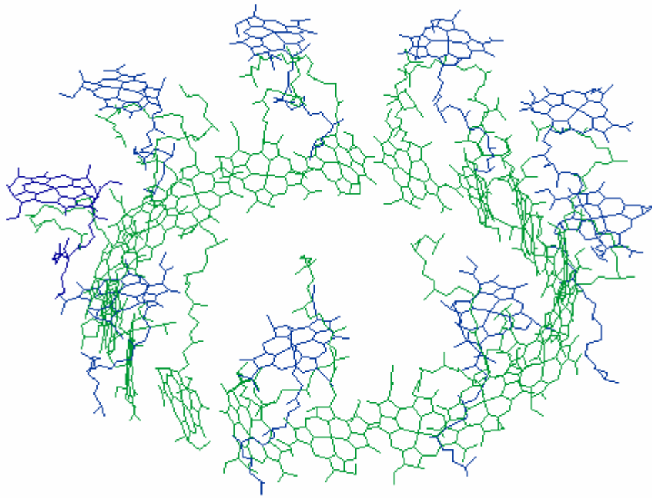
Figure 2-6 : Arrangements structuraux des 9 Bchls-B800 (en bleu) et des 18 Bchls-B850 (en vert) de la protéine LH2 de Rps. acidophila (d'après la structure 3D à 2,45Å de résolution, PDB : 2fkw (Cherezov et al., 2006))
